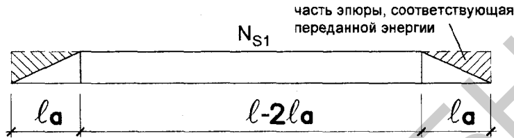
Рис. 2. К определению части потерянной энергии преднапряжения
