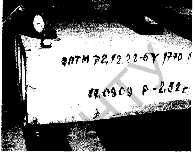
Рис. 8. Разрушение эталонной плиты 2ПТМ72.12.22-9Y1770S7-1 по наклонному сечению при пролете среза c = 2,8d
