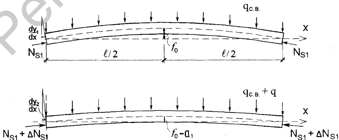
Рис. 7. Два состояния нагруженной предварительно напряженной плиты
