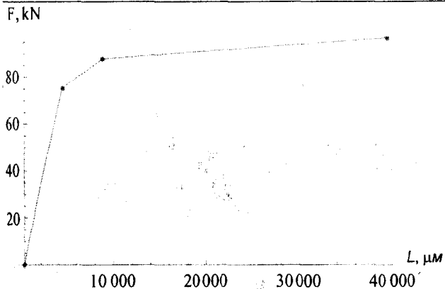
Рис. 6. Зависимость «сила – удлинение» для арматурной пряди Ø 9,3 мм Y1770S7
