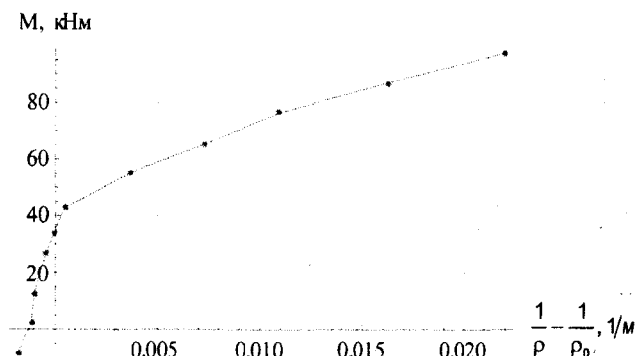
Рис. 5. Диаграмма «момент-кривизна» для плиты 2ПТМ72.12.22-6У1770
