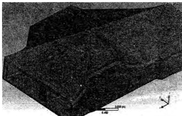
Рис. 4. Конечно-элементная модель опоры
