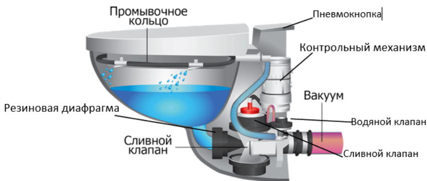
Рисунок 1 – Схема вакуумного унитаза
