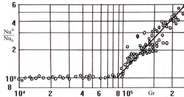
Рис. 3. Зависимость \frac{Nu^3}{Nu_0} = f(Gr)
