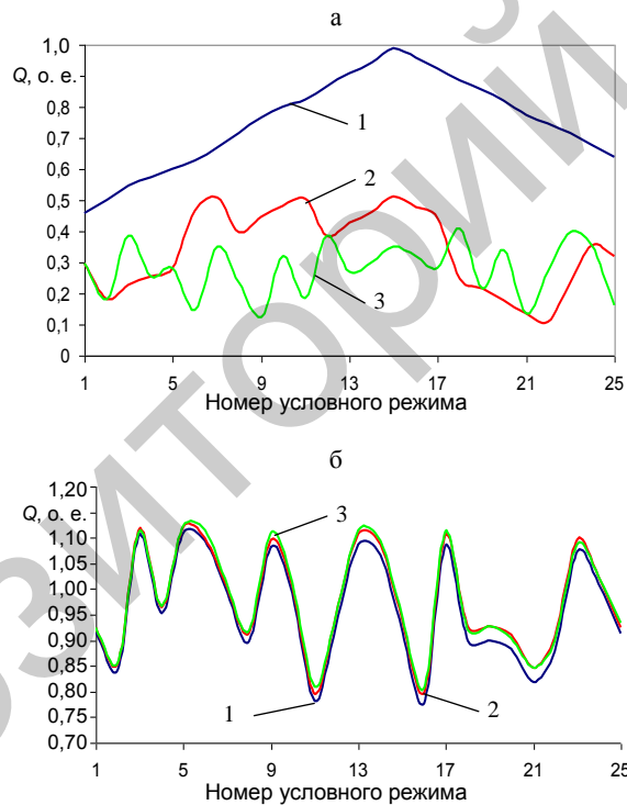
Рис. 7. Диаграмма работы традиционного и fuzzy-управления: а – изменение реактивной нагрузки; б – изменение напряжения; 1 – исходный режим; 2 – при нечетком управлении; 3 – при традиционном управлении
