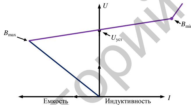
Рис. 2. Рабочая характеристика СТК
