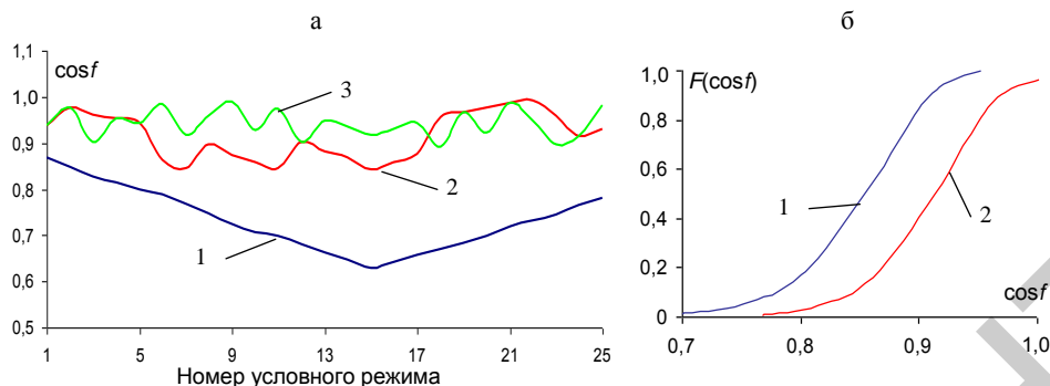
Рис. 8. Закономерность изменения коэффициента мощности: а – кривые изменения: 1 – исходный режим; 2 – при нечетком управлении; 3 – при традиционном управлении; б – функции распределения: 1 – исходный режим; 2 – при нечетком управлении
