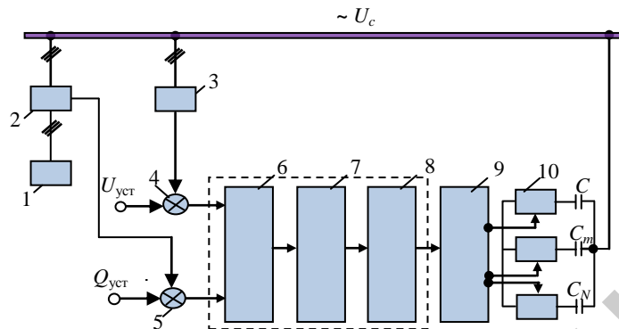
Рис. 3. Структурная схема системы fuzzy-управления реактивной мощностью
