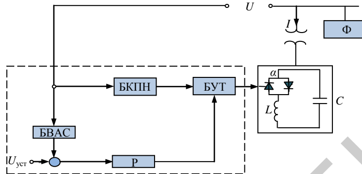
Рис. 1. Схема СТК: БКПН – блок контроля перехода тока через нуль; БУТ – блок управления тиристорами; БВАС – блок выделения амплитуды сигнала; Φ – фильтр; P – регулятор
