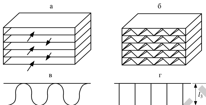
Рис. 2. Схема потоков воздуха и поверхностей теплообмена теплоутилизатора с пластинами: а – гладкими; б – треугольными; в – U-образными; г – П-образными
