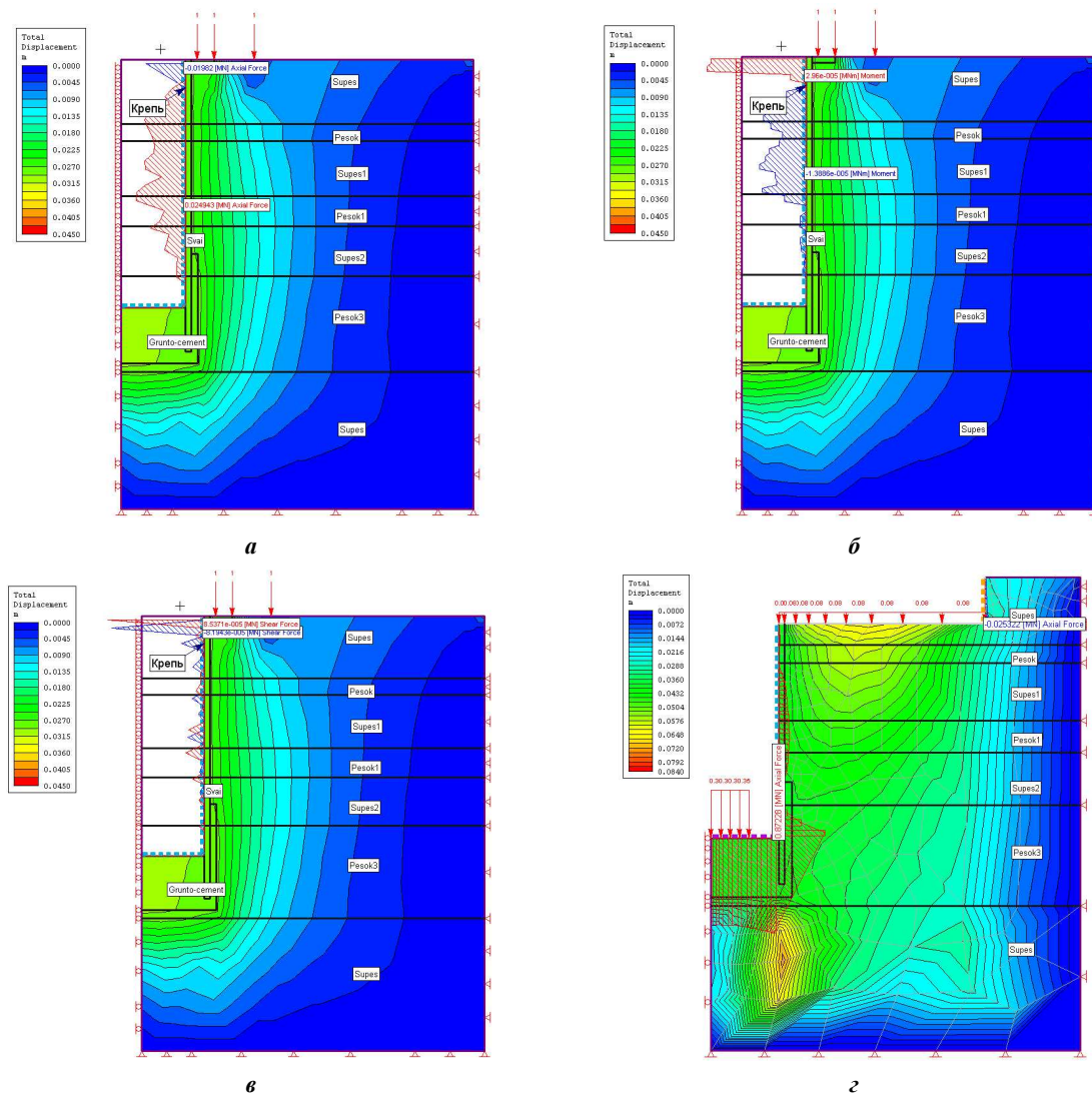
а, з – эпюры осевых усилий сжатия; б, д – эпюры изгибающих моментов; в, е – эпюры усилий сдвига Рисунок 2. – Результаты расчетов общих смещений при проходке шахты (а, б, в) и в период эксплуатации (з, д, е) – см. также с. 98
