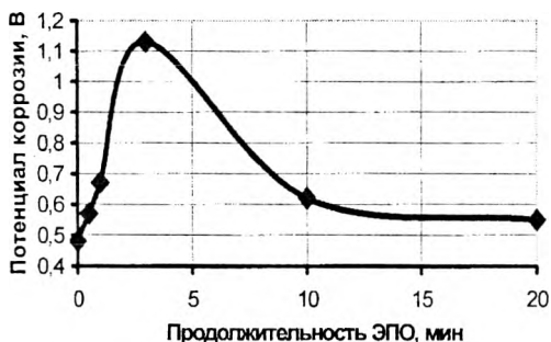
Рисунок 4 - Влияние ЭПО на изменение коррозионной стойкости поверхностного слоя.
