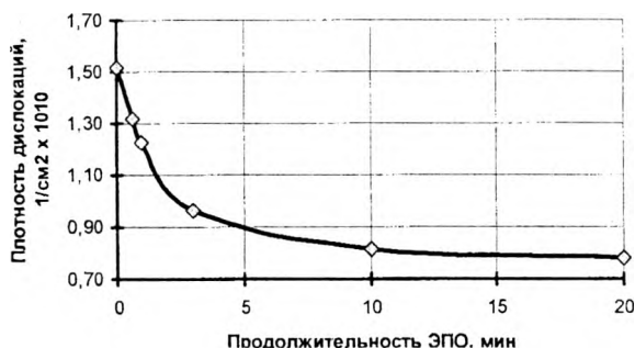
Рисунок 3 - Изменение плотности дислокаций в результате ЭПО
