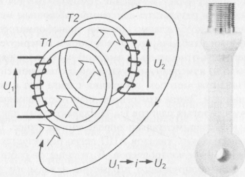
Рис. 1. Трансформаторный датчик измерения проводимости раствора
