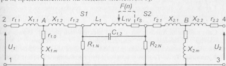
Рис. 2. Эквивалентная схема измерительной ячейки
