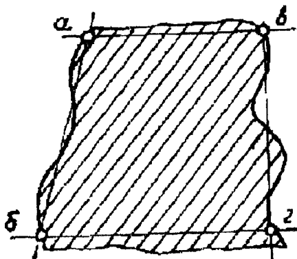
Рис. 6.4. Расчет площади фигуры методом трапеций
