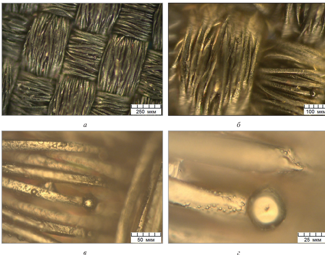
Рис.2. Морфология поверхности ткани с покрытием при различных увеличениях; светлопольное освещение
