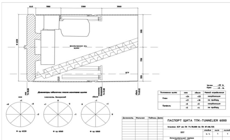
Рис. 2. Паспорт щита ТПК
