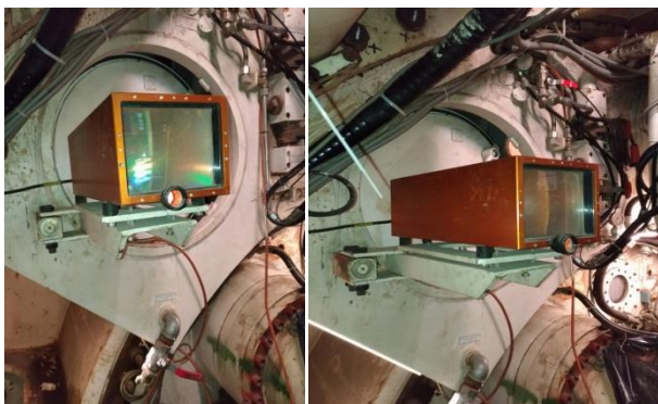
Рис. 3. Комбинированная мишень и место установки.
