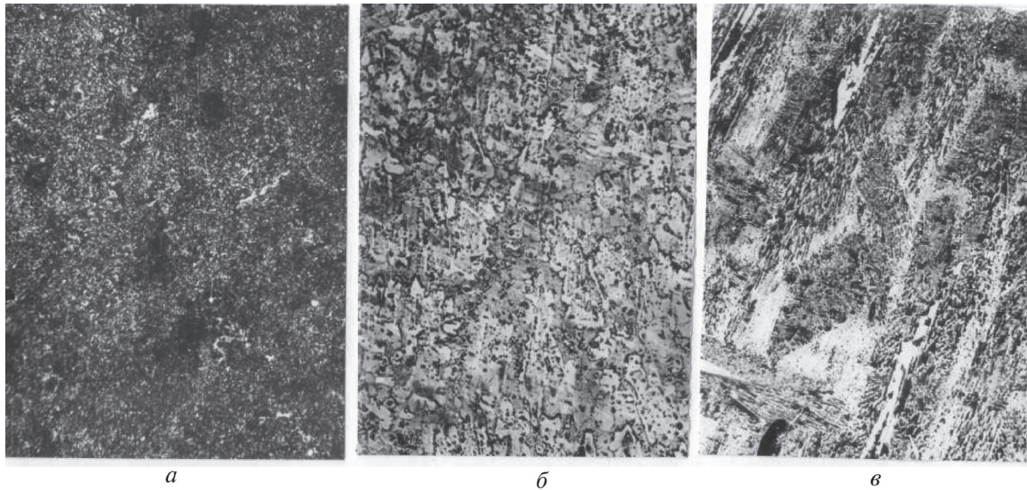
Рис 2. Влияние вводимого РЗМ в качестве модификатора на изменение структуры железобористого сплава: а – иттрий; б – иттербий; в – церий. \times 500
