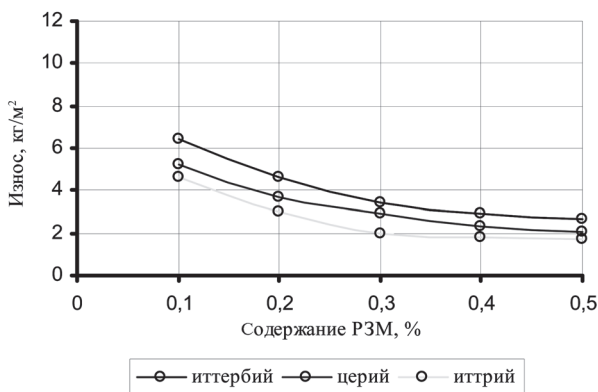
Рис. 3. Износостойкость в системе металл–металл
