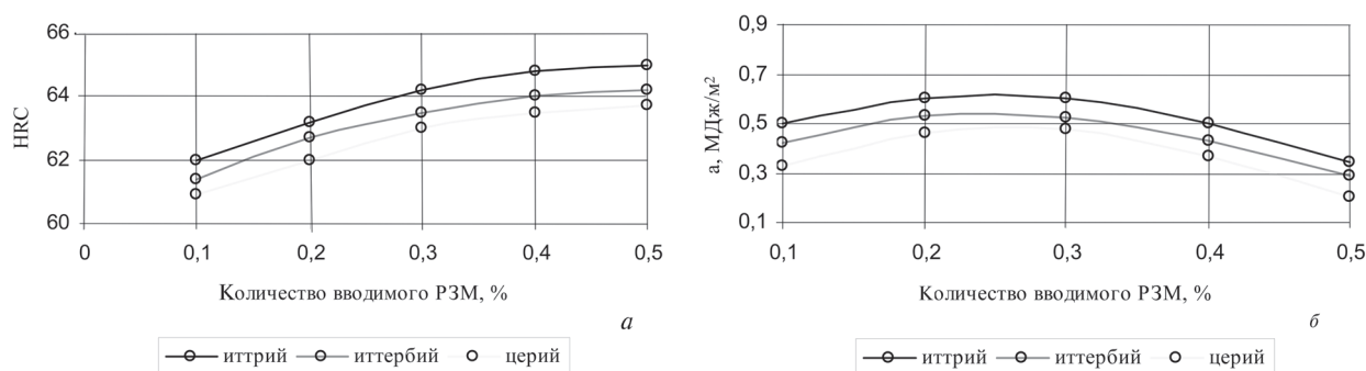
Рис. 1. Влияние количества РЗМ на твердость (а), ударную вязкость (б)
