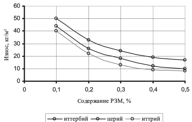
Рис. 4. Износостойкость в системе металл–абразив
