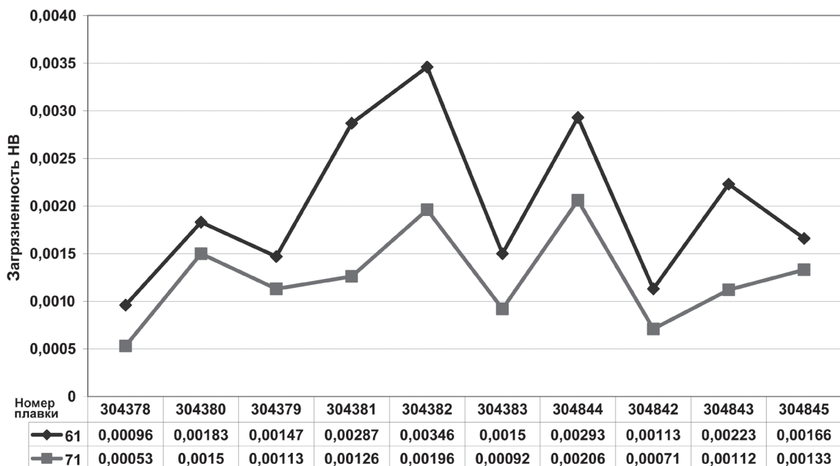
Рис. 1. Диаграмма результатов количественной оценки загрязненности неметаллическими включениями исследуемых плавков
