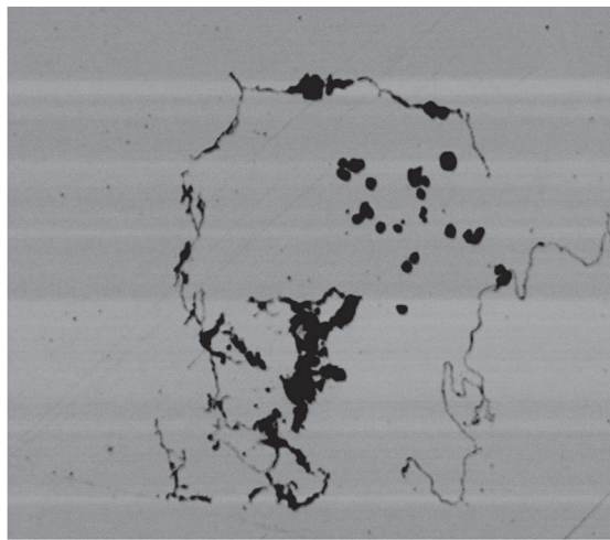
Рис. 6. Оксид алюминия (корунд Al_2O_3 ) в стали 80 ( a ) и 42Cr4Mo2 ( б )
