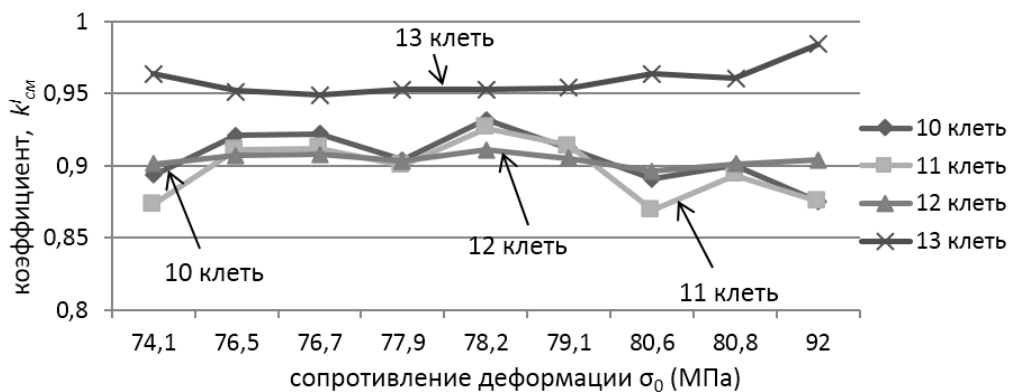
Рис. 2. Изменение коэффициентов влияния СМ k'_{см} в зависимости от сопротивления деформации \sigma_0 для клеток №10-13 НШСПИ 2000
