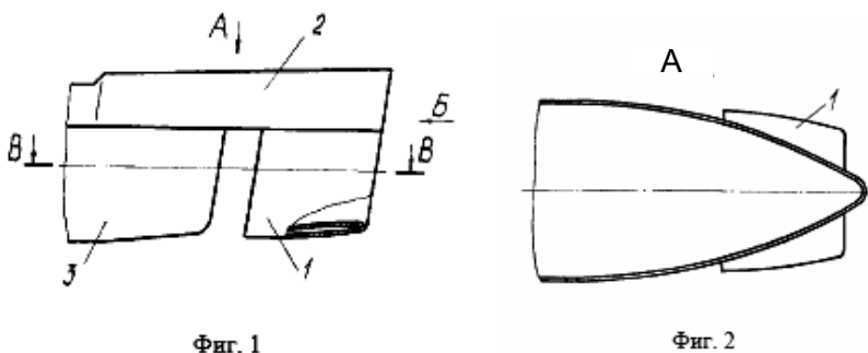
Рис. 4.1. Фигуры № 1 и 2 по патенту № 3524
