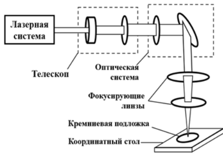
Рисунок 1 – Схема лазерной обработки отверстий в подложке
