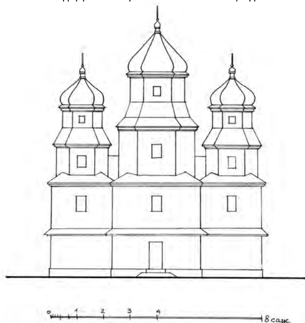
Рис. 2. Фасад церкви св. Михаила в м. Чемерисы Волоские Могилевского у., 1766 г.
