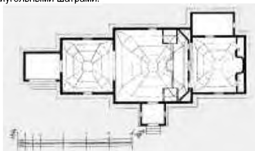
Рис. 3. План церкви св. Михаила в м. Чемерисы Волоские Могилевского у., 1766 г.
