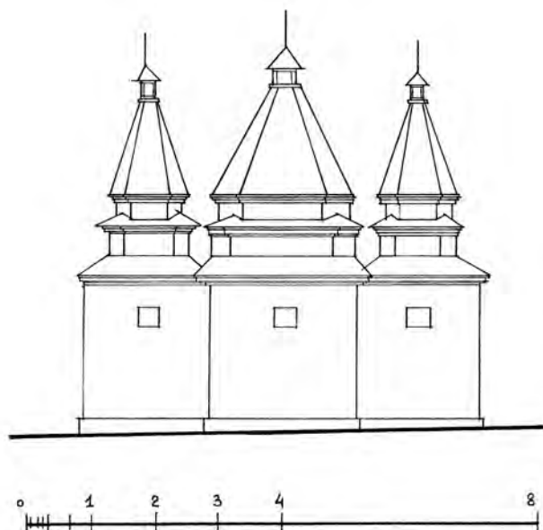
Рис. 1. Фасад церкви в с. Громовка Могилевского уезда. XVIII в.
