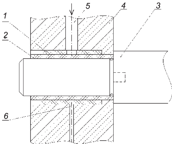
Рис. 2. Трибологическая пара для определения коэффициента трения и износостойкости: 1 – наружная втулка; 2 – внутренняя втулка; 3 – вращающийся вал; 4 – зажимное устройство; 5 – канал для подвода масла; 6 – отверстия для датчика температуры
