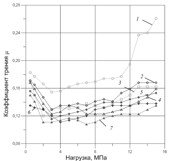
Рис. 5. Влияние нагрузки на коэффициент трения (при скорости трения скольжения 1 м/с без смазки) для различного количества добавок MoS 2 : 1 – эталон; 2 – добавка 1,8% MoS 2 ; 3 – 2,0; 4 – 2,2; 5 – 2,5; 6 – 2,8; 7 – 3,0% MoS 2
