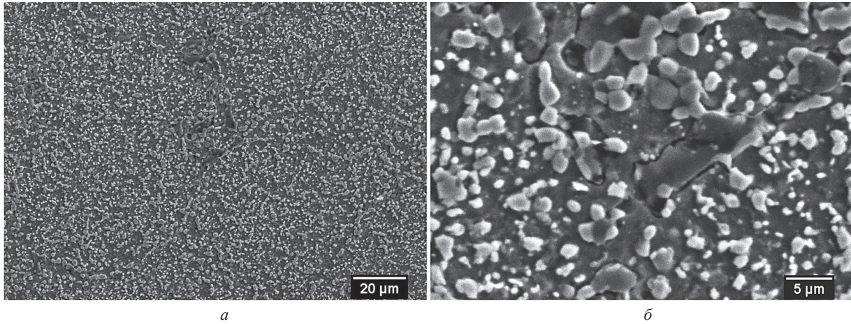
Рис. 3. Структура порошковой быстрорежущей стали с добавкой 1,8% MoS 2 после отжига: а – общий вид; б – фрагмент структуры
