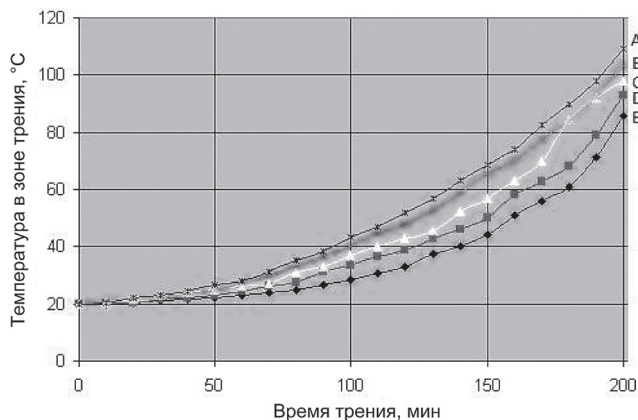
Рис. 6. Влияние времени испытаний на температуру в зоне трения (при скорости трения скольжения 1 м/с без смазки) для различного количества добавок MoS 2 : A – эталон; B – добавка 1,8% MoS 2 ; C – 2,0; D – 2,5; E – 3,0% MoS 2
