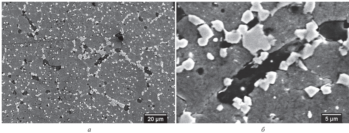
Рис. 4. Структура порошковой быстрорежущей стали с добавкой 3% MoS 2 после полной термической обработки: а – общий вид; б – фрагмент структуры
