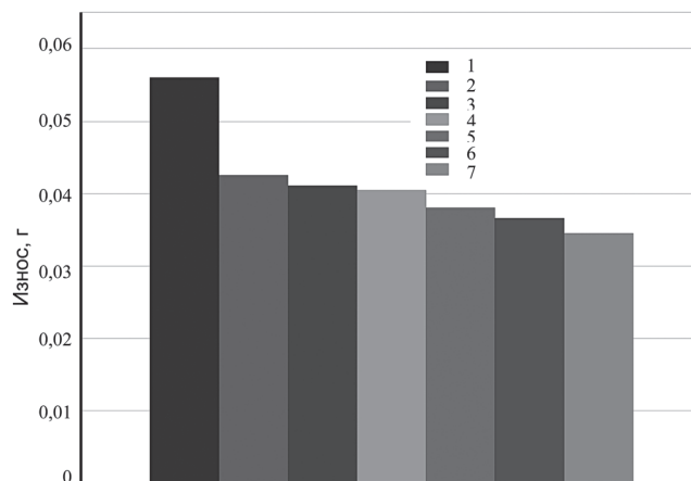
Рис. 7. Влияние количества добавок MoS 2 (при нагрузке 100 кПа и скорости трения скольжения 1 м/с без смазки) на износостойкость: 1 – эталон; 2 – стали с добавкой 1,8% MoS 2 ; 3 – 2,0; 4 – 2,2; 5 – 2,5; 6 – 2,8; 7 – 3,0% MoS 2
