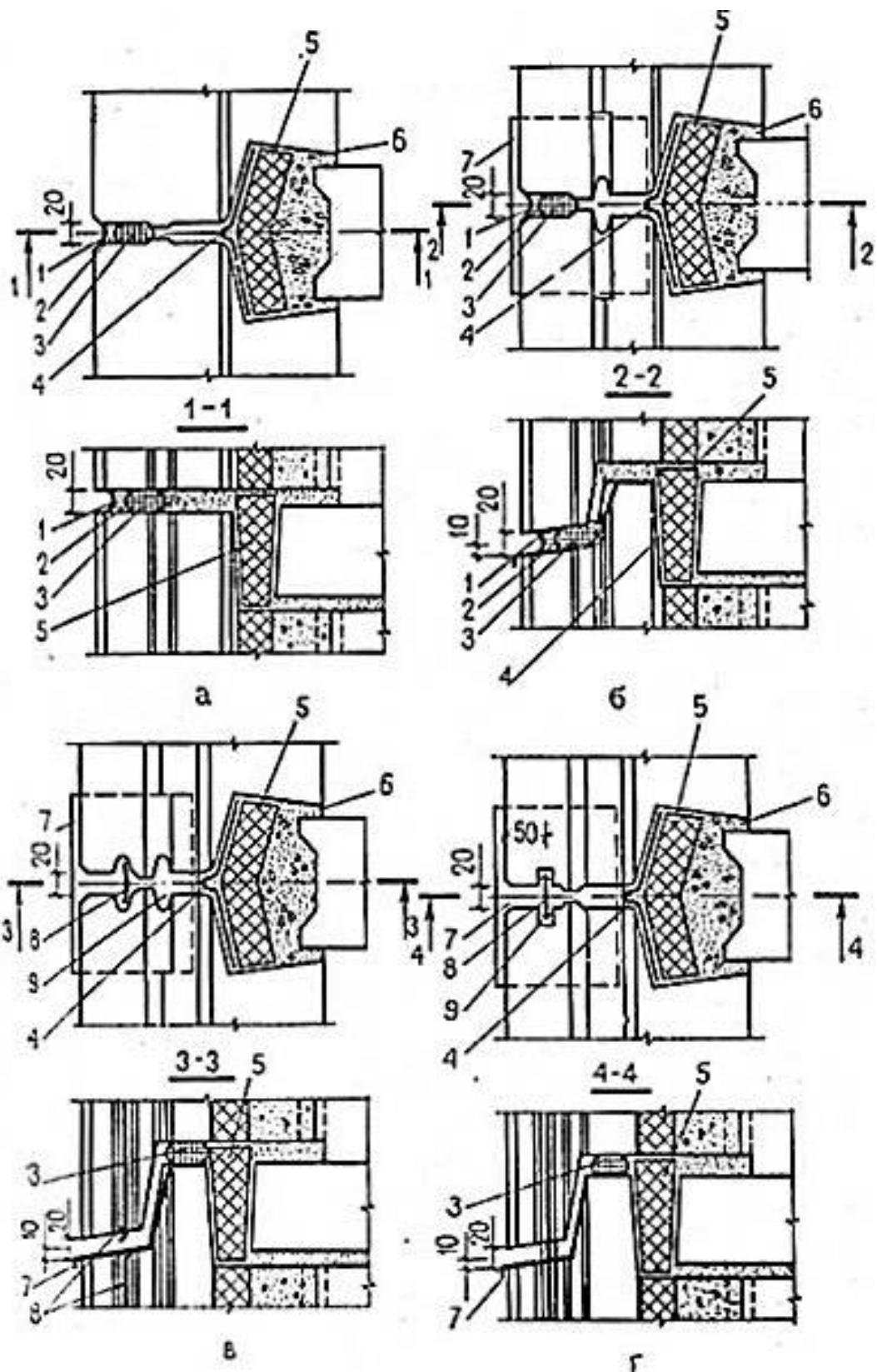
Рис. 2.19. Варианты защиты стыков панельных стен от водо-и воздухопроницания: a – закрытый; б – дренированный; в , г – варианты открытого стыка; 1 – защитное покрытие; 2 – герметизирующая мастика; 3 – упругая прокладка; 4 – наклеенная лента из гидроизоляционного материала; 5 – термовкладыш; 6 – бетон замоноличивания; 7 – водоотводящий фартук; 8 – водоотбойный экран; 9 – декомпрессионная полость
