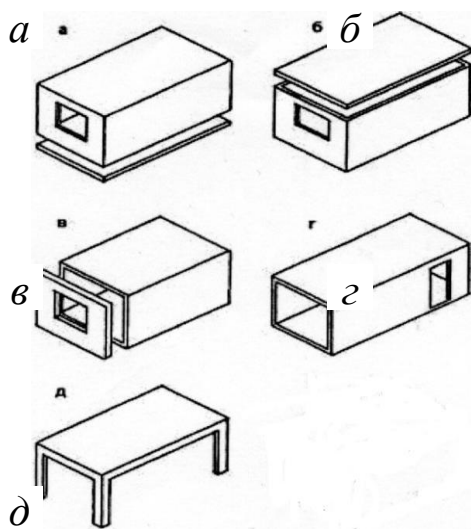
Рис. 4.7. Конструктивно-технологические типы блоков: a – монолитный блок типа «колпак»; б – монолитный блок типа «стакан»; в – лежащий стакан; г – труба; д – столик
