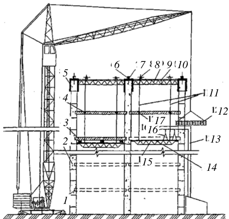
Рис. 5.3. Бетонирование междуэтажных перекрытий методом «сверху вниз»: 1 – гнезда; 2 – стена; 3 – пневматическое отрывное устройство; 4 – монолитное перекрытие; 5–домкратная рама; 6 – домкратный стержень; 7 – гидродомкрат; 8 – тормозные устройства; 9 – опалубочный щит; 10 – рабочий настил; 11 – гибкие тяги; 12 – армокаркас; 13 – бетоновод; 14 – опалубка перекрытия; 15 – несущая ферма опалубки перекрытия; 16 – стойка; 17 – гильза [31, с. 323]
