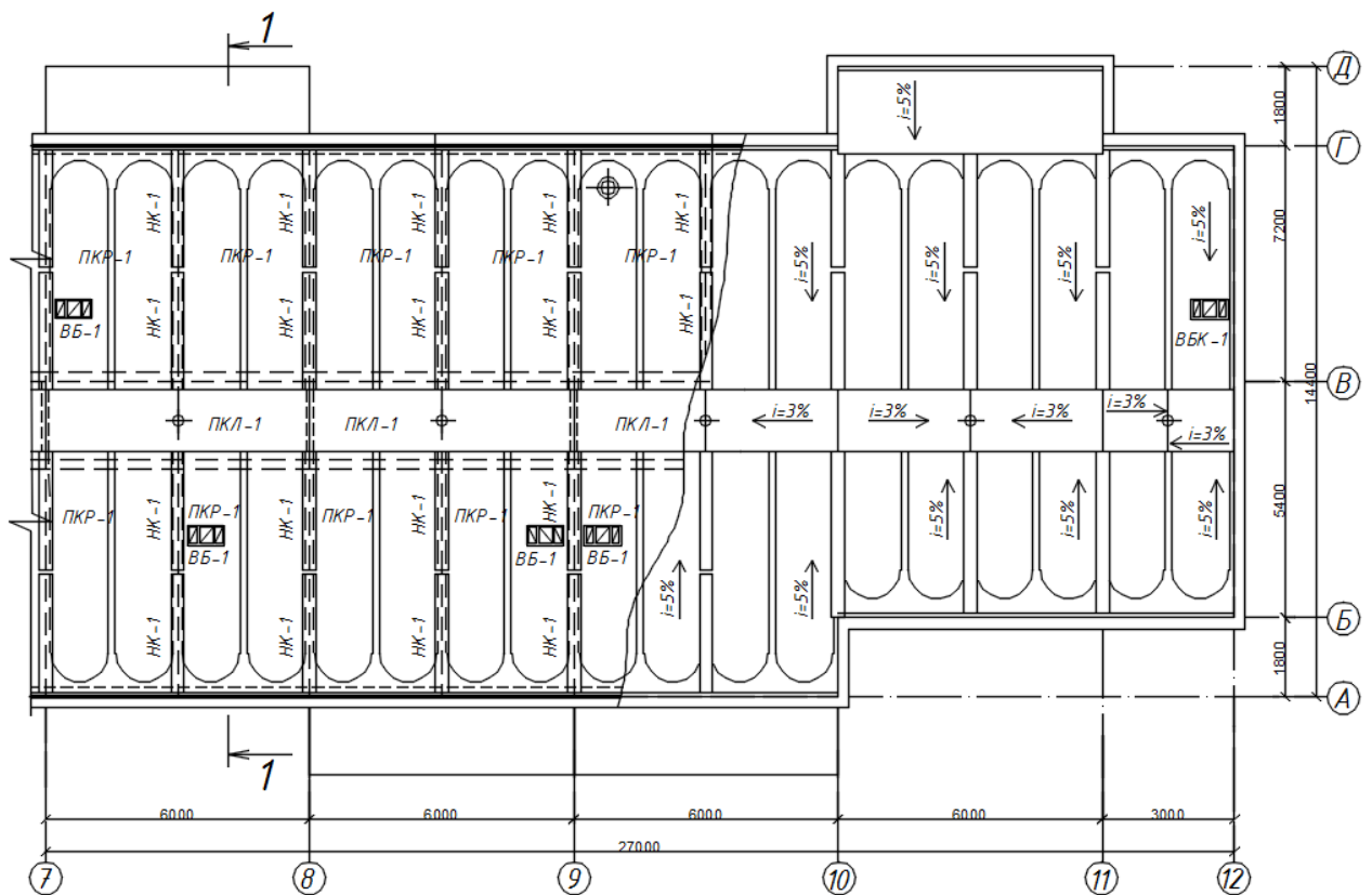
Рис. 2.4. Холодный чердак и безрулонная кровля. План кровли ПКРЧ: ПКЛ – панель кровельная и лотковая; ВБ – вентиляционный блок; НК – нащельник кровельный
