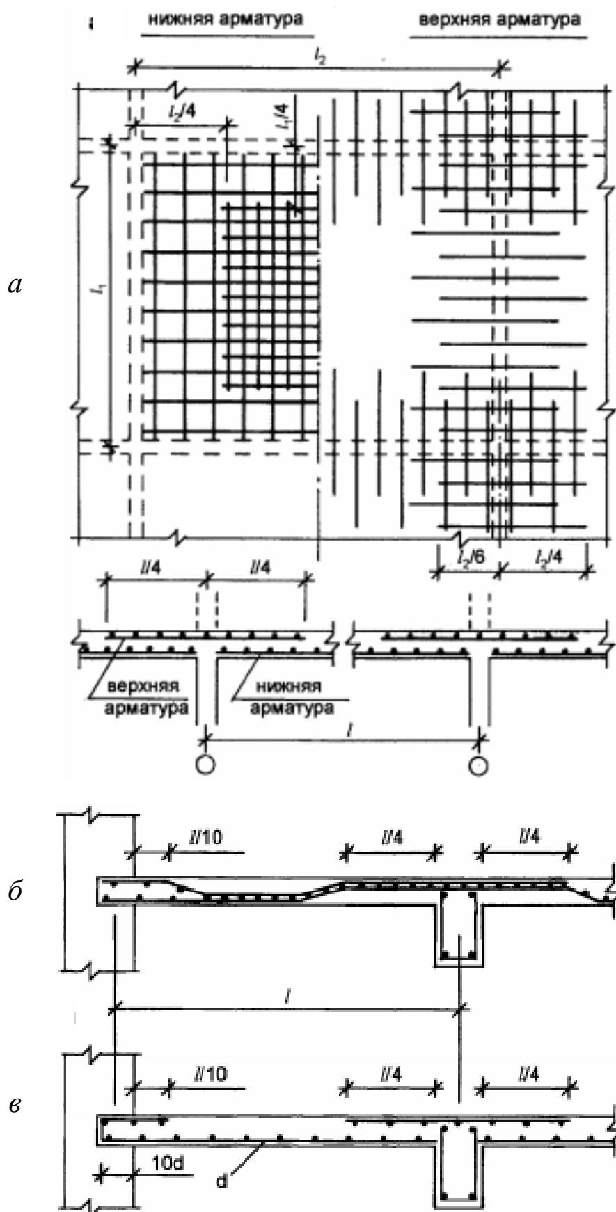
Рис. 5.8. Армирование монолитных перекрытий: а – с плоскими плитами, опертыми по контуру; б – с балочными плитами, рулонными сварными сетками; в – то же с плоскими сварными каркасами [14, с. 97]
