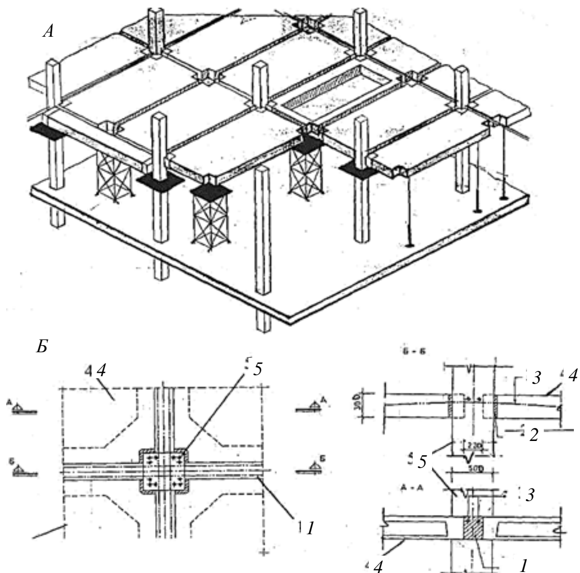
Рис. 3.10. Каркас со скрытыми ригелями (КПНС): А – схема сборки; Б – узел плана перекрытия у колонны; 1 – монолитный ригель; 2 – шов омоноличивания; 3 – канатная натяжная арматура; 4 – плита перекрытия; 5 – колонна
