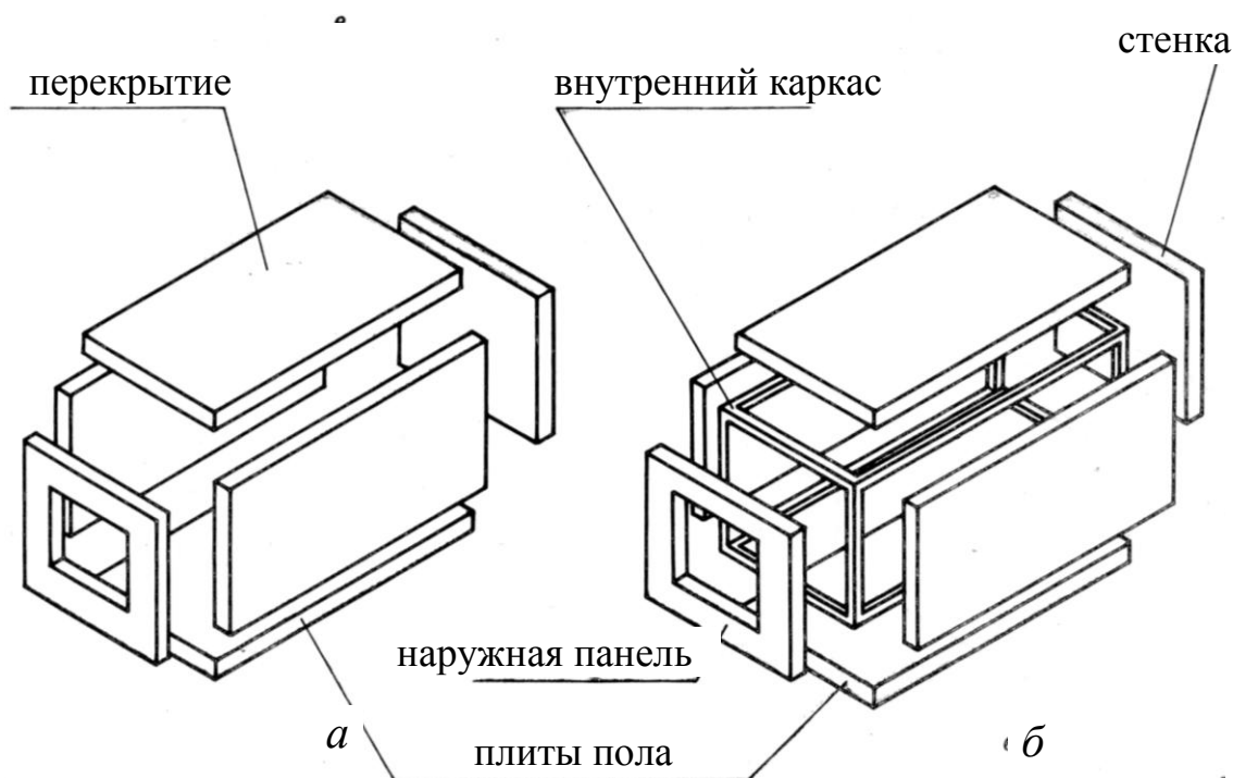
Рис. 4.9. Типы рядовых объемных блоков: a – собираемый из отдельных сборных элементов; б – сборный с каркасным остовом [6, с. 83]
