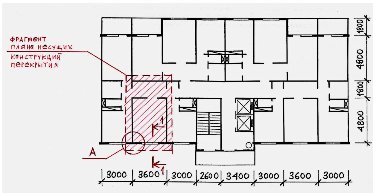
Рисунок 2.1. Пример схемы планировки типового этажа
