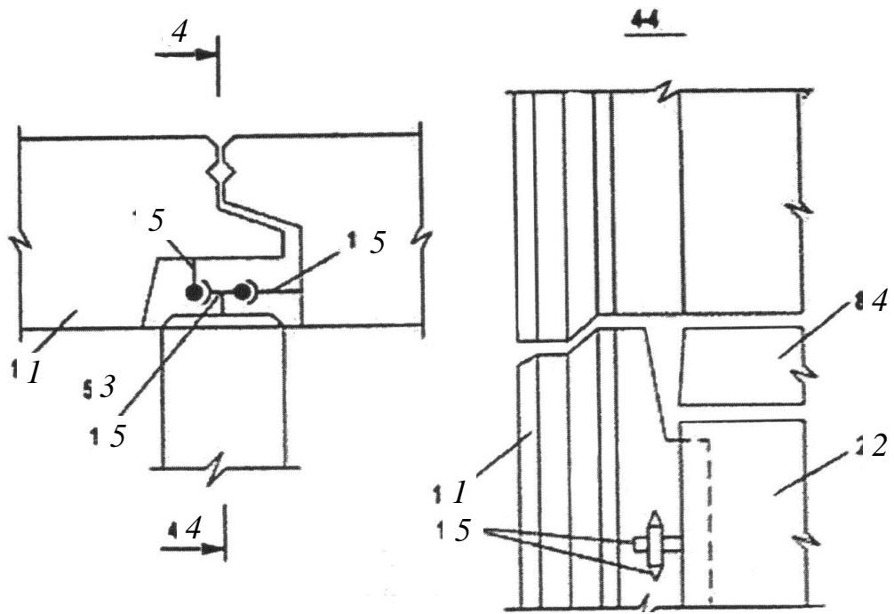
Рис. 2.29. Самофиксирующая связь замкового типа: 1 – панель наружной стены; 2 – панель внутренней стены; 3 – бетон замоноличивания; 4 – панель перекрытия; 5 – закладные связи самофиксации
