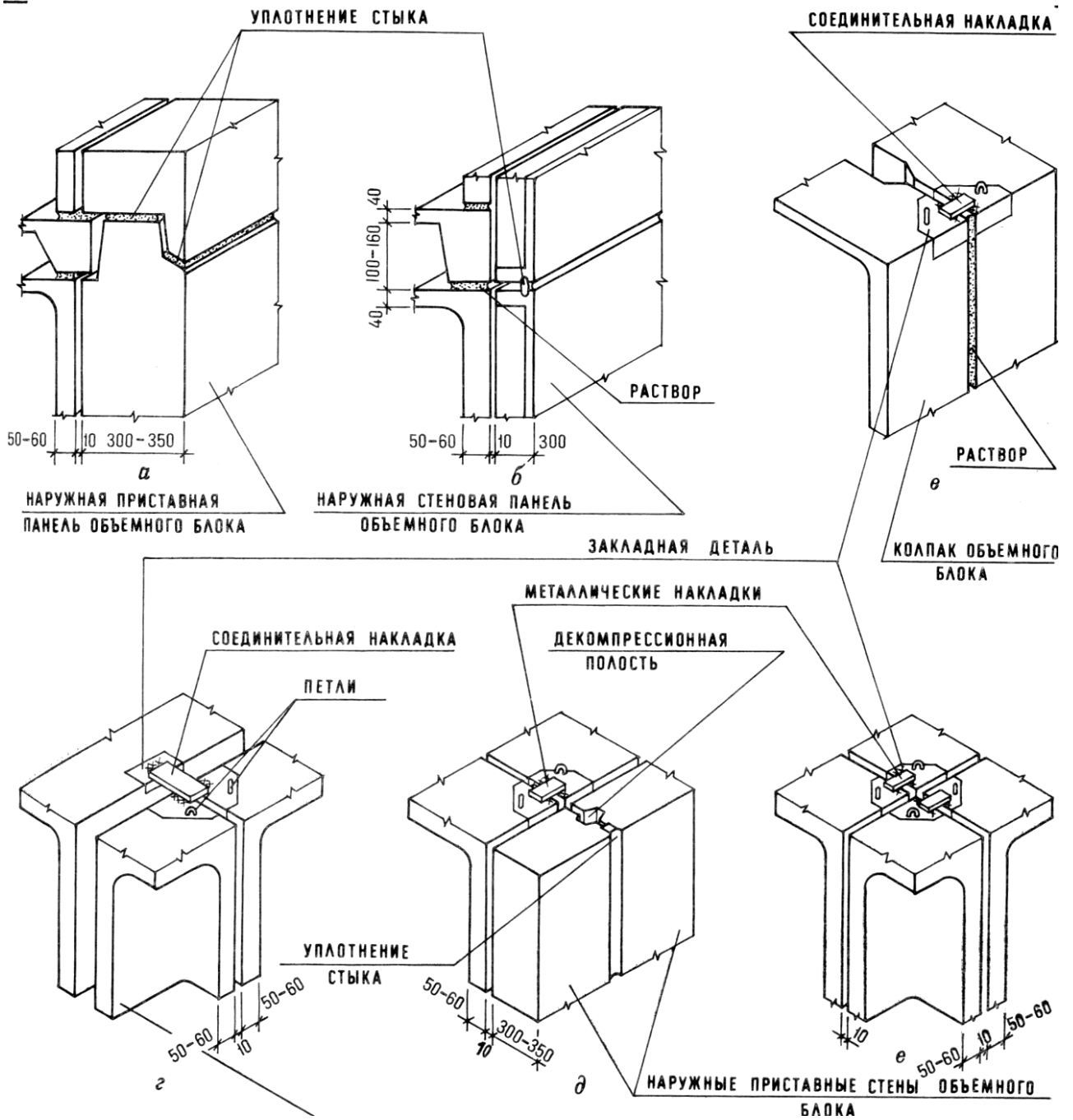
Рис. 4.13. Узлы соединения элементов объемно-блочных зданий: а – объемного блока с наружной стеной при однослойной конструкции наружной панели; б – то же при двухслойной, в – рядовое соединение объемных блоков; г – то же со сдвижкой блоков; д – блоков по наружным стенкам; е – блоков внутренних (четных блоков)
