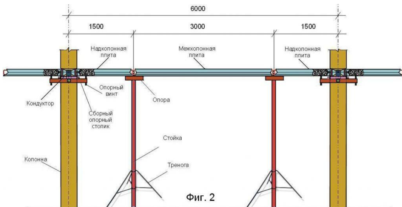
Рис. 3.8. Система безригельного каркаса (КУБ)
