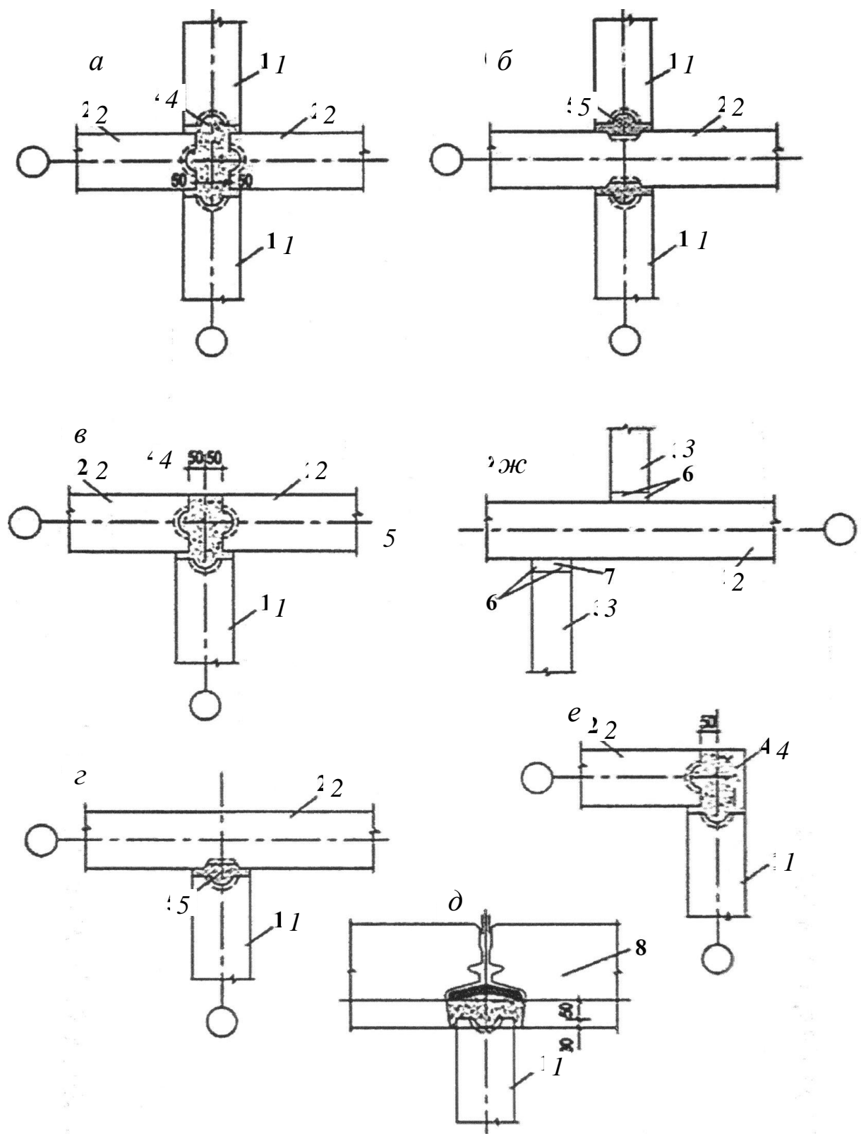
Рис. 2.22. Вертикальные стыки панелей внутренних стен и перегородок: a-e – стыки несущих панелей между собой и с наружной стеной; ж – стык ненесущих перегородок со стеновой панелью; 1 и 2 – напели поперечных и продольных внутренних стен; 3 – панель перегородки; 4 – бетон замоноличивания; 5 – шпоночные рифления стыковых граней панелей; 6 – упругие прокладки; 7 – раствор; 8 – панель наружной стены
