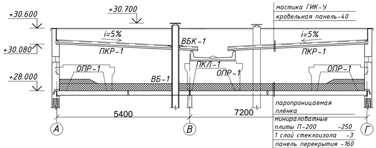
Рис. 2.5. Холодный чердак и безрулонная кровля (поперечный разрез 1 : 1): ВБ – вентиляционный блок; ВБК – вентиляционный блок крышный; ОПР – опорная рама; ПКР и ПКЛ – панель кровельная и лотковая;
