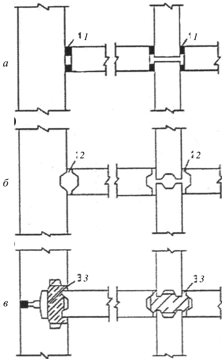
Рис. 2.20. Типы вертикальных стыков панельных стен: а – плоские; б – профилированные бесшпоночные; в – профилированные шпоночные; 1 – звукоизоляционная прокладка; 2 – раствор; 3 – бетон замоноличивания стыка
