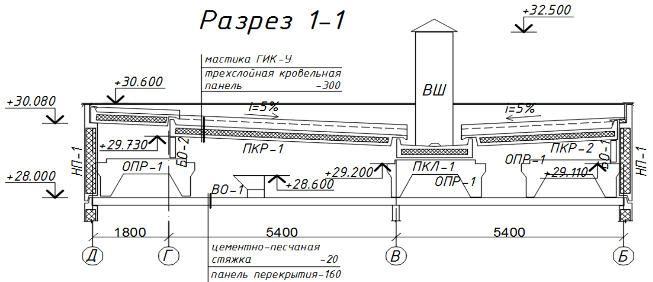
Рис. 2.9. Теплый чердак и безрулонная кровля (поперечный разрез): ВО – Вентиляционный оголовок; ОПР – опорная рама; БО – балка опорная; НП – наружная фризловая панель; ПКР и ПКЛ – панель кровельная ребристая и лотковая; ВШ – общая вытяжная шахта
