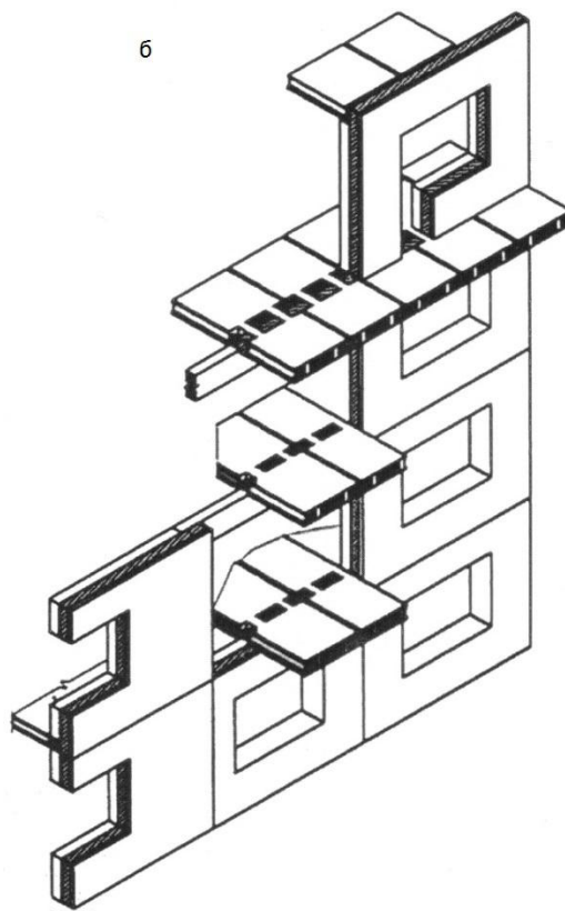
Рис. 2.3.: a – плита пустотная с многопустотными усилителями; б – плита пустотная с многопустотными усилителями в панельном здании
