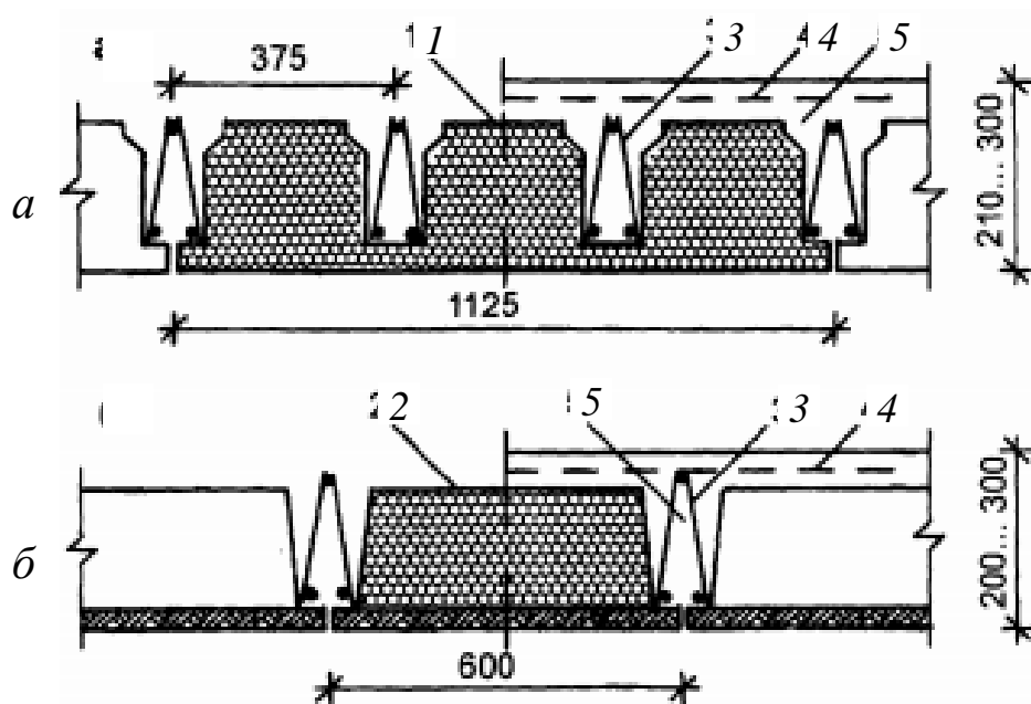
Рис. 5.9. Теплоизолированные монолитные железобетонные ребристые перекрытия: a – с применением пенополистирольных профилированных элементов; б – с применением комбинированных элементов из цементностружечной нижней и пенополистирольной верхней частей; 1 – пенополистирольный элемент межбалочного заполнения; 2 – комбинированный элемент; 3 – арматурный каркас; 4 – арматурная сетка; 5 – бетон замоноличивания
