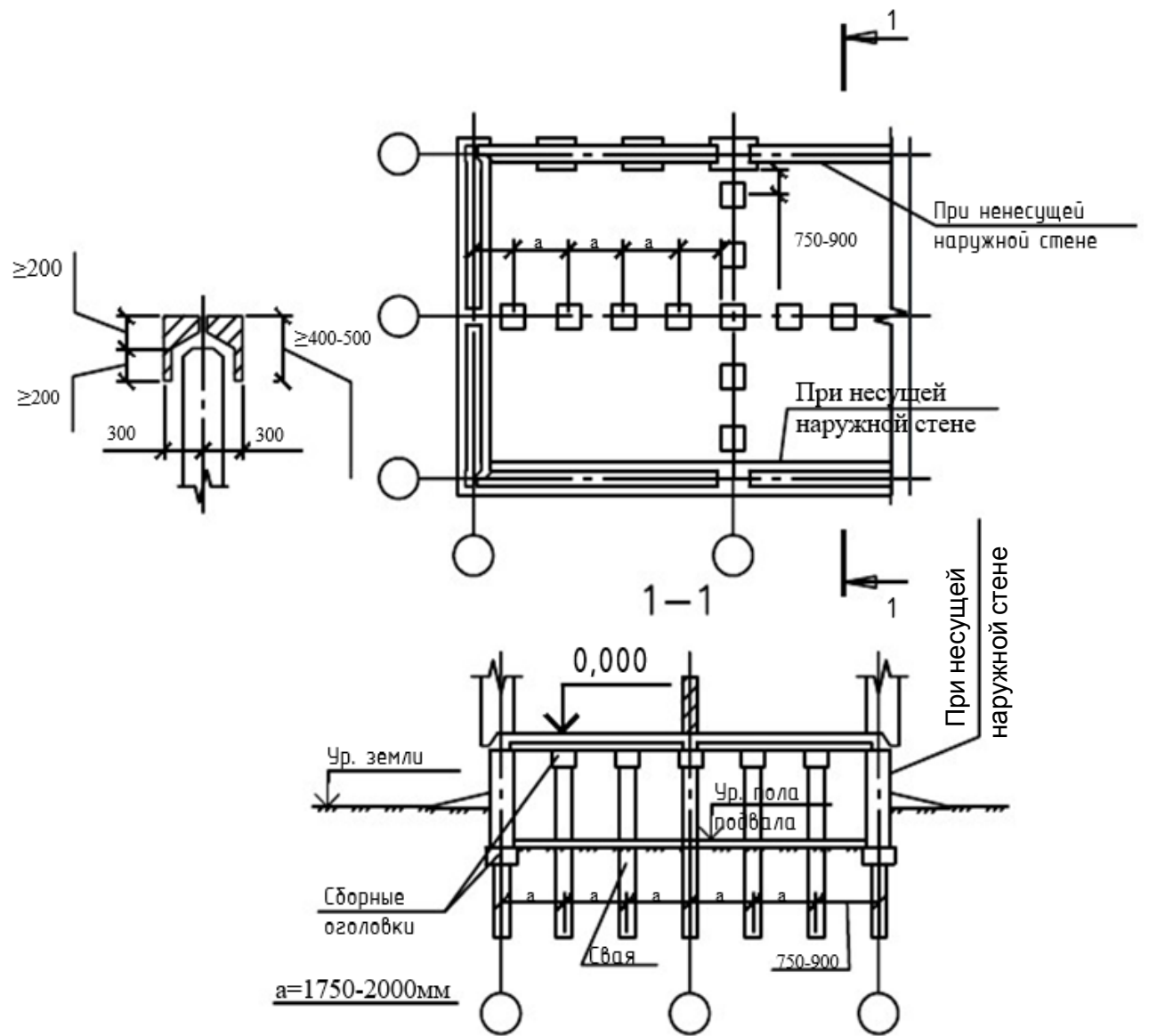
Рис. 2.14. Схема безростверкового свайного фундамента со сборными оголовками
