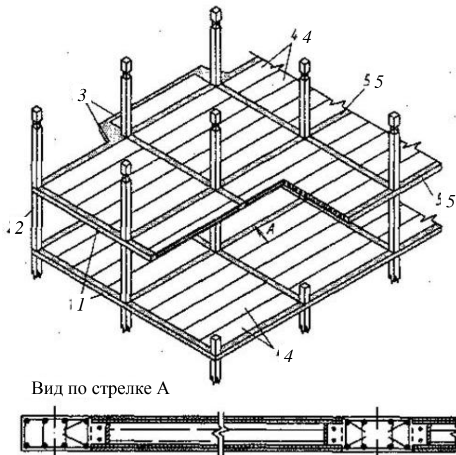
Рис. 3.7. Сборно-монолитный каркас
