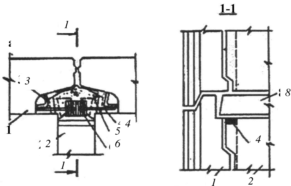
Рис. 2.26. Сварная связь:
