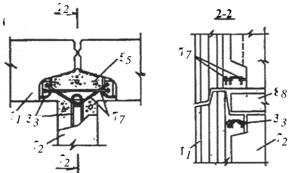
Рис. 2.27. Замоноличиваемая связь типа петля-скоба: 1 – панель наружной стены; 2 – панель внутренней стены; 3 – петлевой арматурный выпуск; 5 – бетон замоноличивания; 7 – стальная накладка; 8 – панель перекрытия
