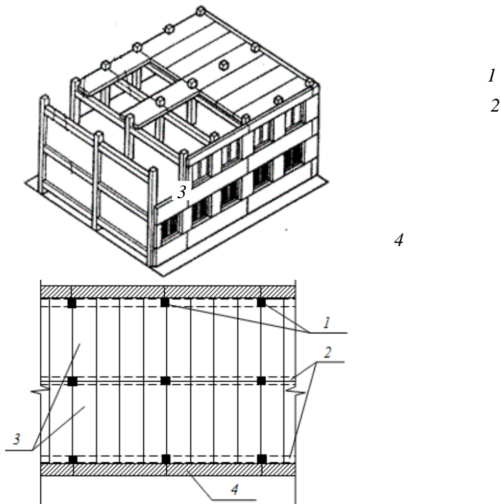
Рис. 3.1. Каркасная конструктивная система: 1 – колонны каркаса; 2 – ригели каркаса; 3 – сборный настил перекрытия; 4 – наружная навесная стеновая панель
