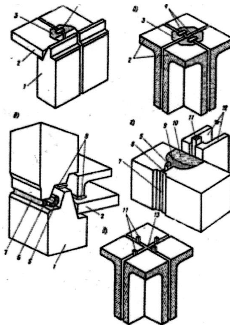
Рис. 4.11. Сопряжение блоков в наружной (а) и во внутренней (б) части зданий: наружные горизонтальный (в) и вертикальный (г) стыки; внутренний вертикальный стык (д):
