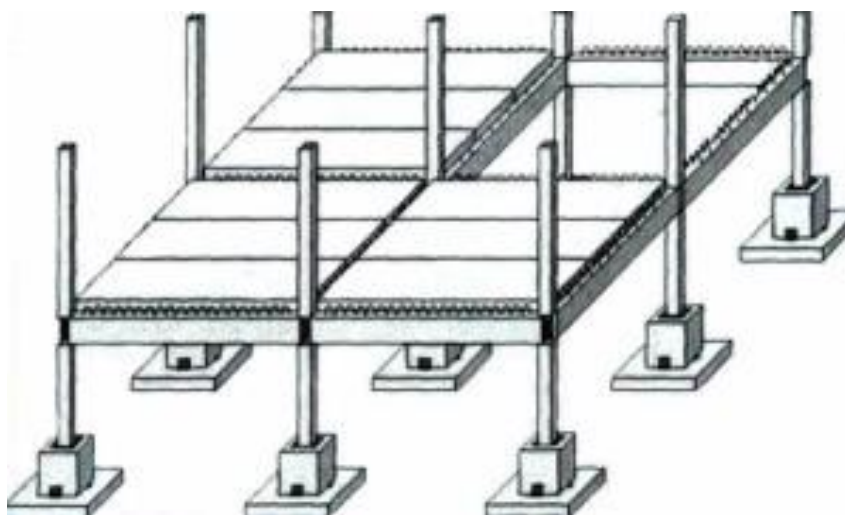
Рис. 3.4. Схема сборного железобетонного каркаса
