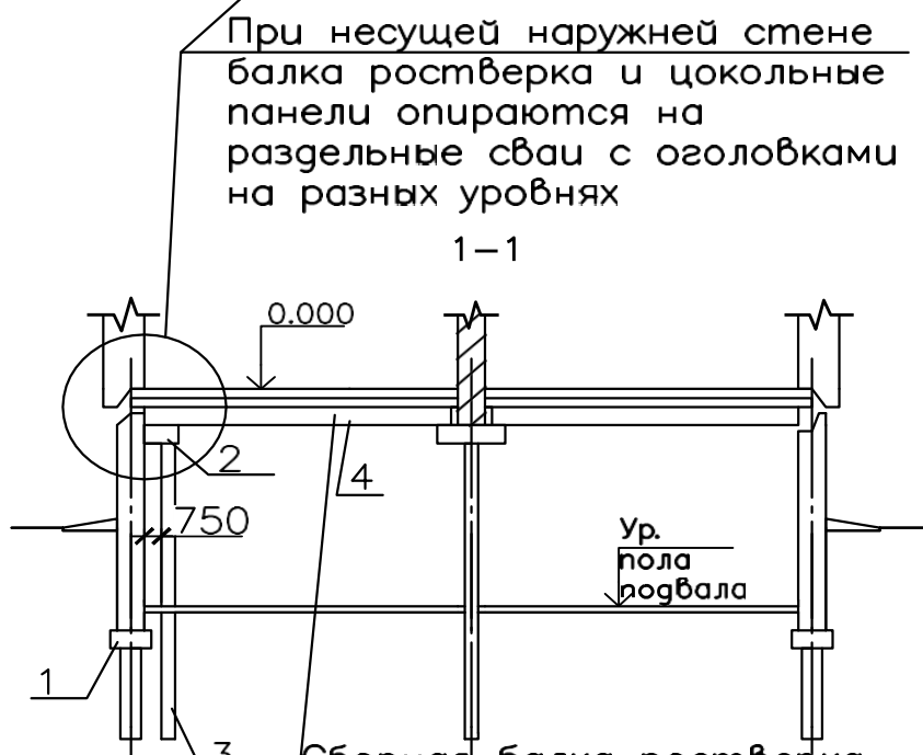
Рис. 2.15. Схема свайного фундамента с высоким сборным ростверком: 1 – монолитный ростверк; 2 – сборный ростверк; 3 – сборная железобетонная свая; 4 – сборная железобетонная балка ростверка
