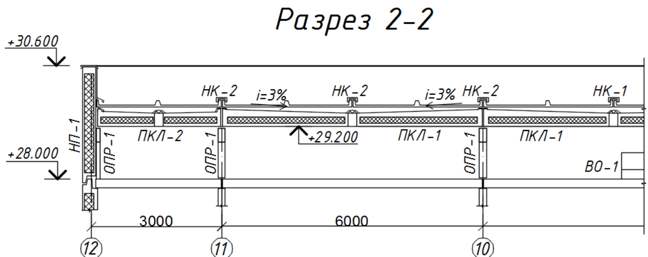
Рис. 2.10. Теплый чердак и безрулонная кровля. Продольный разрез: НП – наружная фризловая панель; НК – нащельник кровельный; ПКЛ – панель кровельная лотковая; ВО – вентиляционный оголовок; ОПР – опорная рама
