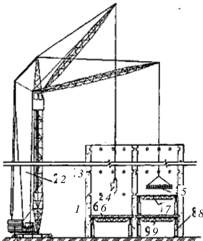
Рис. 5.2. Бетонирование междуэтажных перекрытий методом «снизу вверх»: 1 – монолитные стены; 2 – кран; 3 – оставленные при бетонировании гнезда; 4 – бадья для подачи бетонной смеси; 5 – армокаркас; 6 – опалубка перекрытия; 7 – ферменный прогон; 8 – телескопическая стойка; 9 – монолитное перекрытие [31, с. 320]
