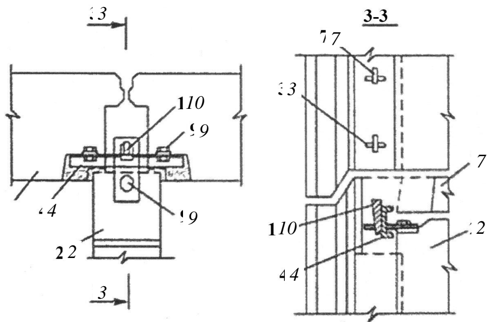
Рис. 2.28. Болтовая связь: 1 – панель наружной стены; 2 – панель внутренней стены; 3 – петлевой арматурный выпуск; 4 – стыковая накладка; 7 – стальная скоба; 8 – панель перекрытия; 9 – болтовая связь; 10 – стальной клин
