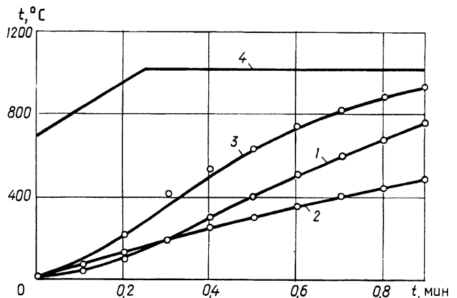
Рис. 1. Сравнение аналитических и численных решений задачи нагрева проволоки в печи патентирования: 1 — нагрев излучением; 2 — конвективный нагрев; 3 — радиационно-конвективный нагрев; 4 — температура печи
