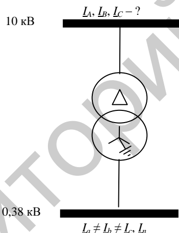
Рис. 2. Трехфазный двухобмоточный трансформатор 10/0,38 кВ
