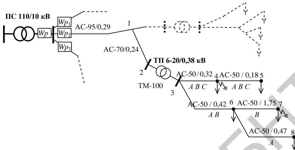
Рис. 1. Схема электрической сети 0,38–10 кВ с цифровыми приборами учета: W_p – на низковольтном вводе 6–10 кВ; W_{p1} , W_{p2} , W_{p3} – на отходящих линиях 6–10 кВ
