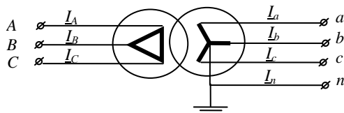
Рис. 3. Несимметричная трехфазная токовая нагрузка трансформатора 10/0,38 кВ
