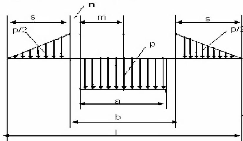
Рисунок 2.2 – Расчетная схема определения напряжения изгиба в поршневом пальце ДВС.
