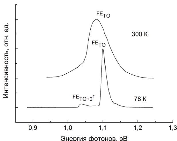
Рисунок 2 – Спектры электролюминесценции эталонных кремниевых p-n структур, измеренные при прямом токе 10 мА для различных температур. Спектральное разрешение 3 нм
