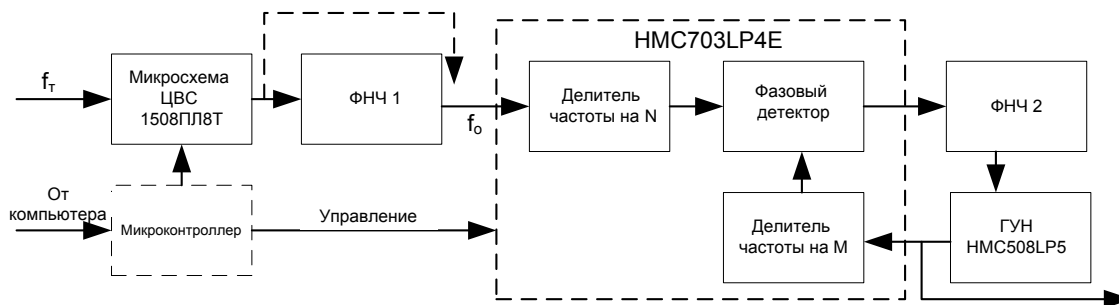
Рисунок 1 – Схема умножения частоты на петле фазовой автоподстройки частоты
