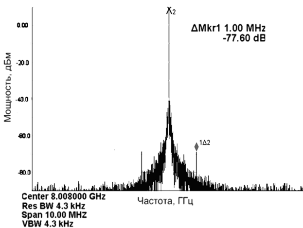
Рисунок 3 – Спектр сигнала:
