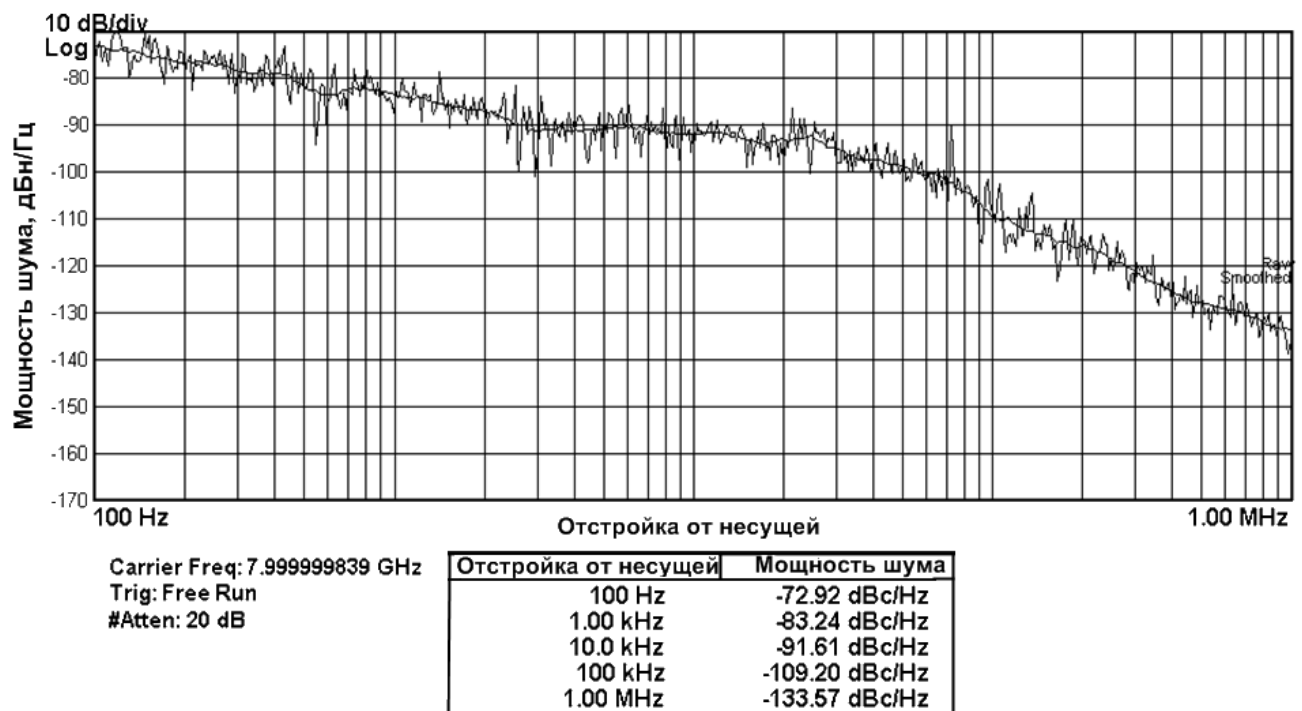
Рисунок 2 – Фазовые шумы при работе: а – от опорного генератора; б – от цифрового вычислительного синтезатора
