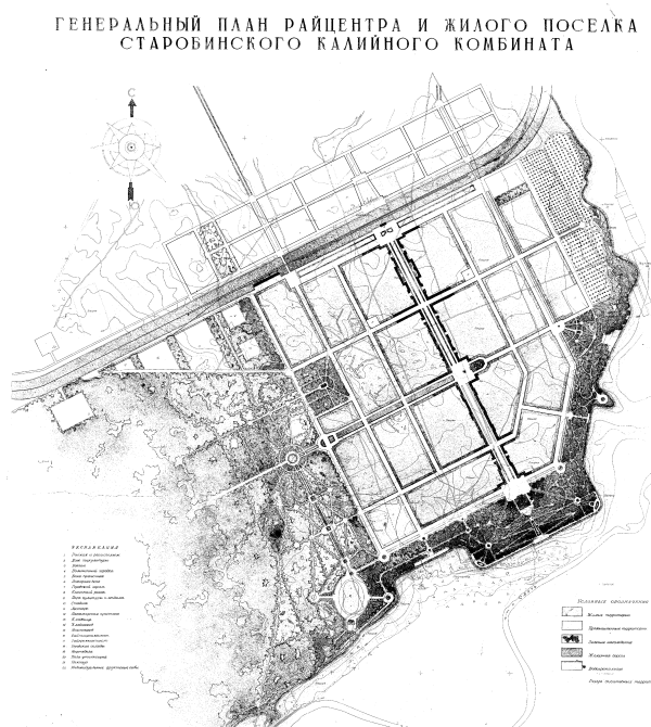
Рис 1. Планировка жилой зоны рабочего поселка Старобинского калийного комбината (арх. Г.А. Парсаданов)
