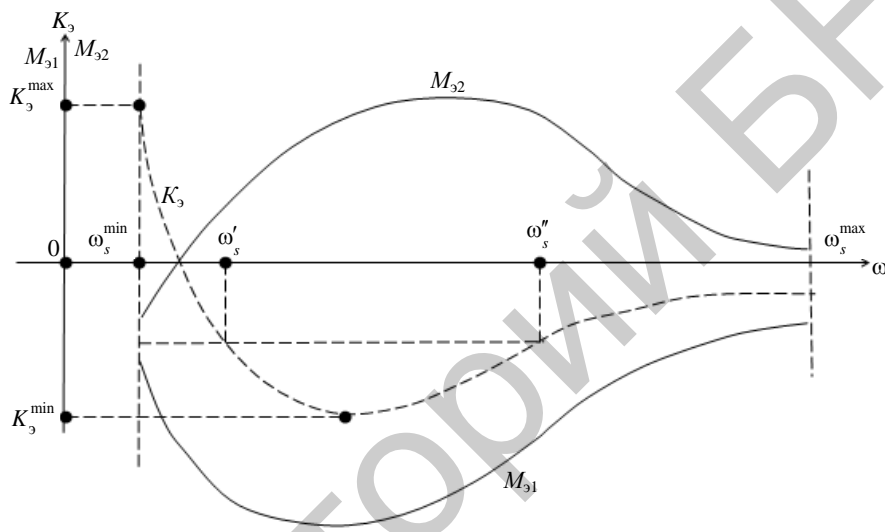
Рис. 3. Зависимость M_{s1} , M_{s2} и M_{s2}/M_{s1} от частоты напряжения статора
