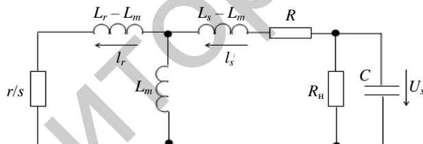
Рис. 1. Схема замещения ААГ в стационарном режиме: R(r) – активное сопротивление статорной (роторной) обмотки; L_s ( L_r ) – индуктивность рассеяния статорной (роторной) обмотки; L_m – взаимная индуктивность; s – скольжение; R_n – сопротивление нагрузки; C – емкость самовозбуждения
