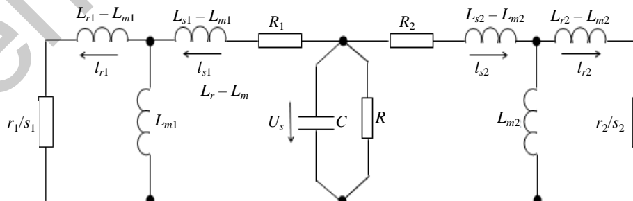
Рис. 2. Схема замещения АДС в стационарном режиме
