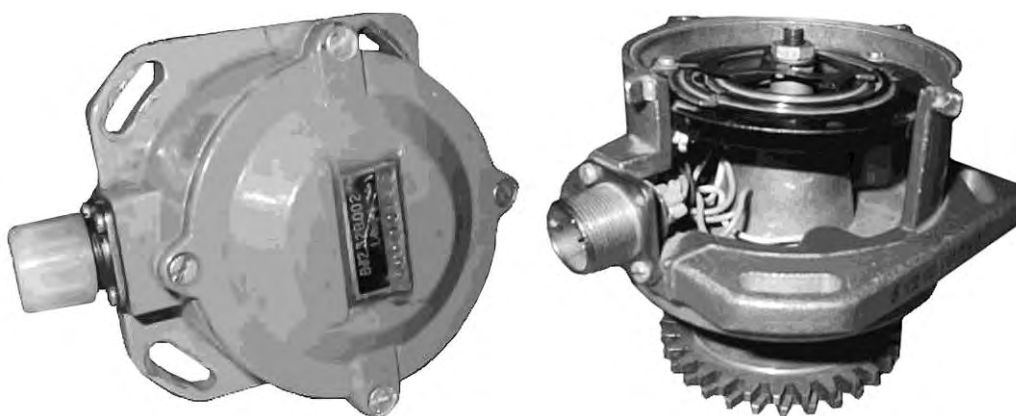
Рис. 5.39. Прибор приведения
