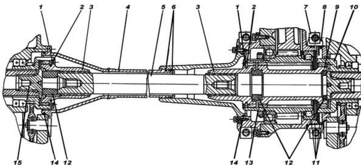
Рис. 9.3. Соединение гитары с правой и левой КП:
