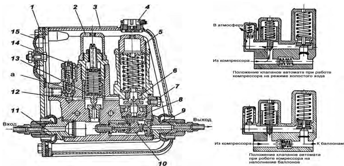
Рис. 8.40. Автомат давления АДУ-2С:
