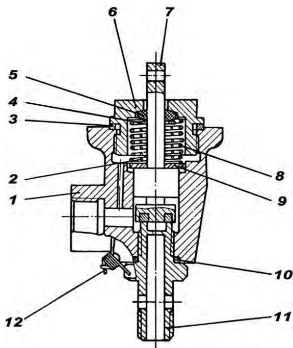
Рис. 8.36. Топливный кран подогревателя:
