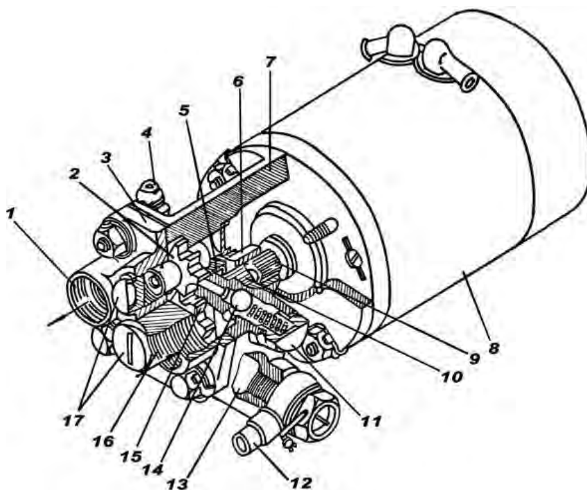
Рис. 8.25. Маслозакачивающий насос МЗН-2:
