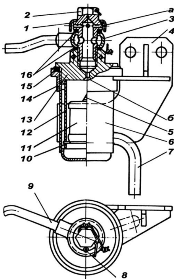
Рис. 8.3. Поплавковый клапан:
