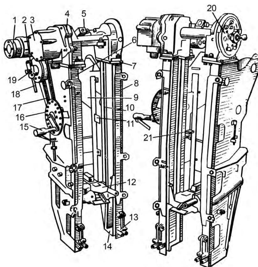
Рис. 5.72. Механизм подъема кассет:
