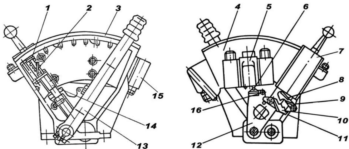
Рис. 9.10. Избиратель передач
