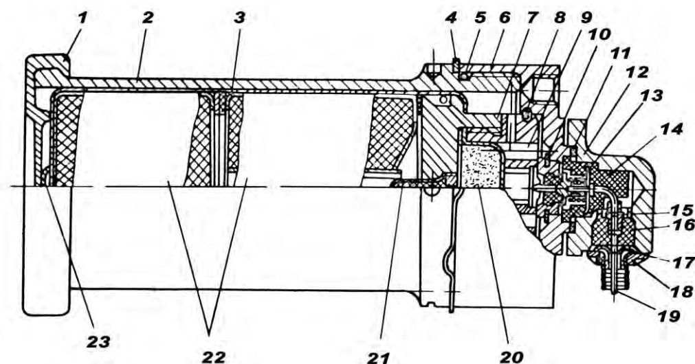
Рис. 5.19. Пусковая установка с дымовой гранатой:
