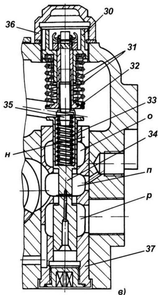
Рис. 9.15. Механизм распределения (окончание):
