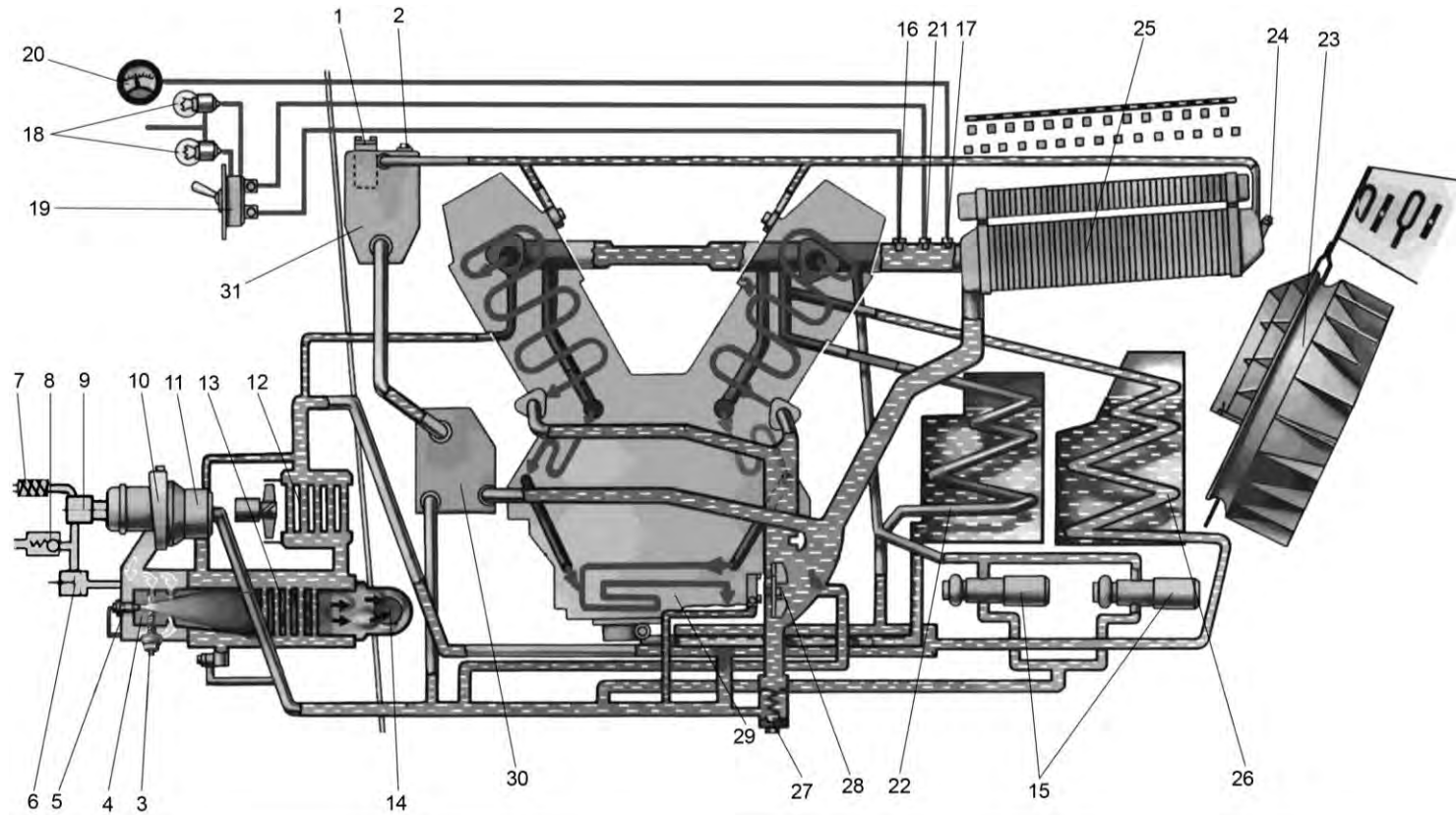
Рис. 8.27. Система охлаждения и подогрева. Схема гидравлическая принципиальная:
