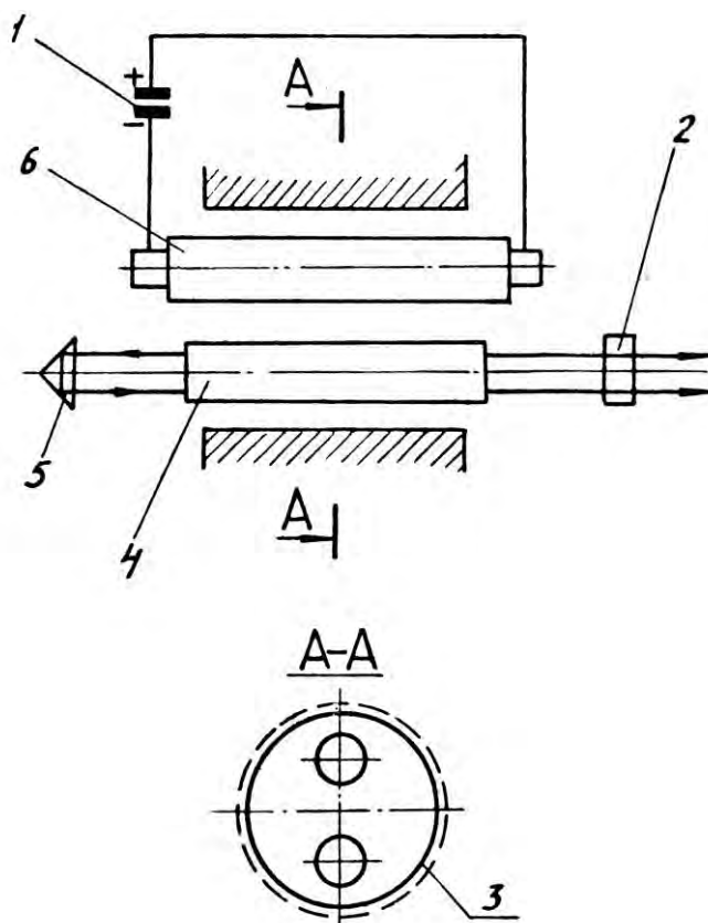
Рис. 5.34. Схема оптического квантового генератора:
