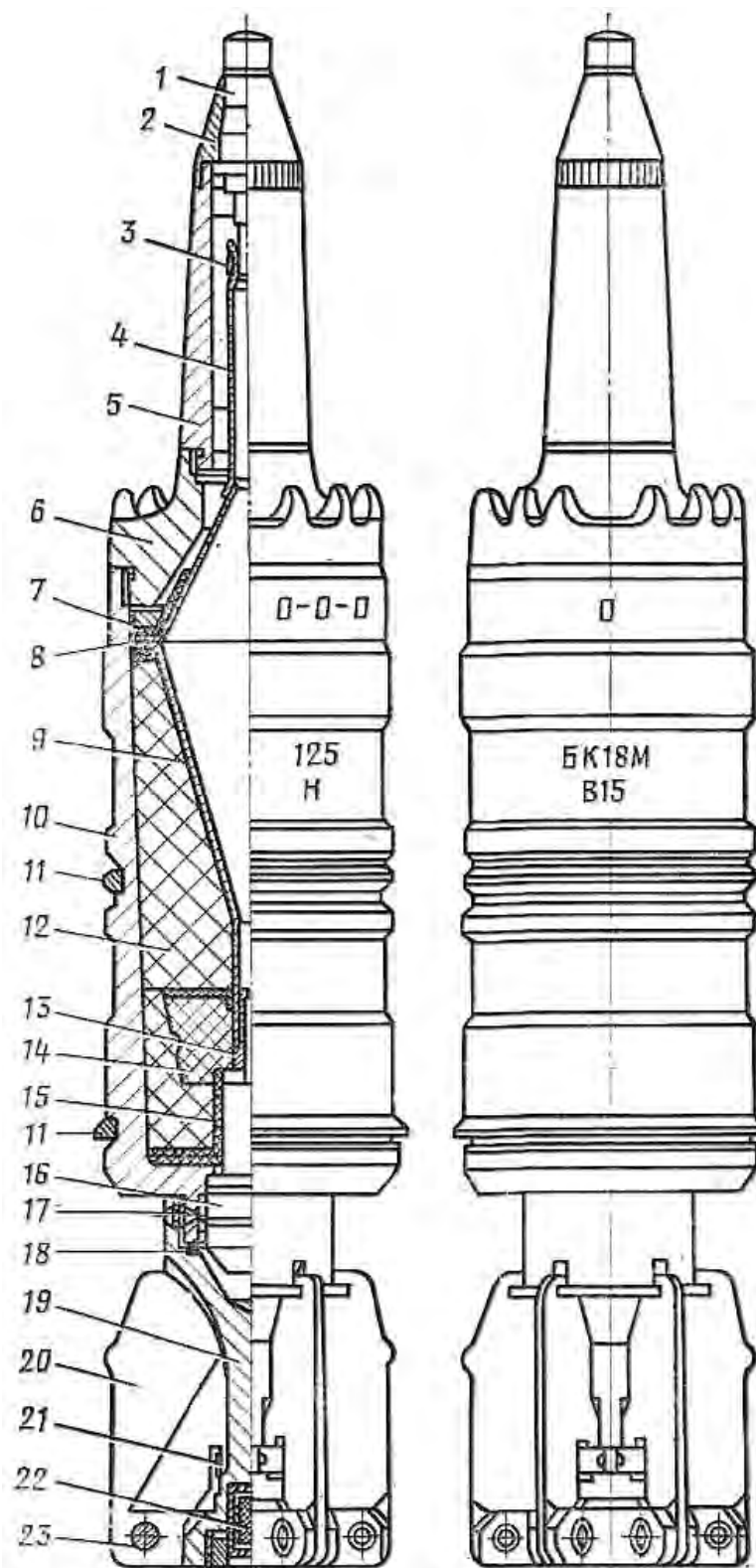
Рис. 5.24. Кумулятивный снаряд ЗБК18М:
