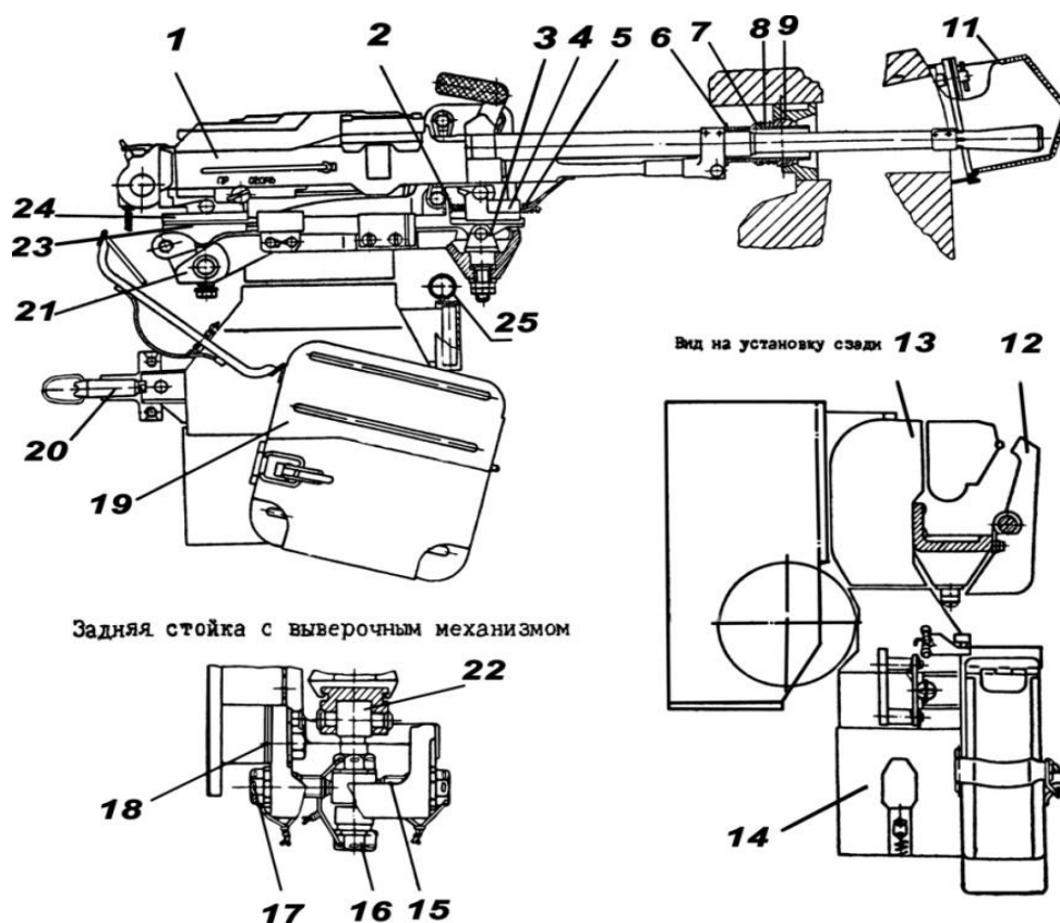
Рис. 5.14. Установка спаренного пулемета ПКТ:
