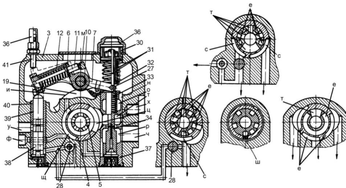
Рис. 9.16. Механизм распределения. Схема каналов:
