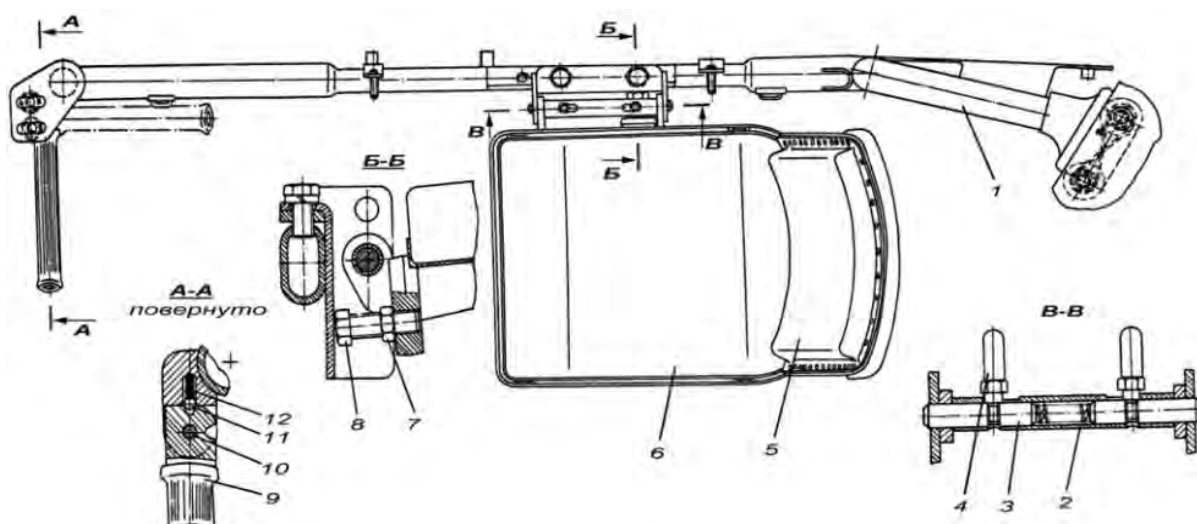
Рис. 4.9. Сиденье наводчика:
