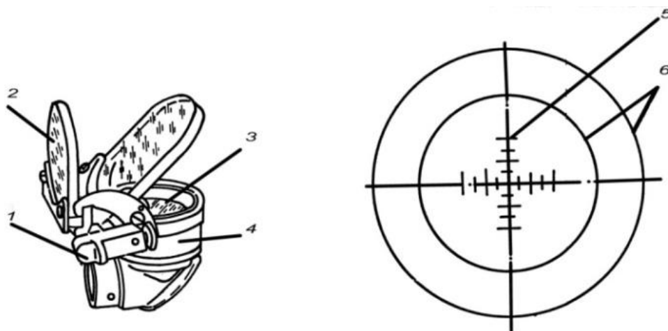
Рис. 5.17. Коллиматорный прицел К10-Т:
