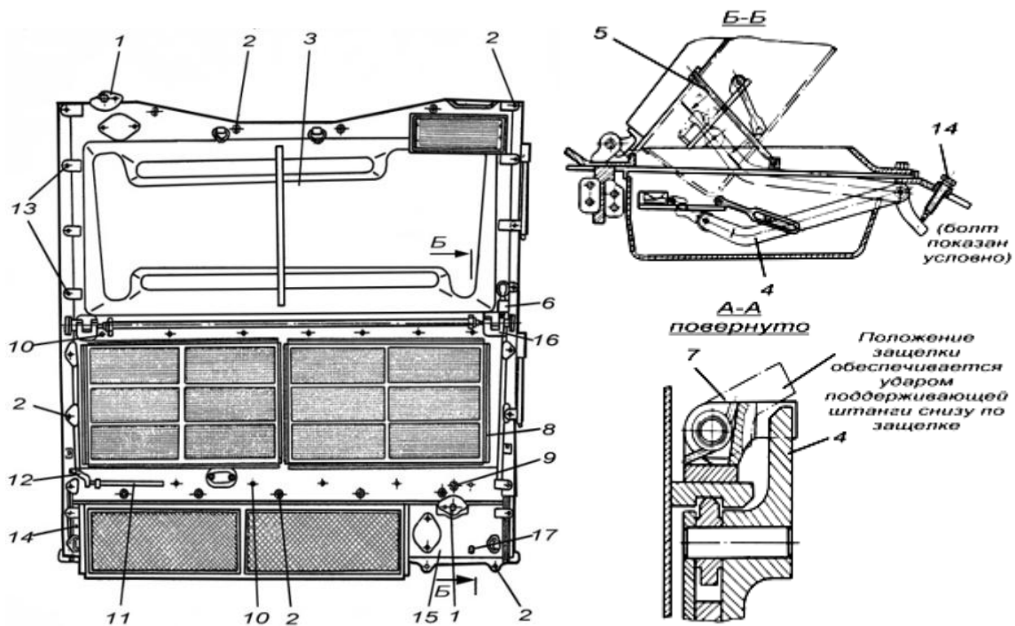
Рис. 4.5. Крыша над силовым отделением:
