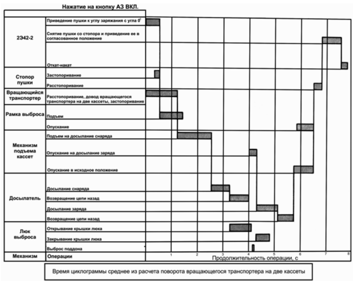
Рис. 5.85. Циклограмма работы АЗ
