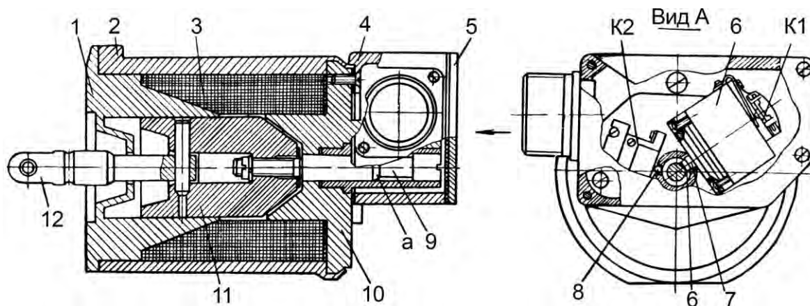
Рис. 5.69. Электромагнит стопора ВТ:
