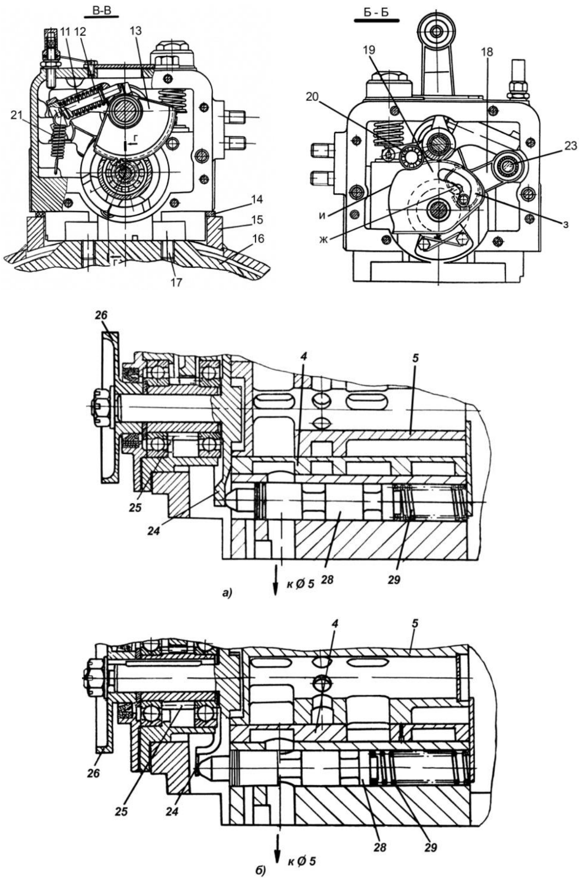
Рис. 9.15. Механизм распределения (продолжение)
