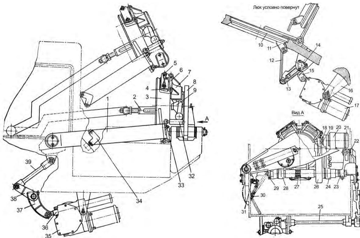
Рис. 5.75. Механизм удаления поддона:
