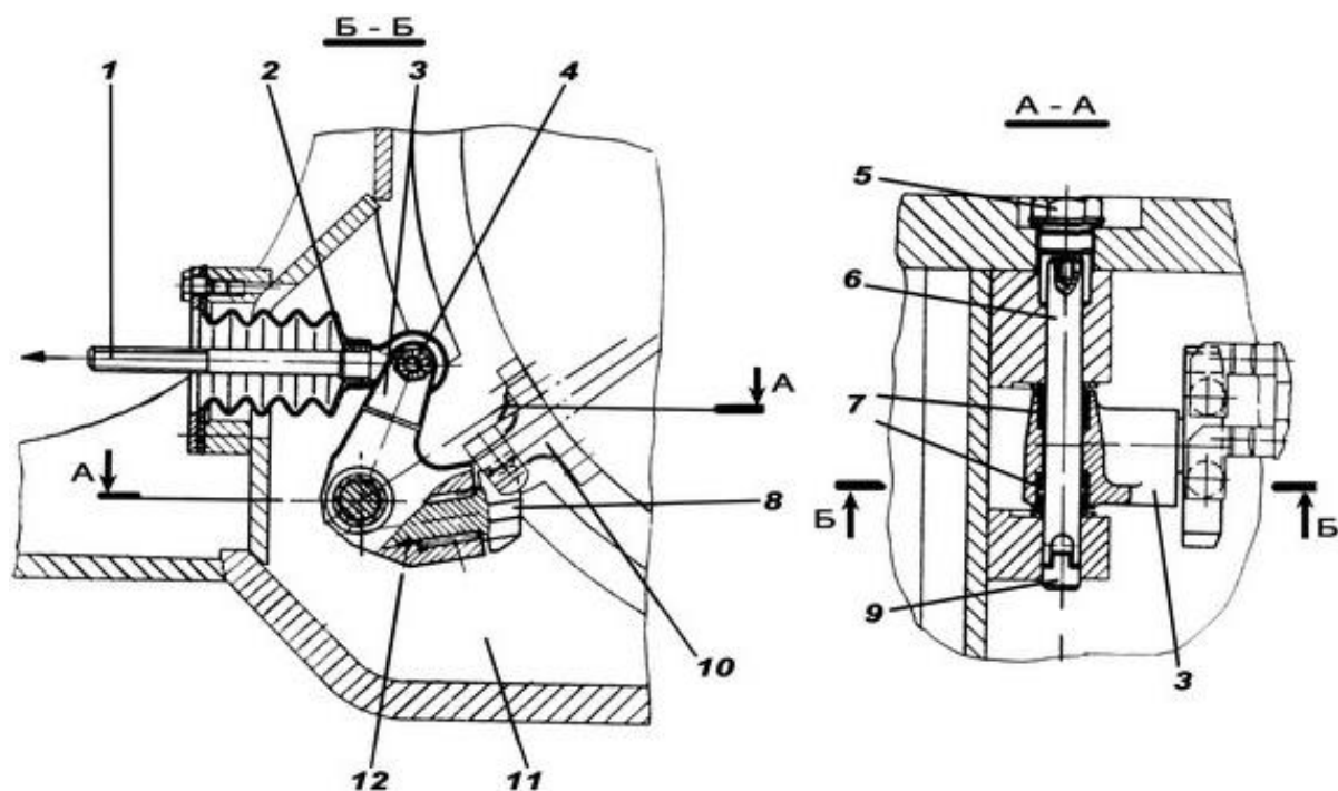
Рис. 9.13. Привод остановочного тормоза правой КП:
