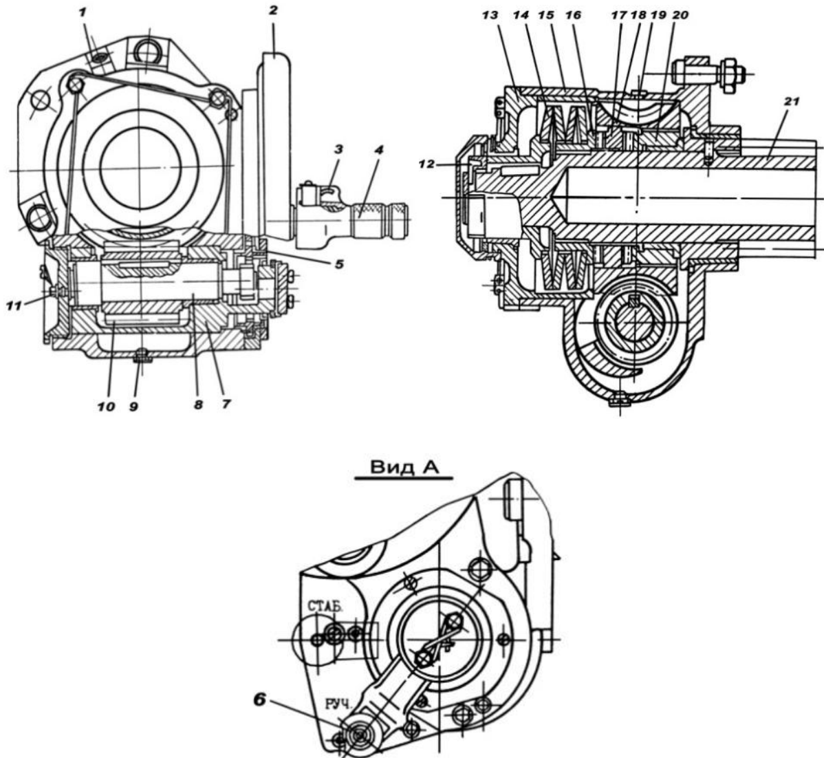
Рис. 5.12. Подъемный механизм пушки (устройство):
