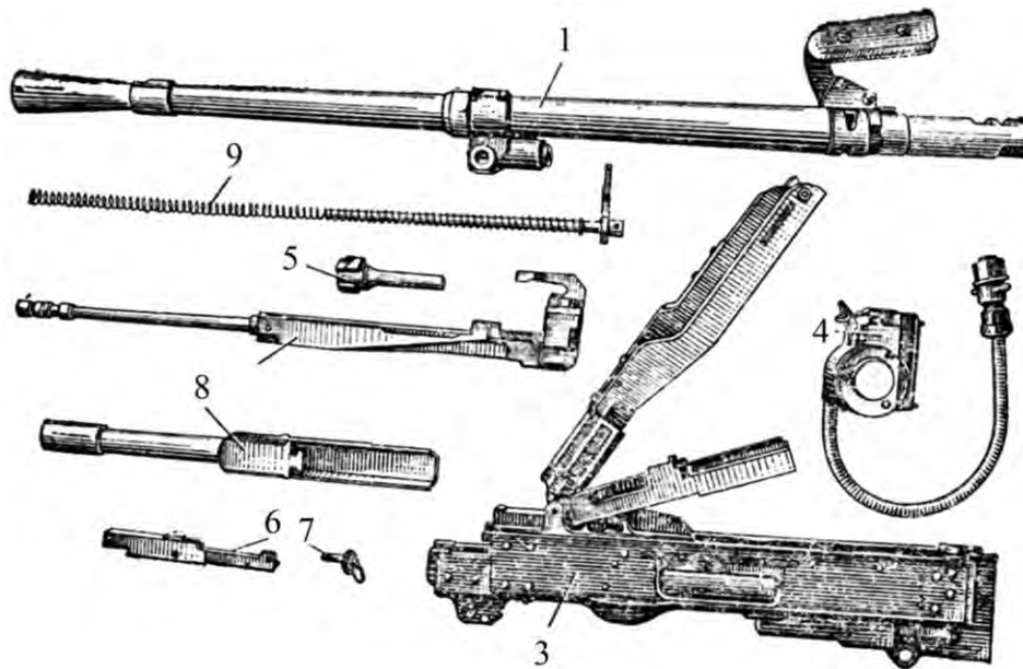
Рис. 5.13. Пулемет ПКТ (общее устройство):
