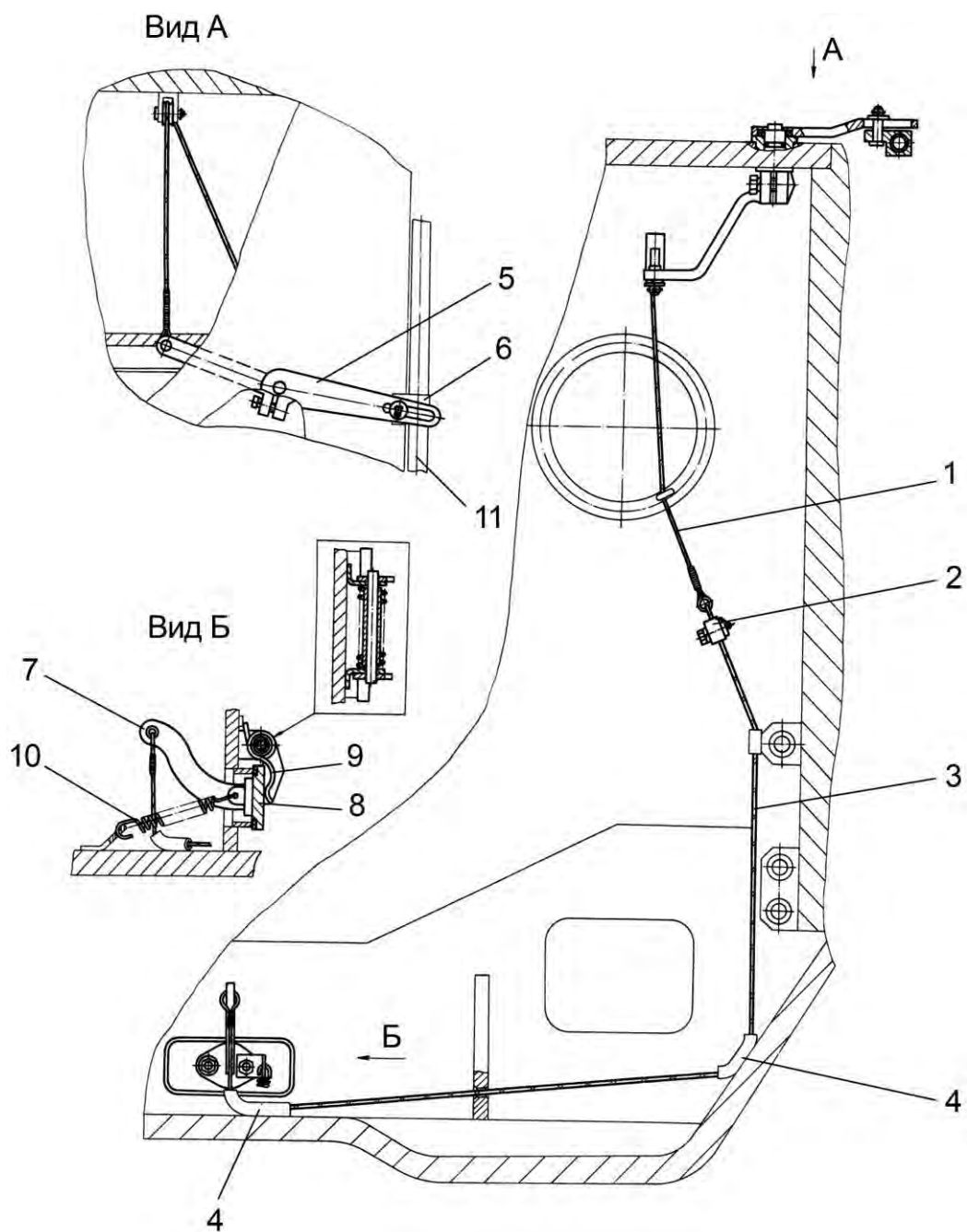
Рис. 16.6. Лючок перетока воды с приводом: 1 – трос; 2 – зажим; 3 – трос; 4 – направляющая трубка; 5 – двуплечий рычаг; 6 – поводок; 7 – рычаг; 8 – крышка; 9, 10 – пружины; 11 – продольная тяга крышек ОПВТ
