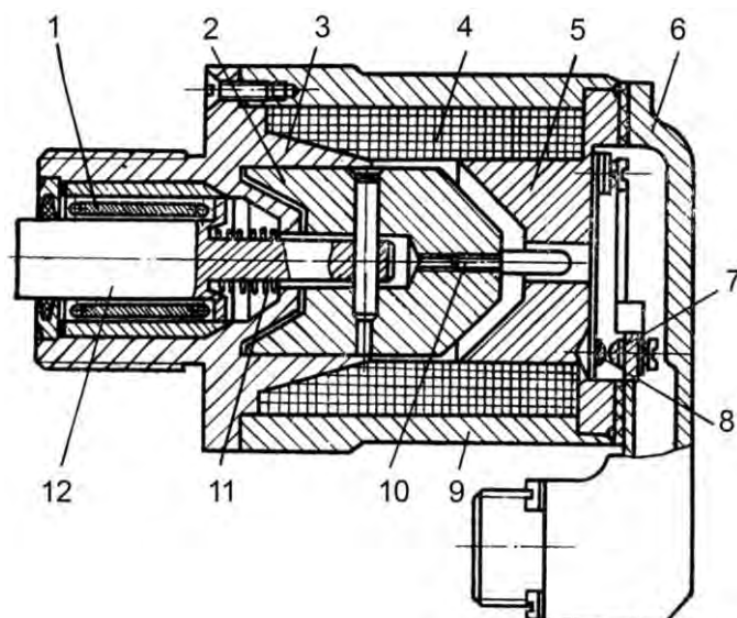
Рис. 5.76. Электромагнитный стопор МУП: 1 – подшипник; 2 – якорь; 3, 6 – крышки; 4 – катушка; 5 – стопы; 7, 8 – неподвижный и подвижный контакты; 9 – корпус; 10 – винт; 11 – пружина; 12 – палец
