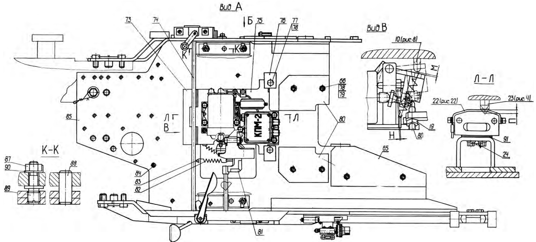
Рис. 5.7. Ограждение (окончание):
