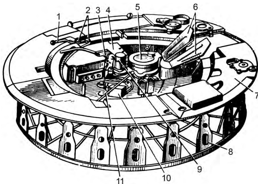
Рис. 5.62. Вращающийся транспортер:
