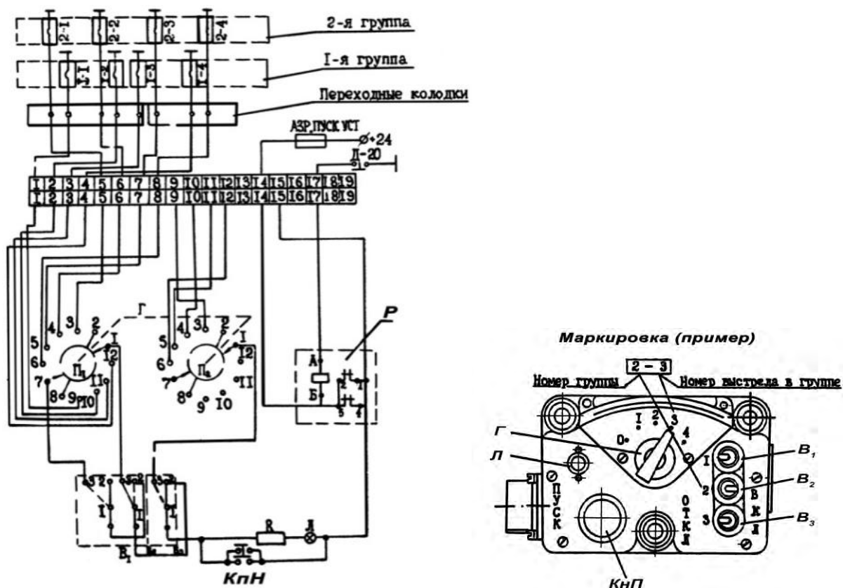
Рис. 5.20. Система пуска дымовых гранат. Схема электрическая и пульт управления: B_1, B_2, B_3 – выключатели залпов; L – контрольная лампа; G – переключатель пусковых установок; KnП – кнопка запуска; P – реле блокировки; Д-20 – датчик люка водителя (люк закрыт)
