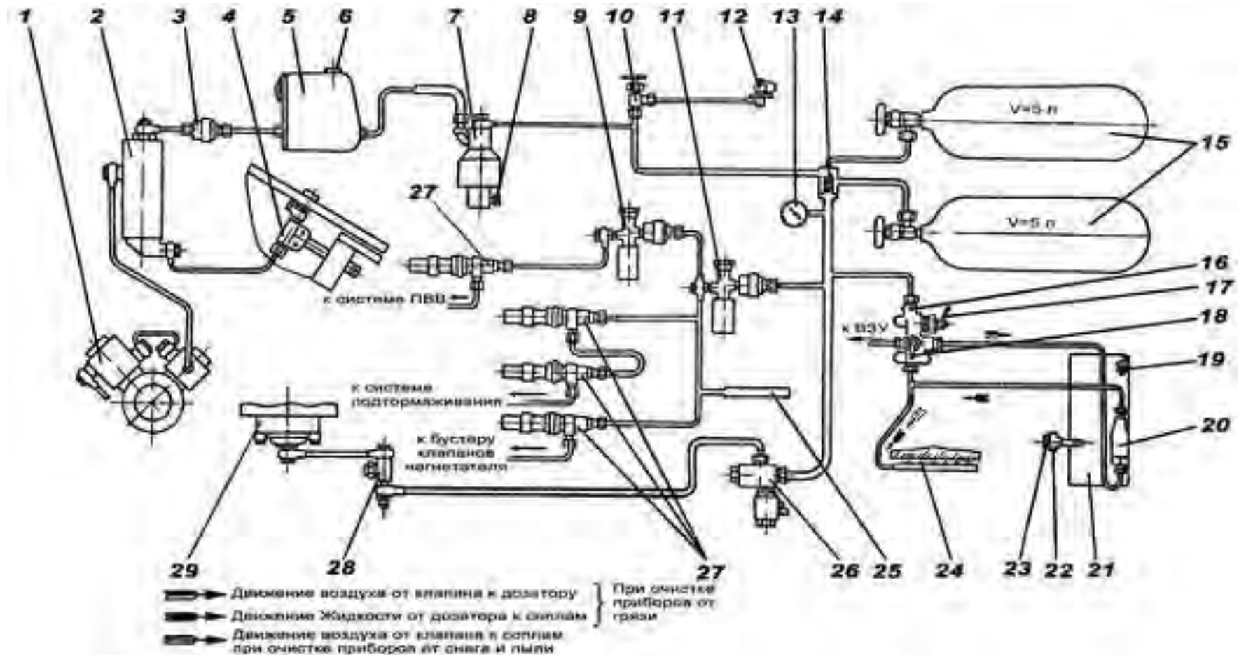
Рис. 8.37. Система воздушная и гидропневмоочистки:
