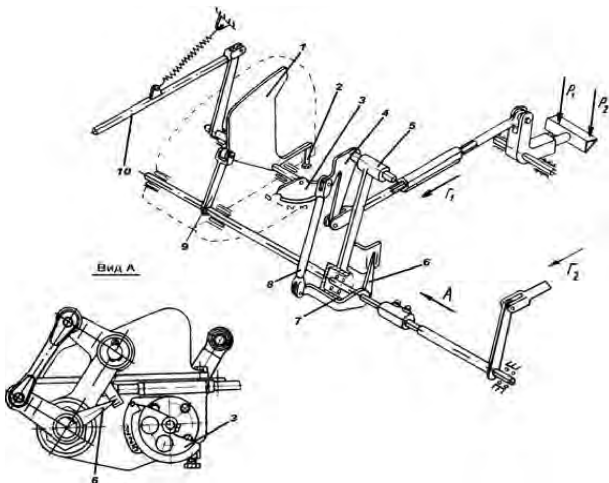
Рис. 9.12. Уравнительное устройство:
