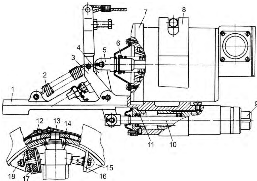
Рис. 5.68. Стопор ВТ:
