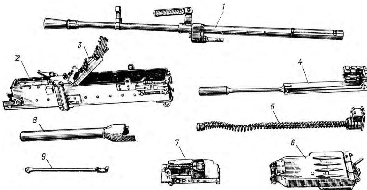
Рис. 5.16. Основные части и механизмы пулемета НСВ-12,7:
