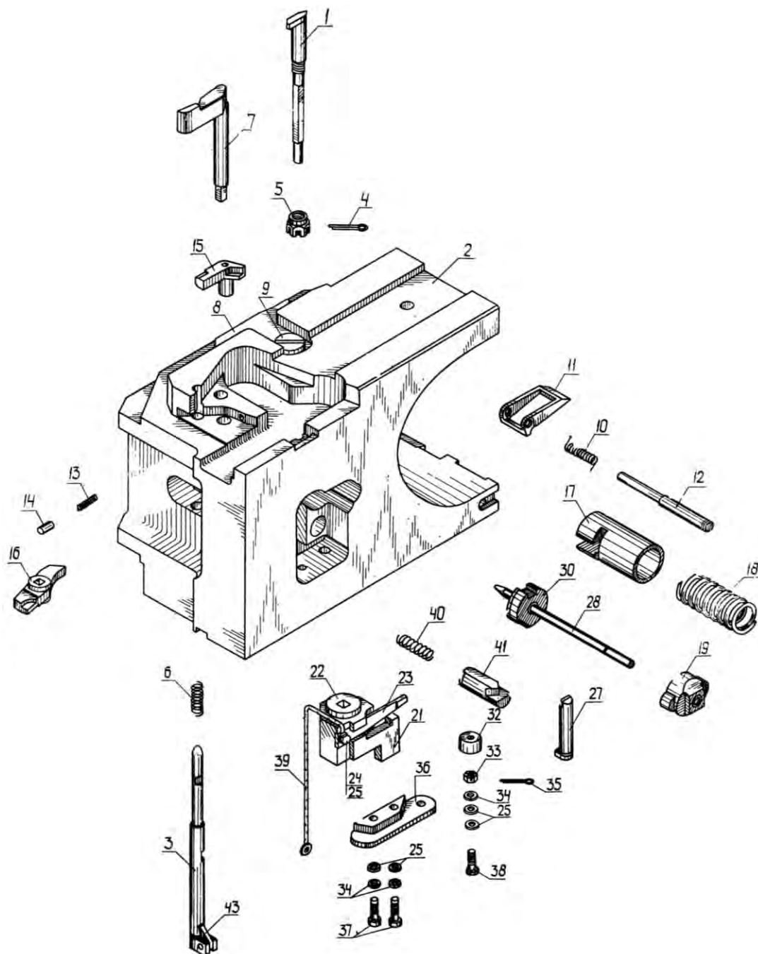
Рис. 5.6. Клины затвора и гальваноударный механизм:
