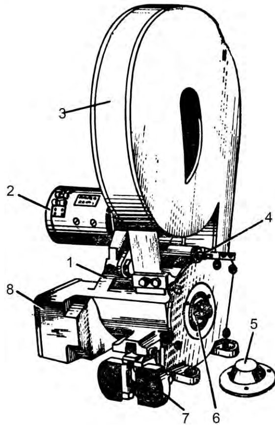
Рис. 5.78. Механизм досылания:
