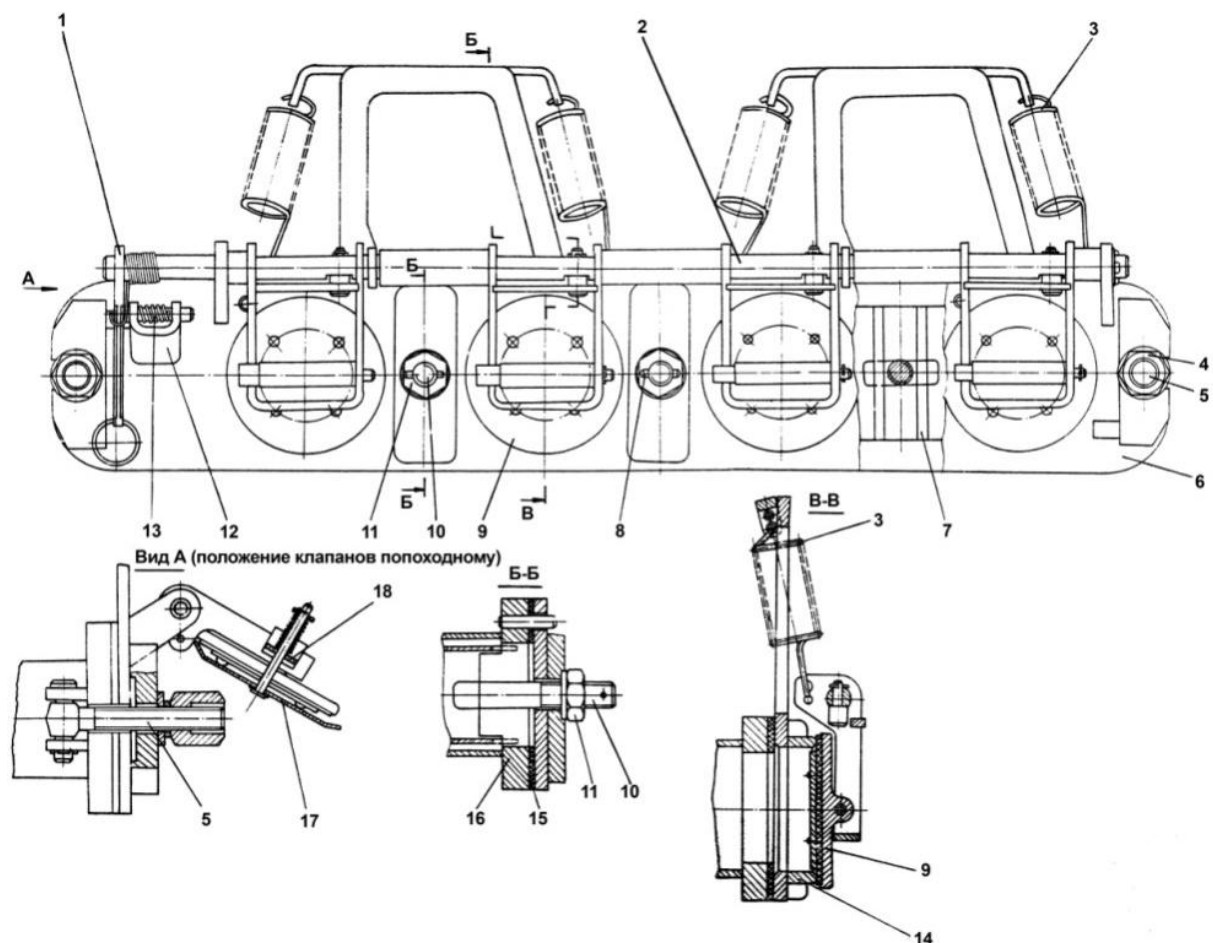
Рис. 16.4. Выпускные клапаны:
