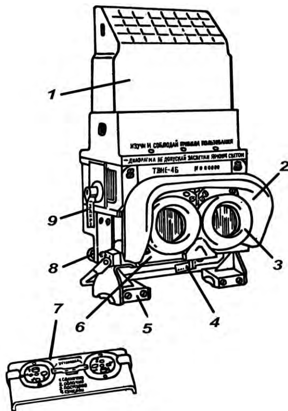
Рис. 6.5. Прибор ТВНЕ-4Б:
