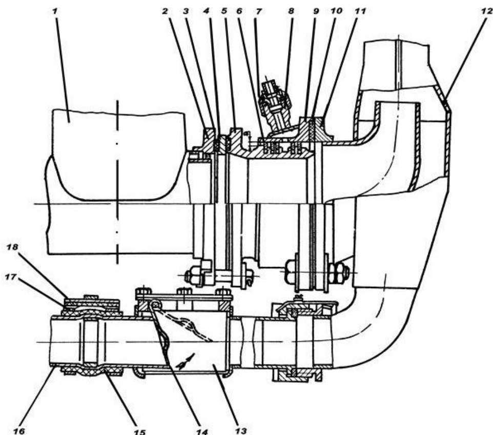
Рис. 8.19. Компенсатор:
