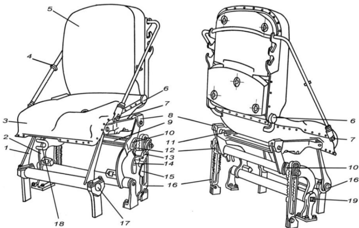
Рис. 4.7. Сиденье механика-водителя:
