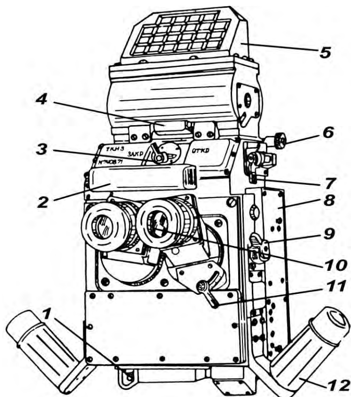
Рис. 6.1. Прибор наблюдения ТКН-3:
