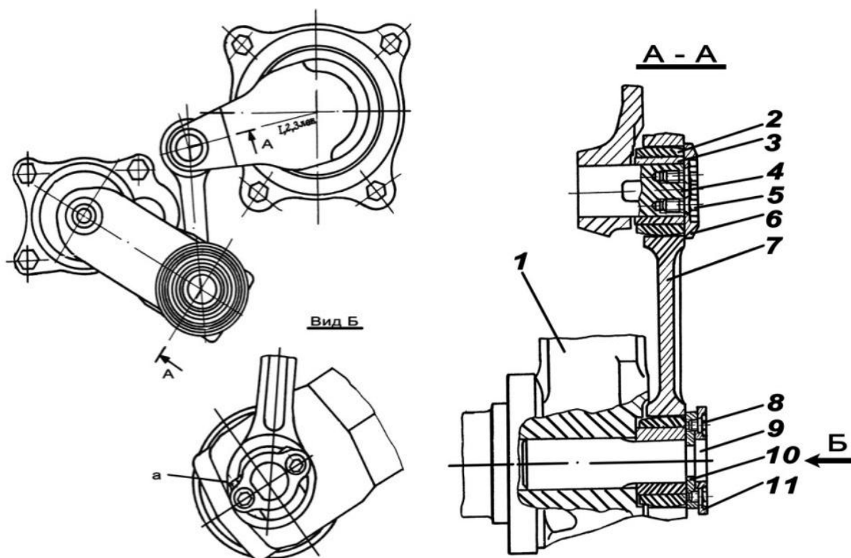
Рис. 10.6. Шарниры гидроамортизатора:
