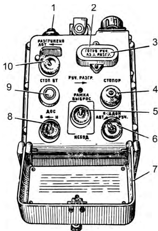
Рис. 5.83. Пульт загрузки автомата зарядания: 1, 4 – кнопки; 2, 3, 9 – сигнальные лампы; 5, 6, 8, 10 – переключатели; 7 – крышка АВАРИЙНО (крышка необходима для предотвращения от случайного нажатия на кнопку СТОПОР и переключатели ПОДДОН, РАМКА ВЫБРОС-ИСХОД, ДОС)
