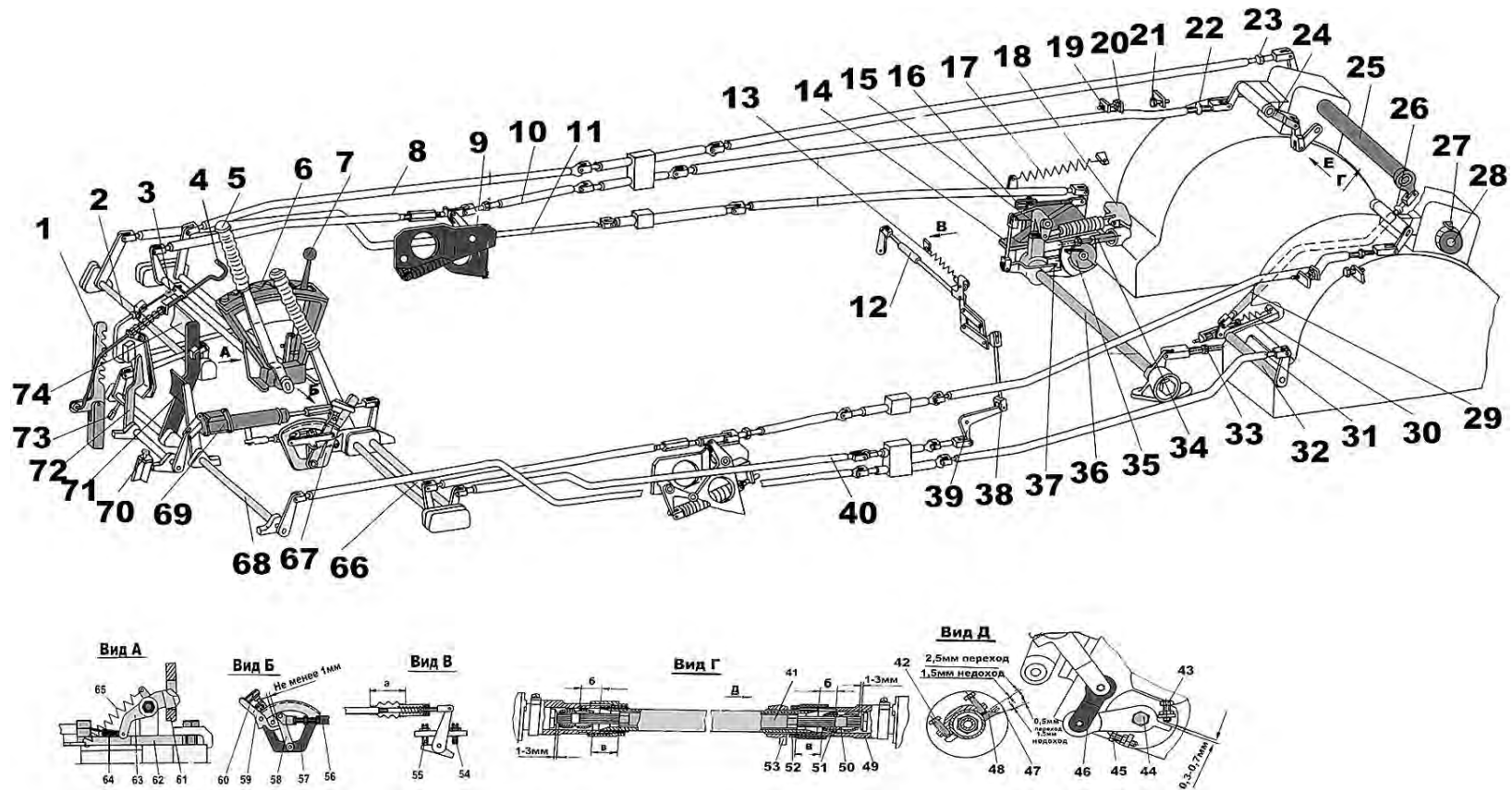
Рис. 8.11. Приводы управления:
