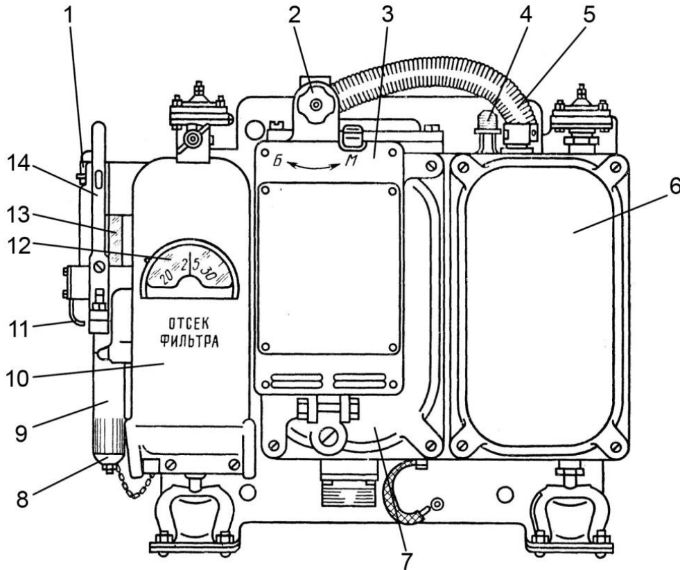
Рис. 13.2. Датчик Б-2:
