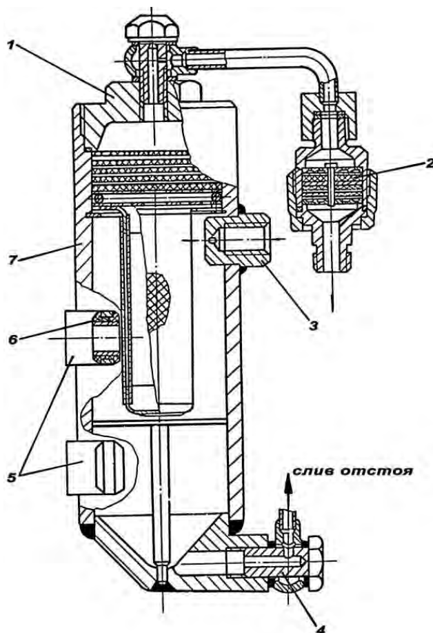
Рис. 8.39. Влагомаслоотделитель:
