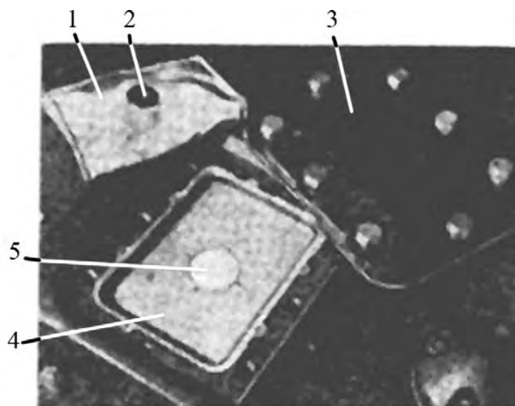
Рис. 5.29. Шахта для головки прицела-дальномера: 1 – мешочек с влагопоглотителем; 2 – смотровое окно; 3 – броневая крышка; 4 – поддон; 5 – пористый фильтр
