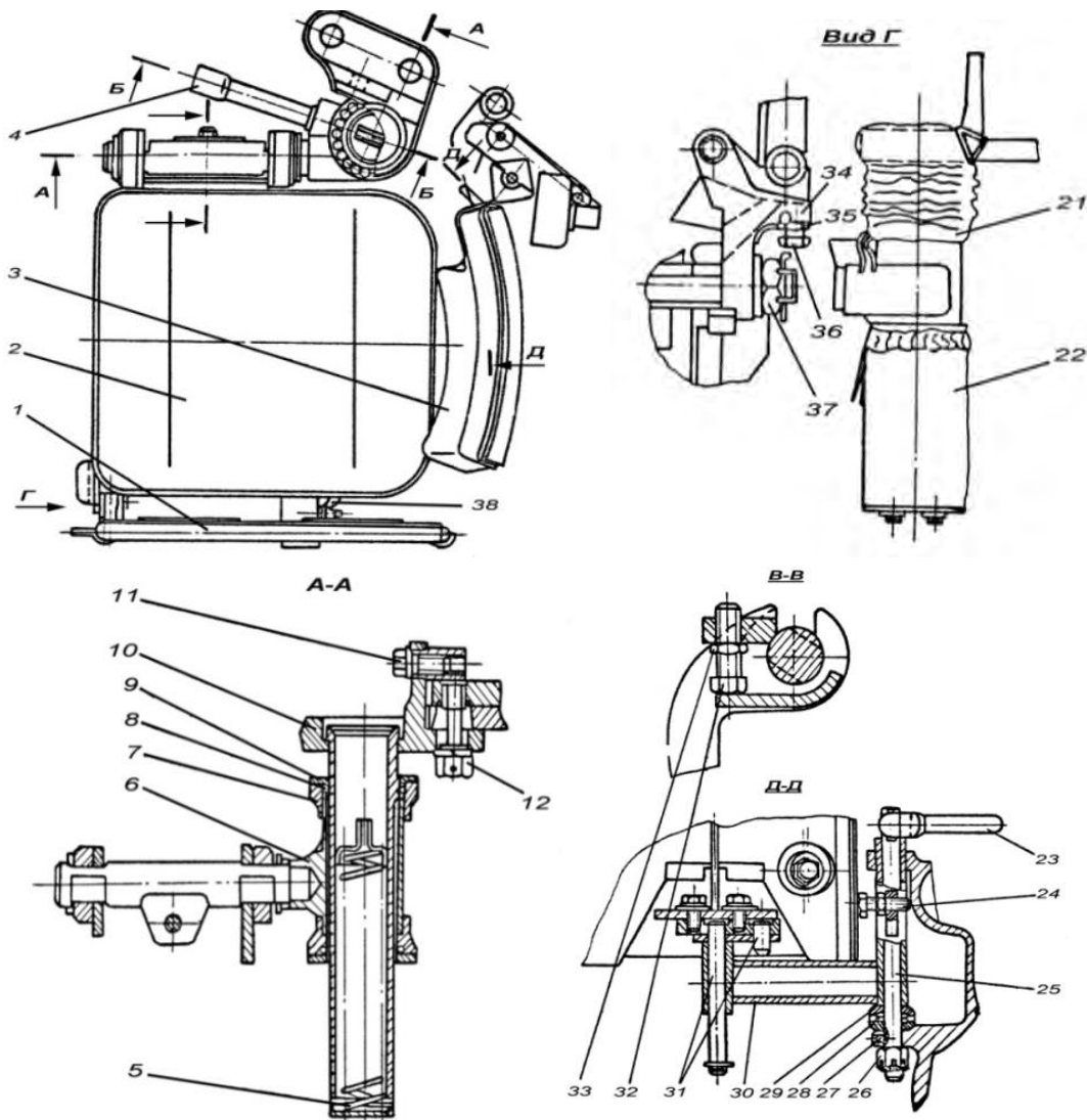
Рис. 4.8. Сиденье командира:
