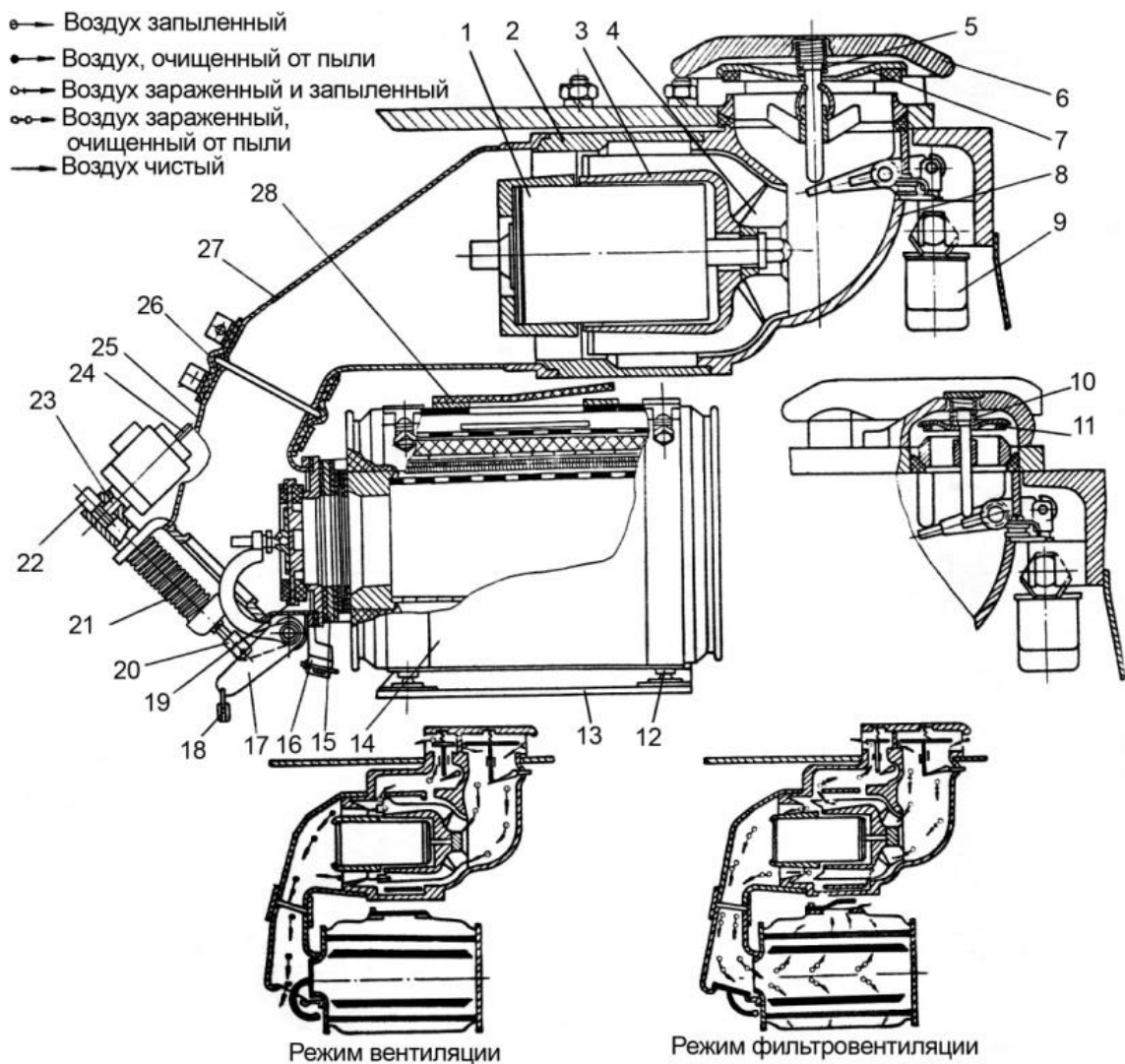
Рис. 13.4. Фильтровентиляционная установка:
