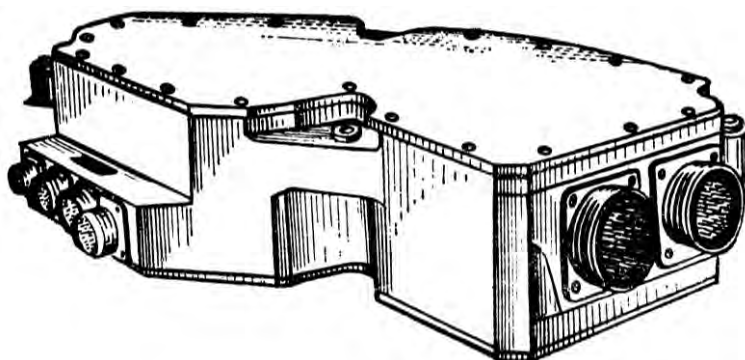
Рис. 5.81. Коробка распределительная автомата заряжания
