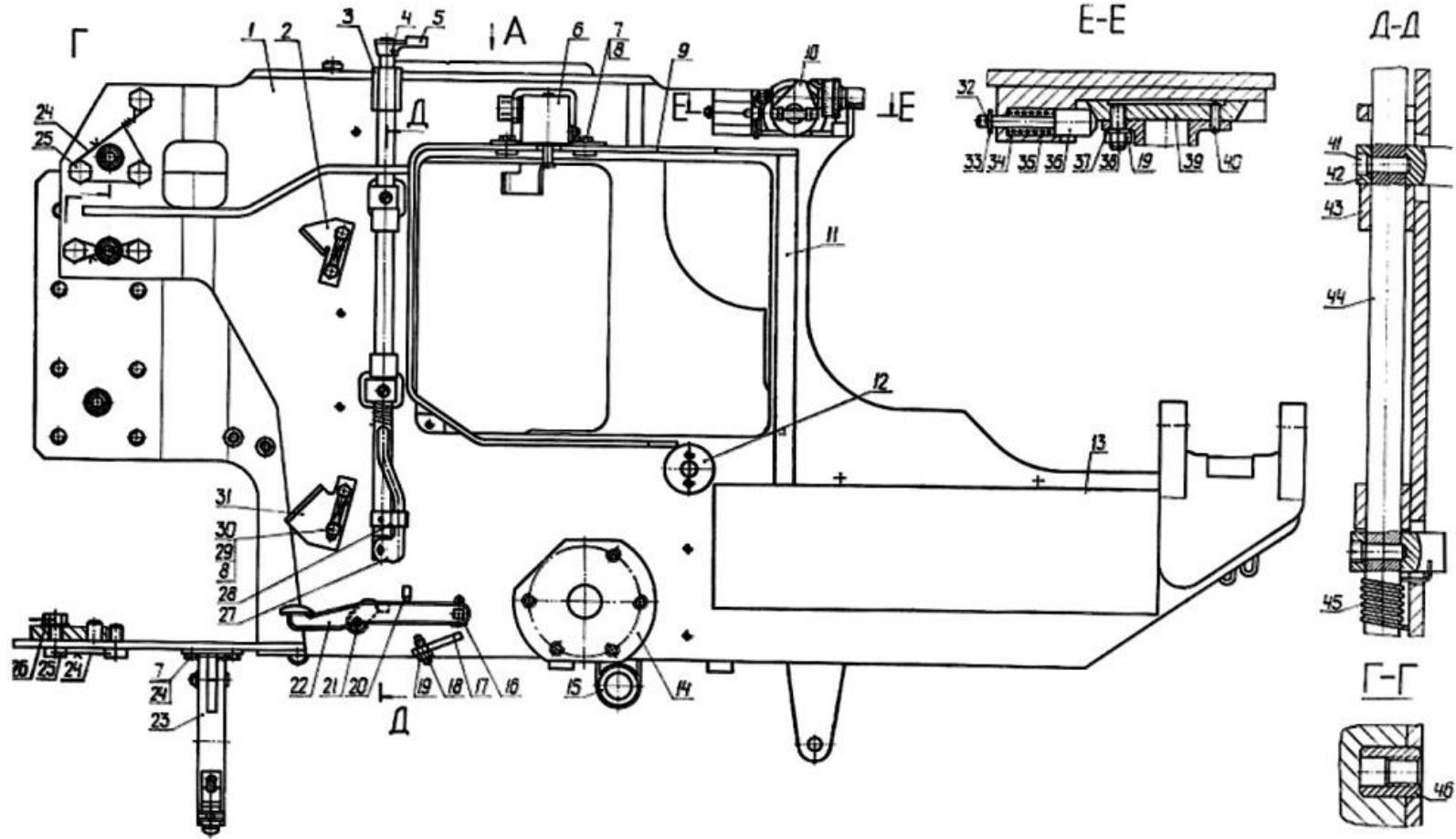
Рис. 5.7. Ограждение (начало)
