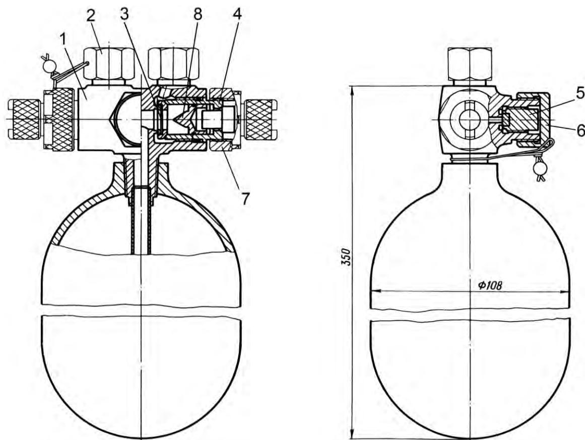
Рис. 14.1. Баллон ППО: 1 – корпус; 2 – заглушка; 3 – мембрана; 4 – пробка; 5 – штуцер; 6 – заглушка; 7 – гайка; 8 – пробойник
