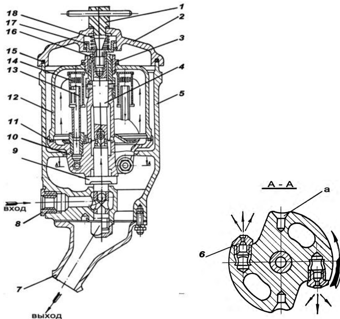
Рис. 8.24. Центробежный маслоочиститель:
