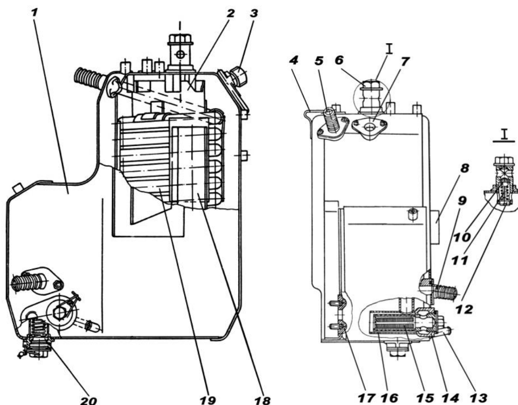
Рис. 8.20. Основной масляный бак:
