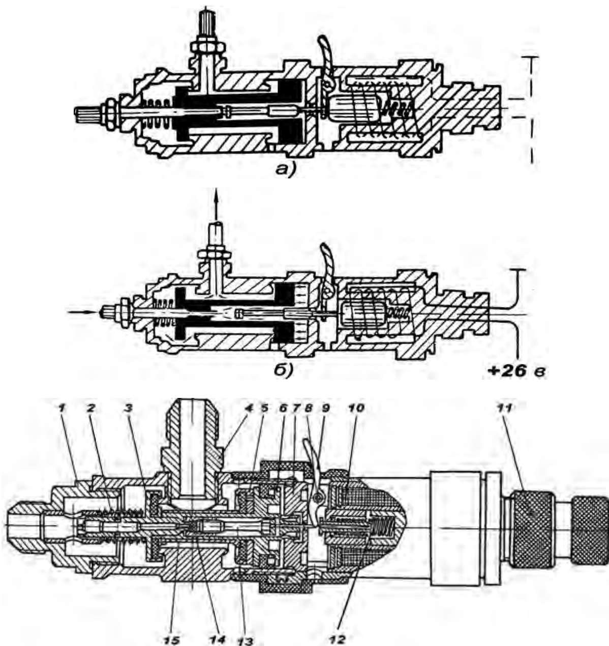
Рис. 8.44. Электропневмоклапан ЭК-48:
