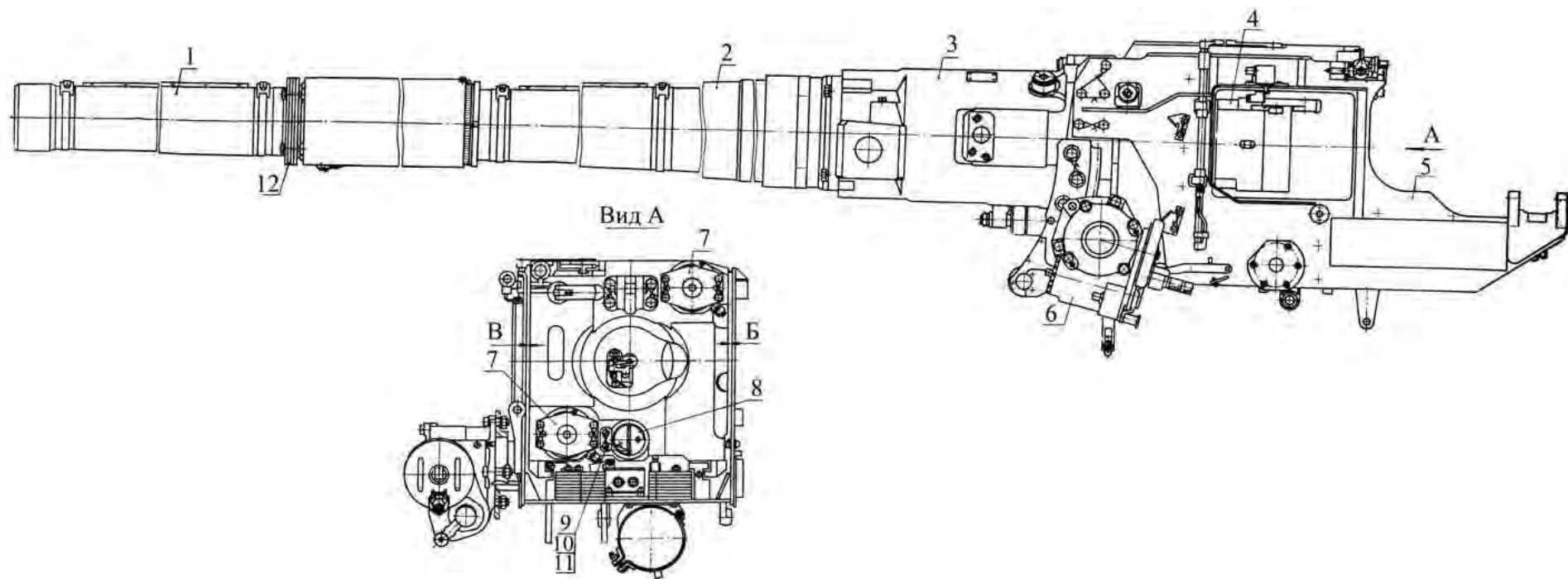
Рис. 5.3. Танковая пушка 2А46М:
