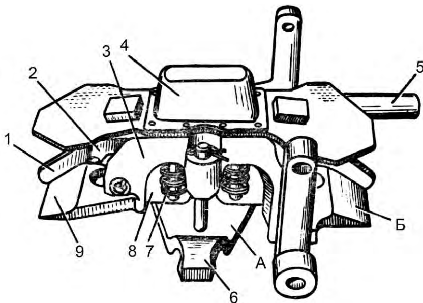
Рис. 5.73. Захват:
