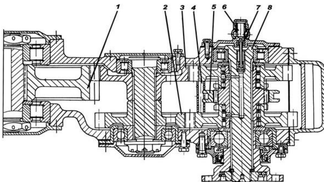
Рис. 9.6. Редуктор привода вентилятора:
