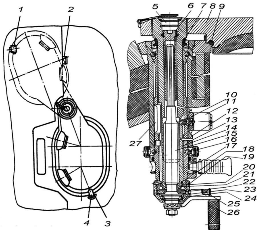
Рис. 4.3. Люк механика-водителя:
