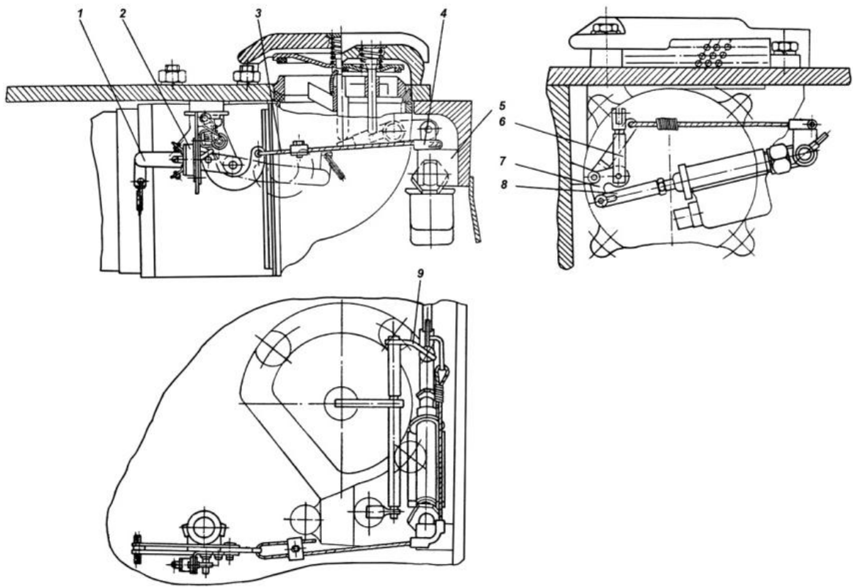
Рис. 13.5. Приводы к клапанам нагнетателя: 1 – рукоятка с кольцом; 2 – переключатель; 3 – трос; 4 – направляющая трубка; 5 – кронштейн крепления бустера; 6 – тяга; 7 – трехплечий рычаг; 8 – регулировочная вилка; 9 – рычаг нагнетателя
