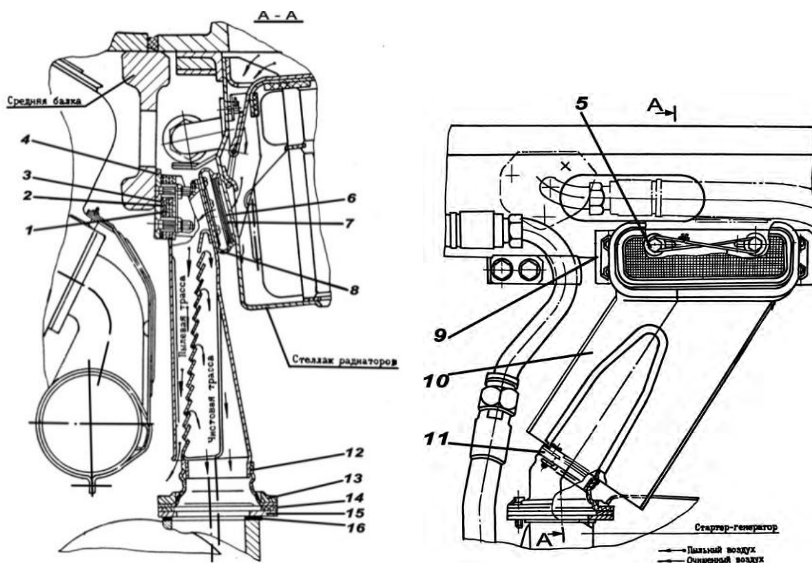
Рис. 11.1. Установка инерционной решетки:
