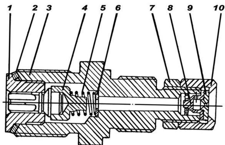
Рис. 8.35. Форсунка подогревателя:
