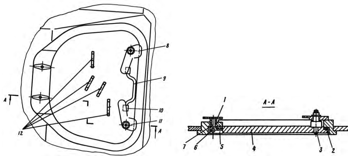
Рис. 4.4. Люк запасного выхода:
