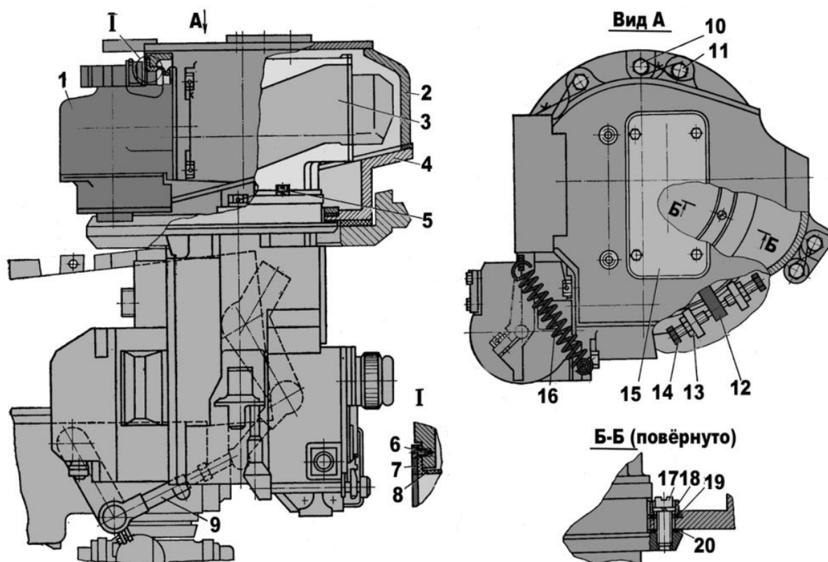
Рис. 5.55. Установка прицела-прибора наведения 1К13:
