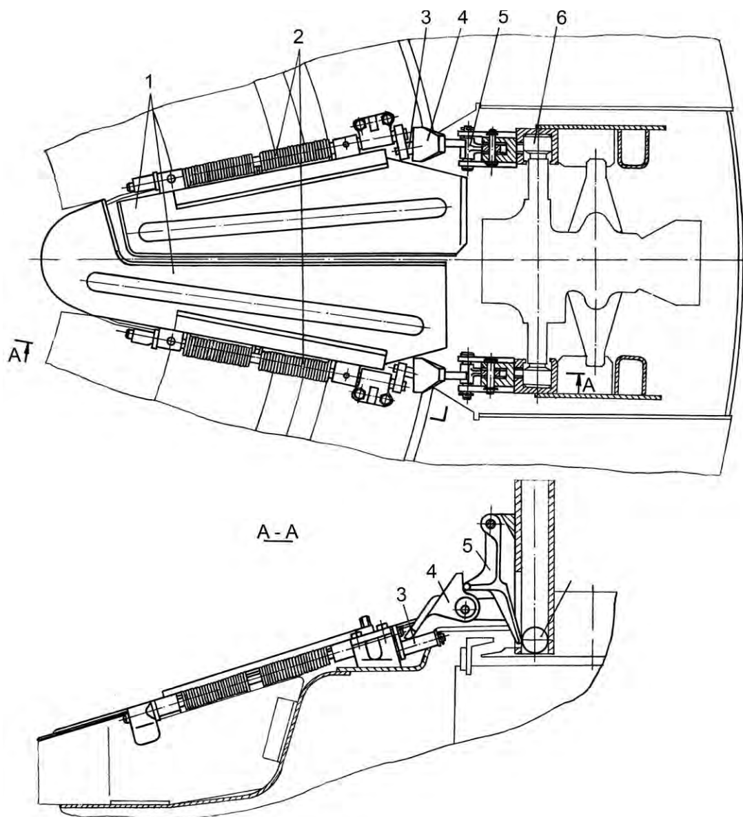
Рис. 5.70. Механизм закрывания окна выдачи ВТ: 1 – створки; 2 – пружины; 3 – оси; 4, 5 – рычаги; 6 – ролик захвата МПК
