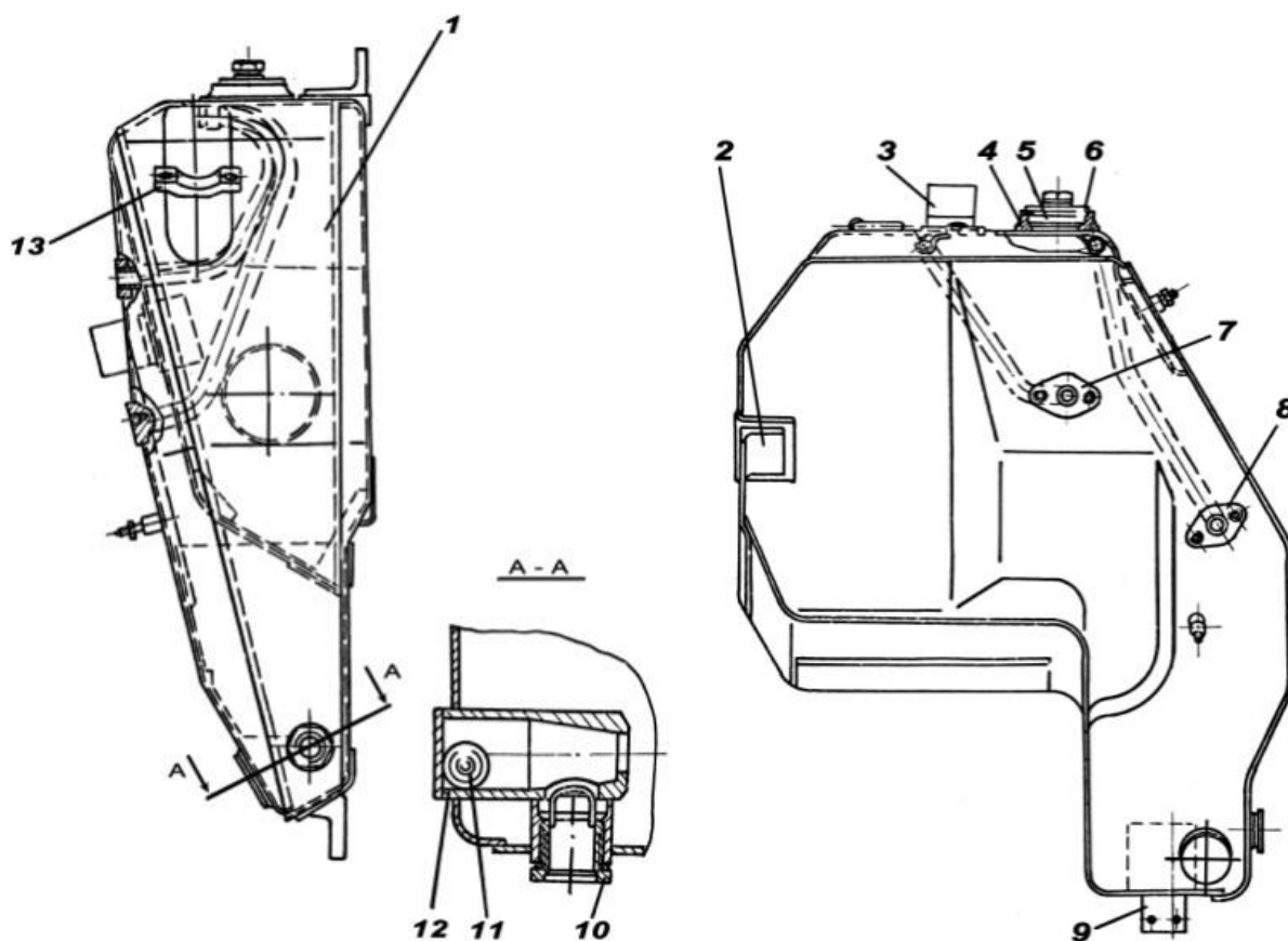
Рис. 8.21. Дополнительный масляный бак:
