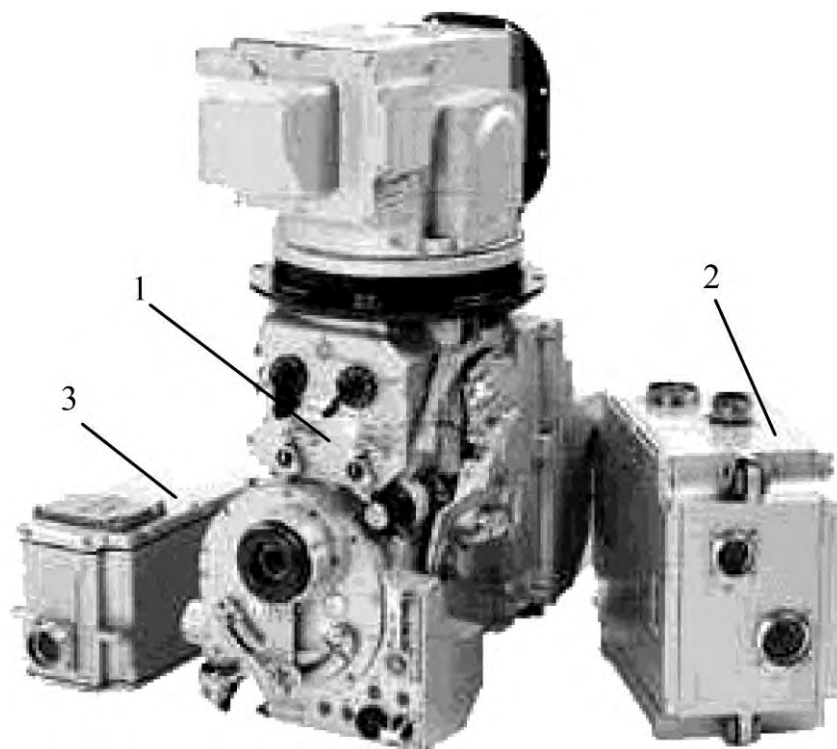
Рис. 5.54. Прицел-прибор наведения 1К13: 1 – блок оптико-механический; 2 – электронный блок; 3 – блок 1К75
