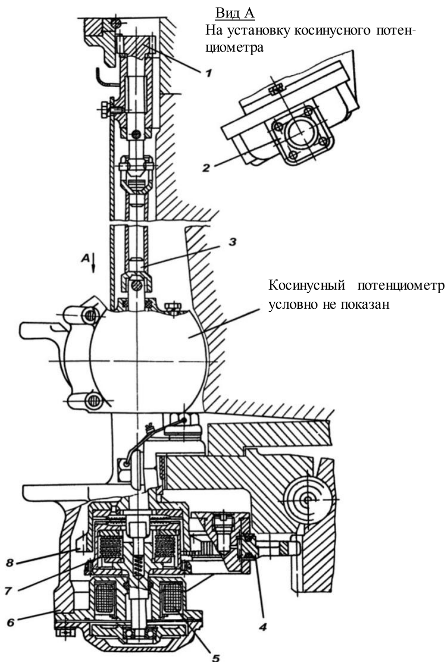
Рис. 4.14. Привод командирской башенки: 1 – ведомый валик; 2 – косинусный потенциометр; 3 – карданная передача; 4, 8 – шестерни; 5 – электромагнит; 6 – корпус; 7 – фрикцион
