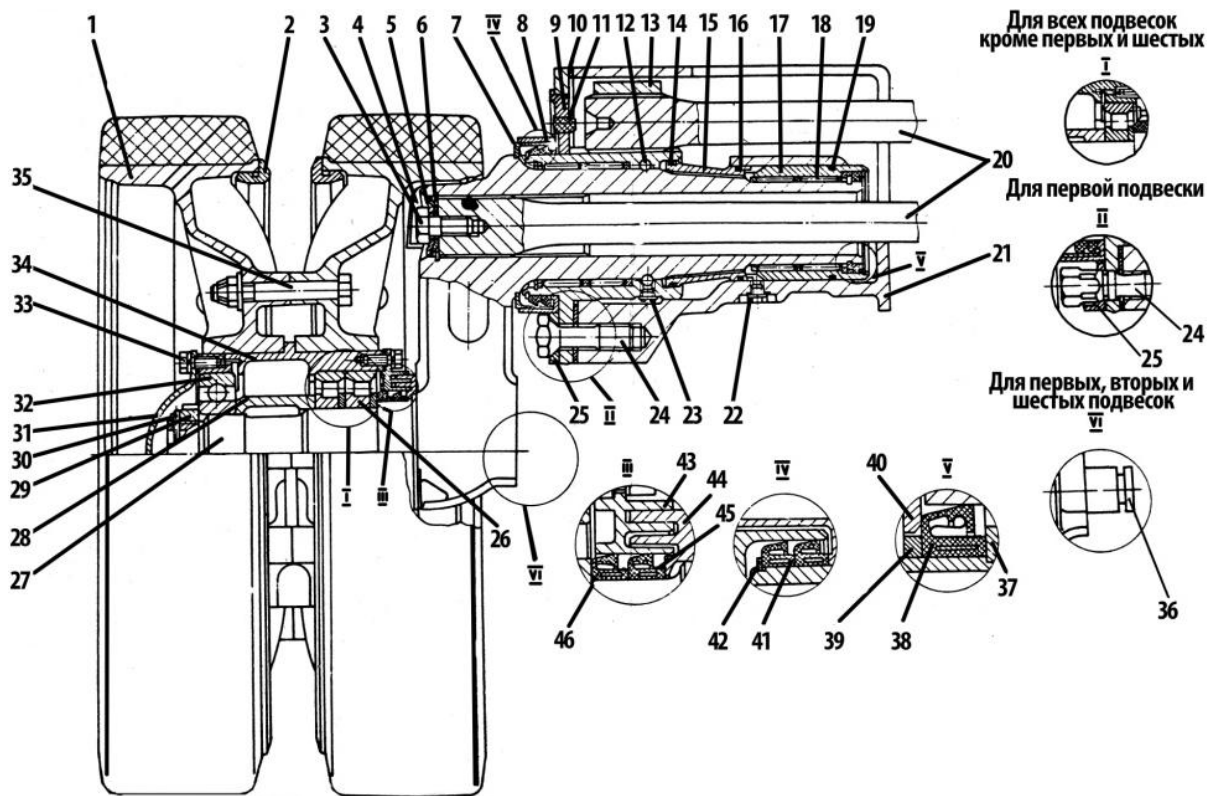
Рис. 10.2. Опорный каток и элементы подвески:
