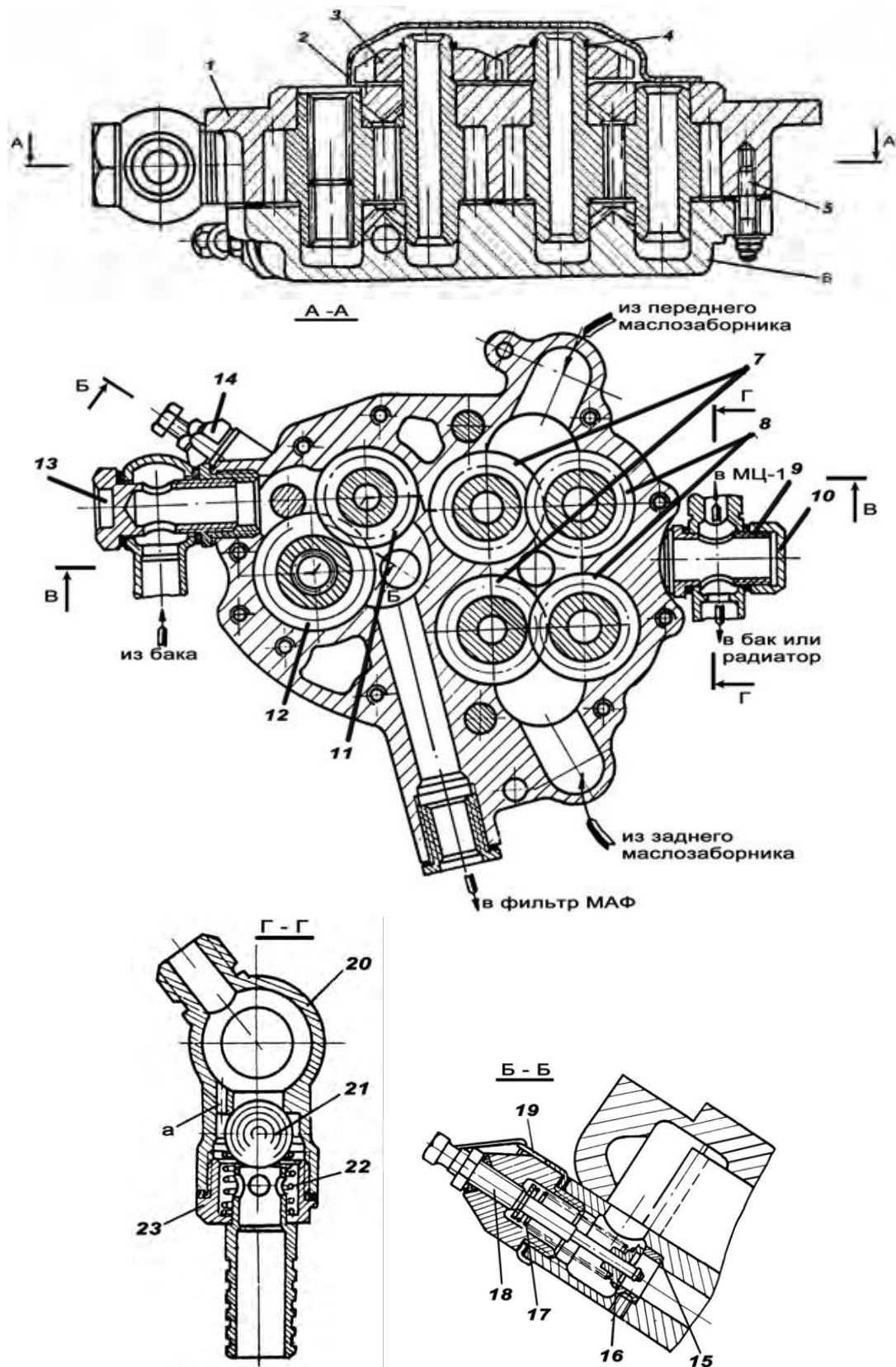
Рис. 8.22. Масляный насос:
