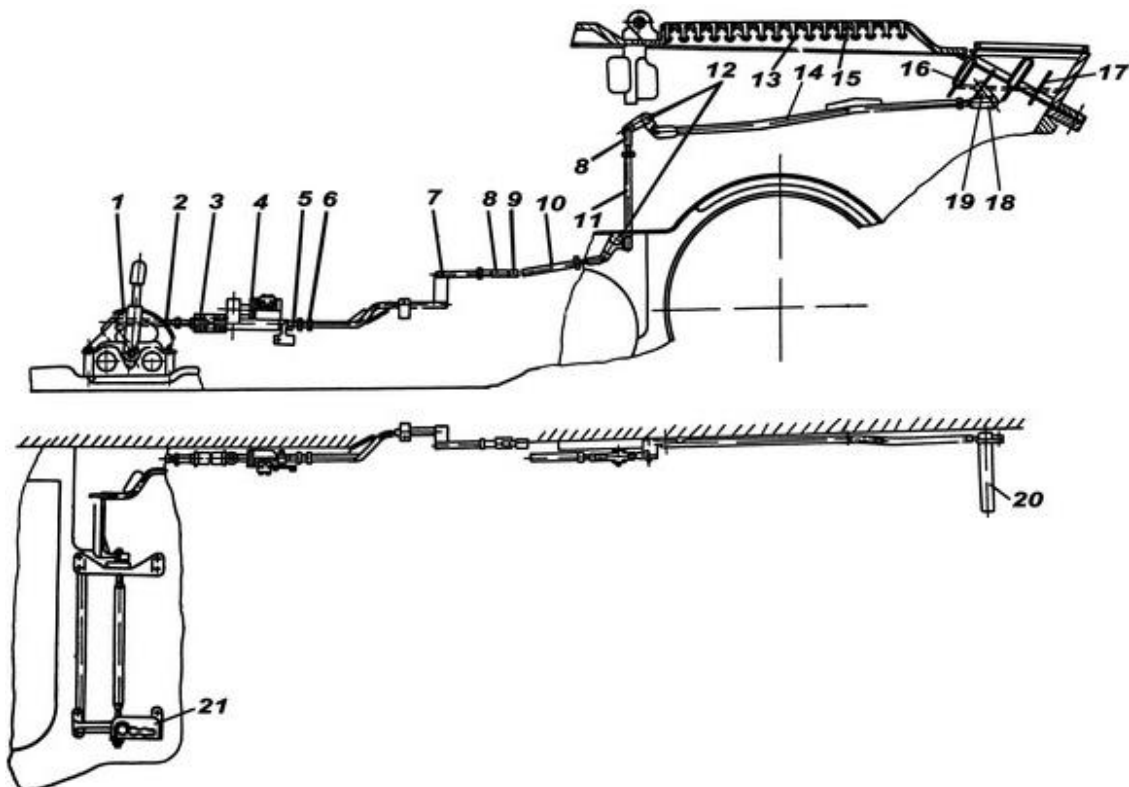
Рис. 8.32. Привод жалюзи:
