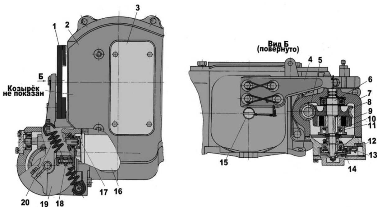
Рис. 5.57. Привод электромеханический защитной крышки:
