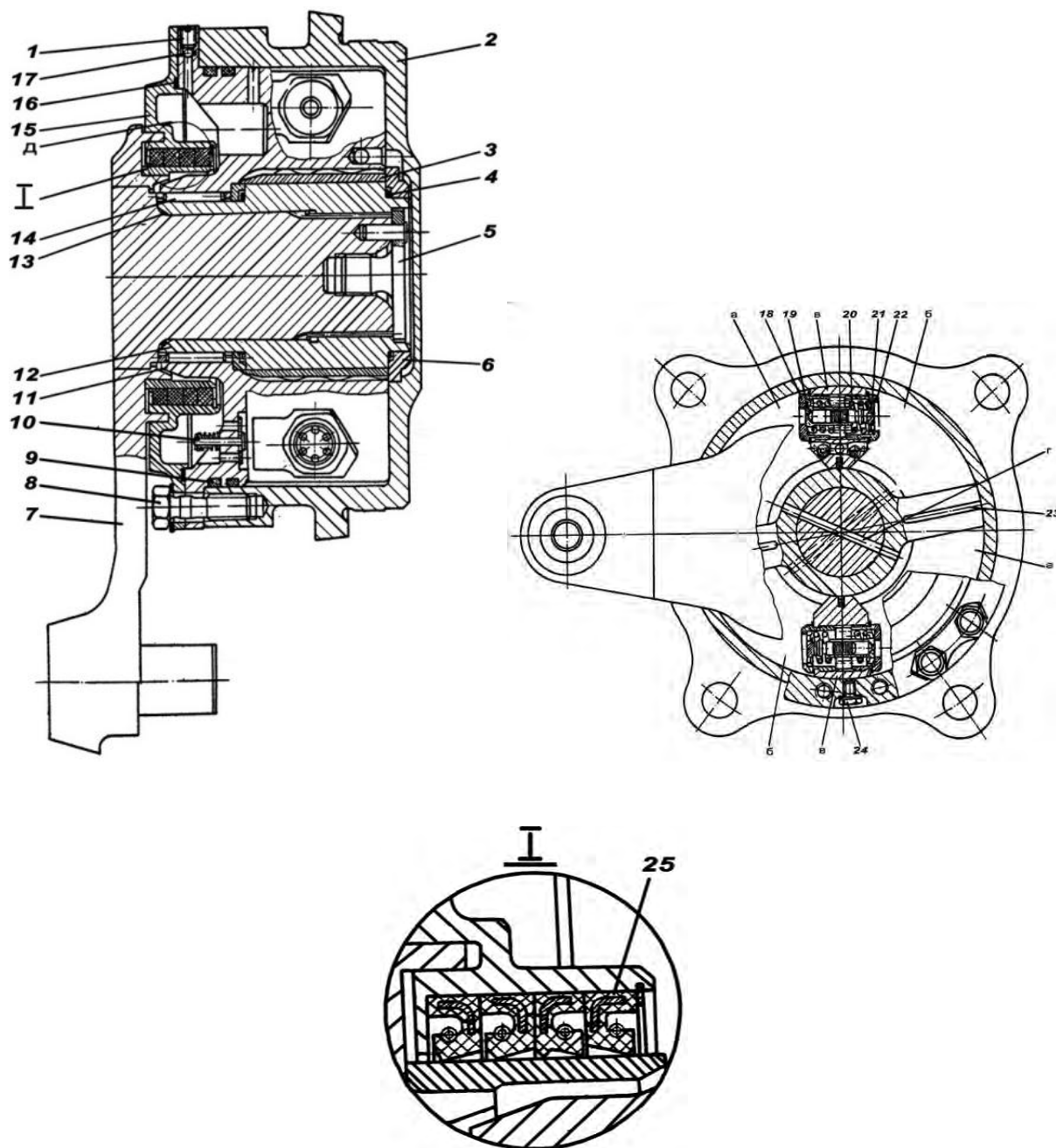
Рис. 10.5. Устройство гидроамортизатора:
