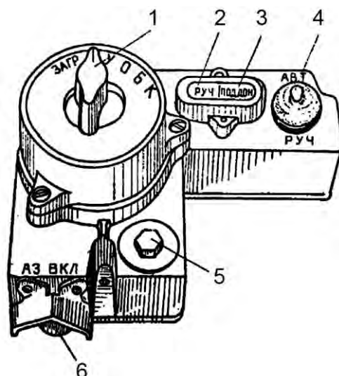
Рис. 5.82. Пульт управления автомата зарядки:
