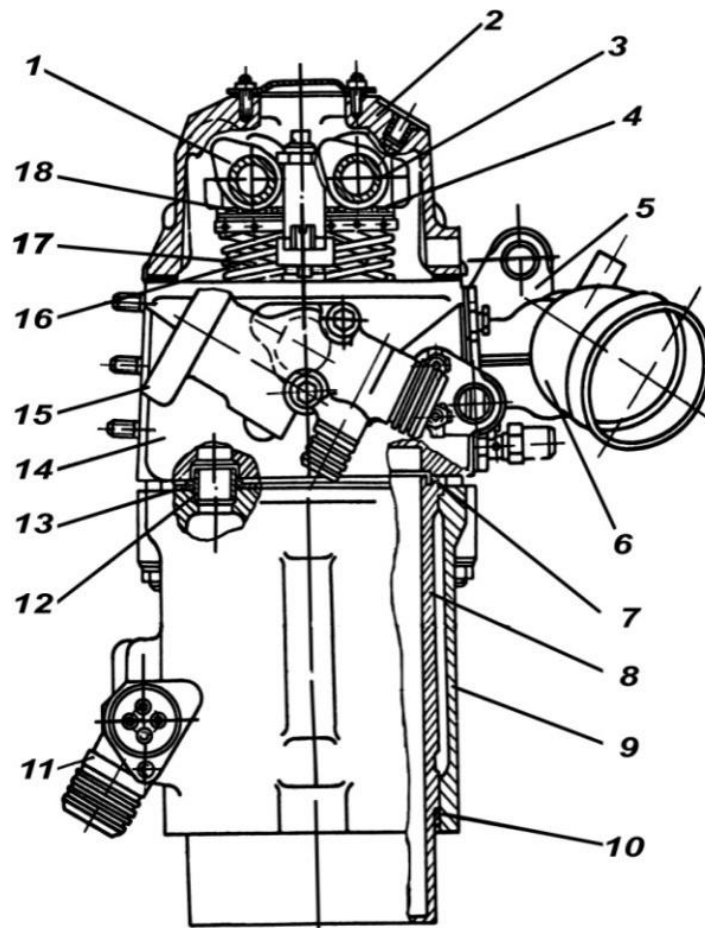
Рис. 8.1. Блок цилиндров:
