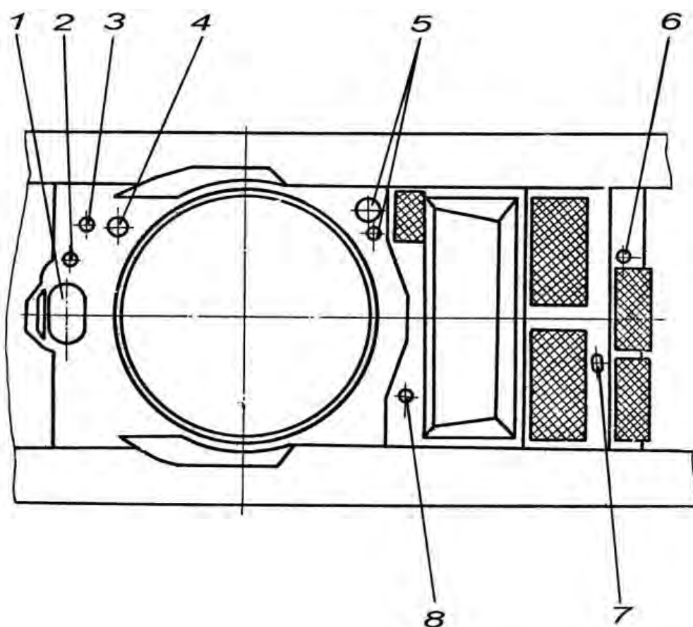
Рис. 4.1. Расположение люков на крыше:
