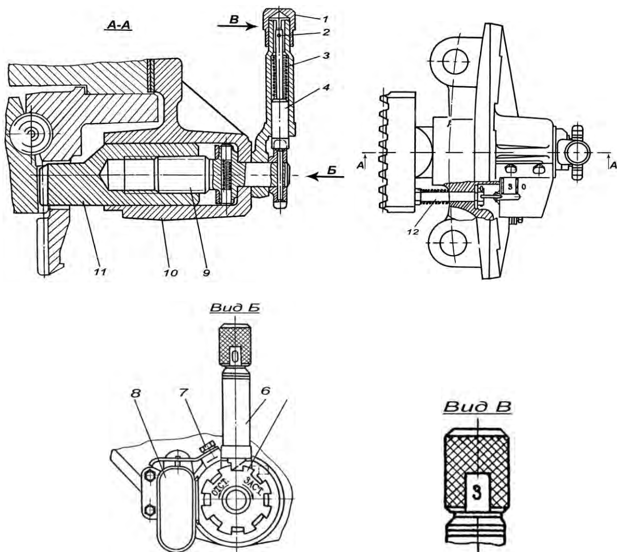
Рис. 4.11. Стопор башни:
