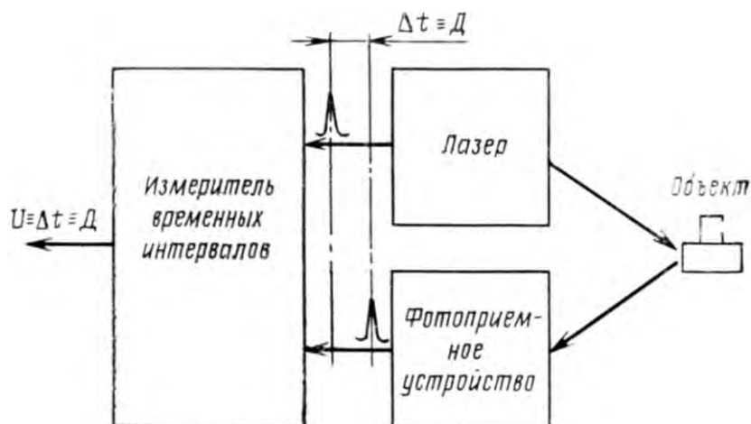
Рис. 5.32. Структурная схема дальномера
