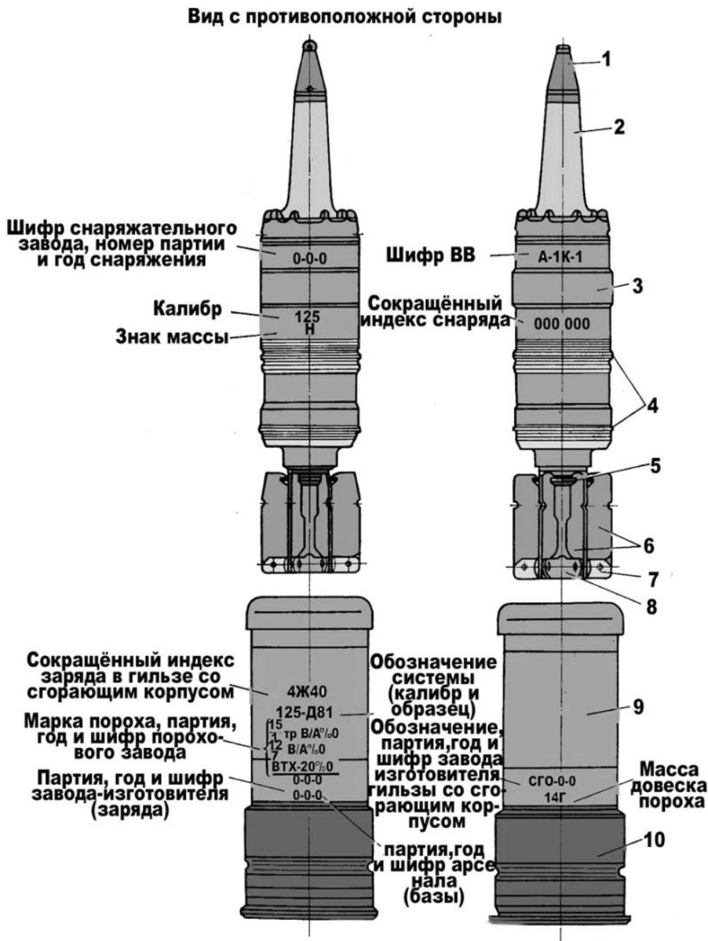
Рис. 5.23. Выстрел с кумулятивным снарядом:
