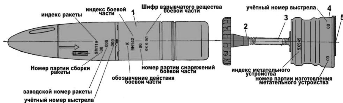
Рис. 5.26. Выстрел 3УБК14 с управляемой ракетой 9М119: 1 – управляемая ракета 9М119; 2 – корпус; 3 – досылатель; 4 – поддон; 5 – индукторная втулка
