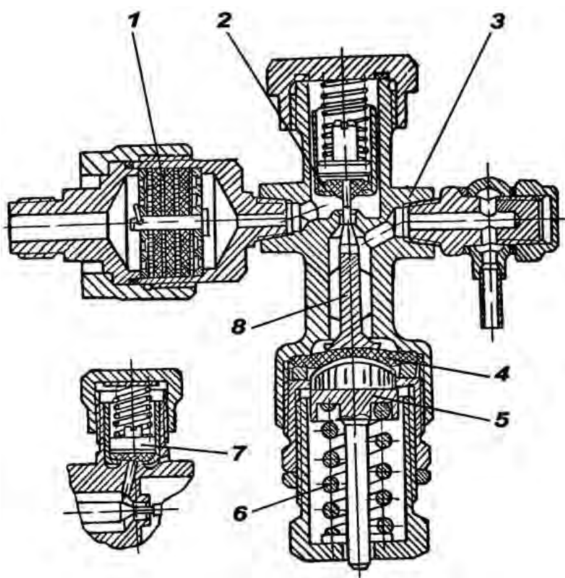
Рис. 8.43. Редуктор ИЛ611-150-70К:
