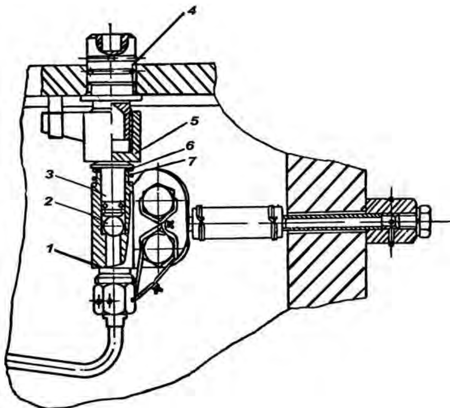
Рис. 8.41. Клапан слива отстоя из влагомаслоотделителя: 1 – корпус; 2 – шарик; 3 – толкатель; 4 – упорный винт; 5 – гайка; 6 – уплотнение; 7 – пружина
