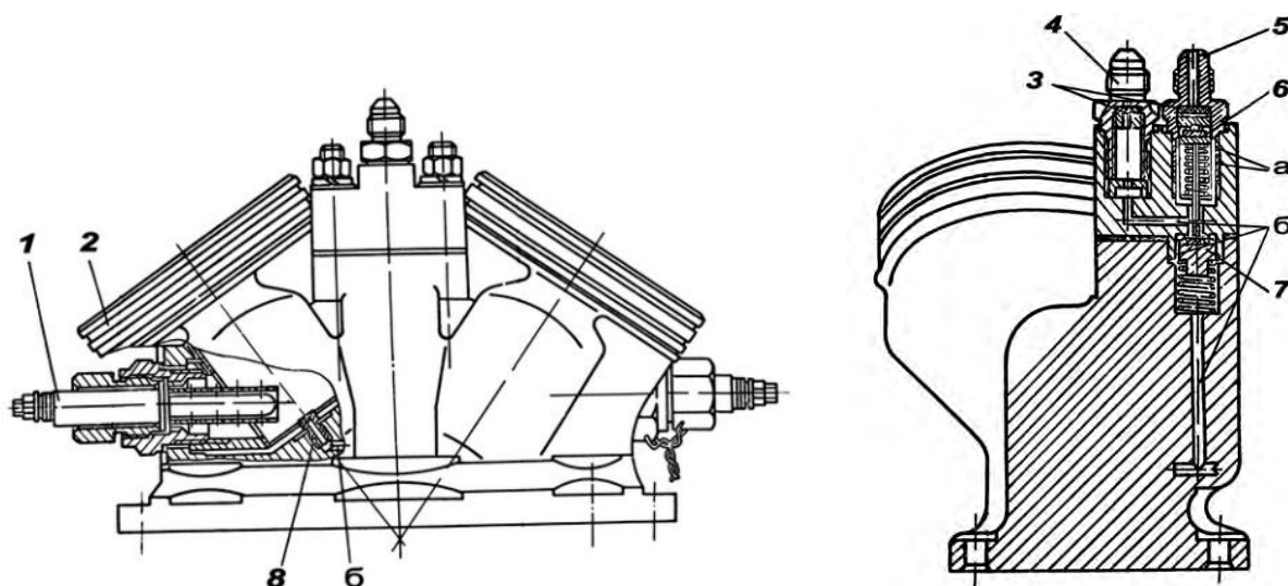
Рис. 8.45. Подогреватель впускного воздуха:
