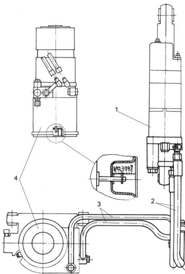
Рис. 5.38. Гидропривод:
