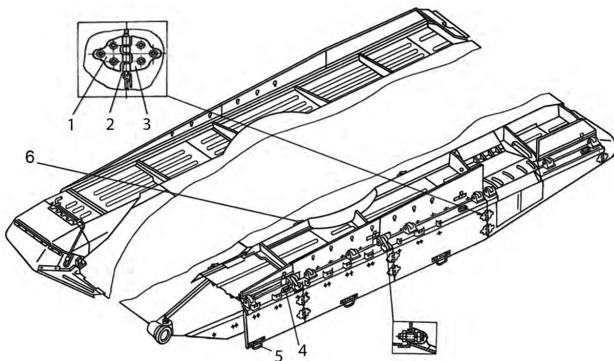
Рис. 3.3. Щитки бортовые: 1, 3 – петли; 2 – ось; 4, 5, 6 – скоба
