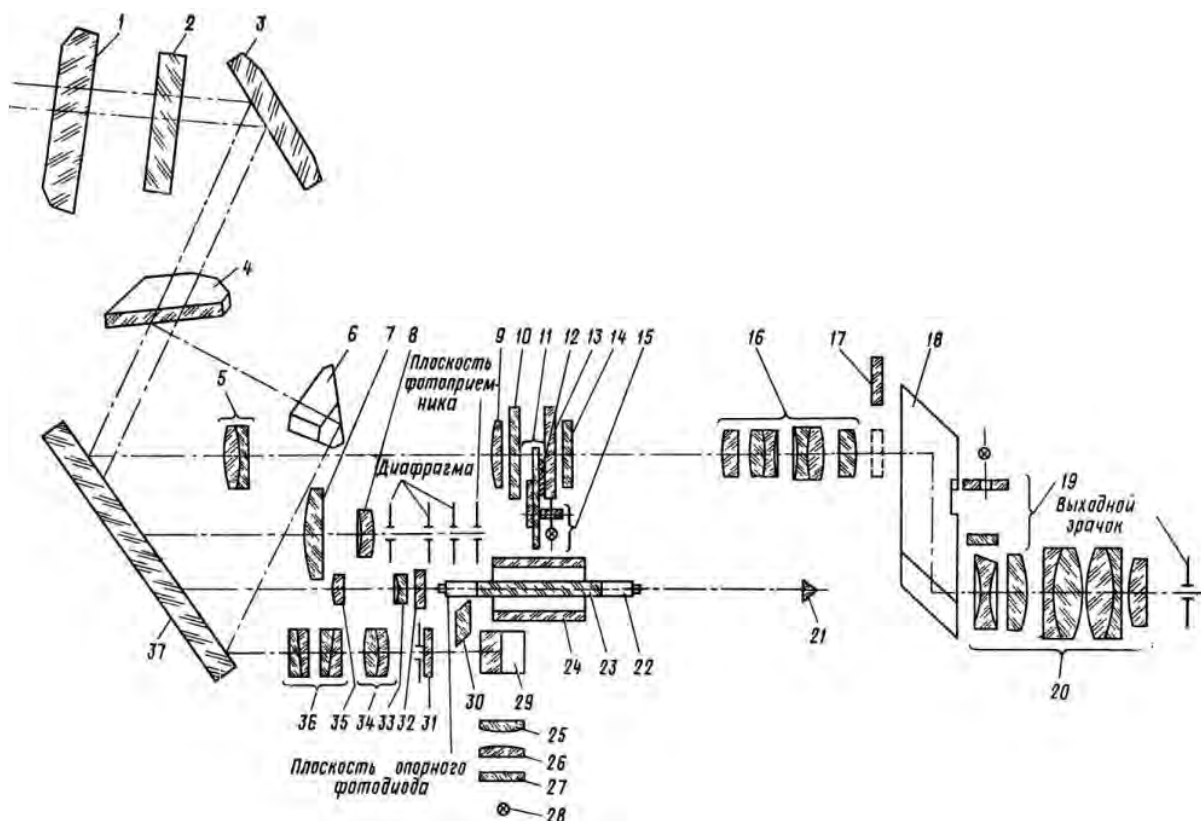
Рис. 5.35. Оптическая схема изделия 1А40-1:
