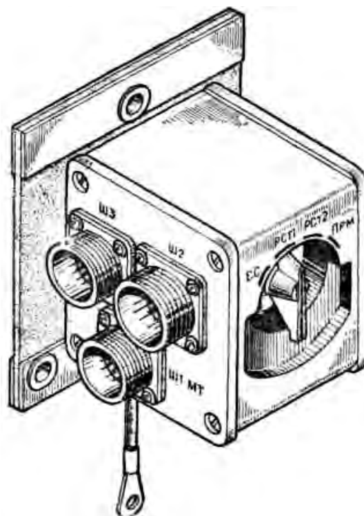
Рис. 12.4. Прибор БВ35
