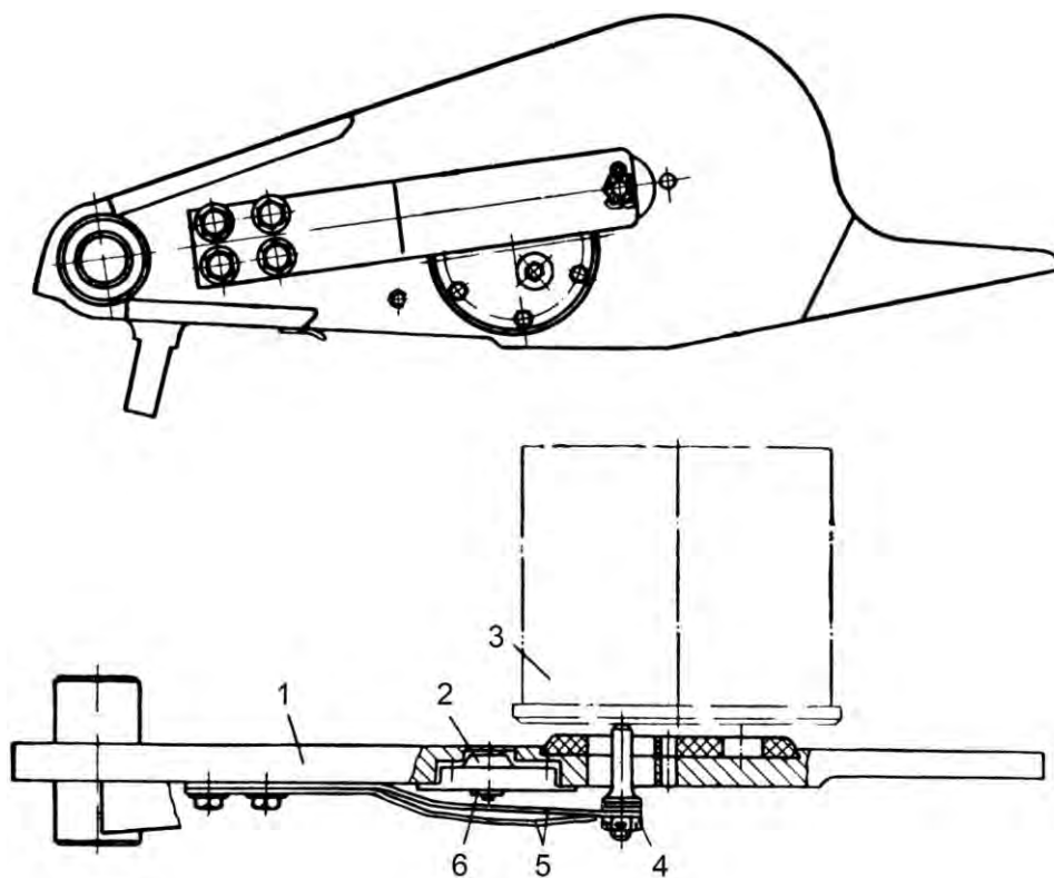
Рис. 5.77. Упор поддона: 1 – пластина; 2 – электрическая кнопка; 3 – поддон; 4 – винт; 5 – пластинчатые пружины; 6 – контакт
