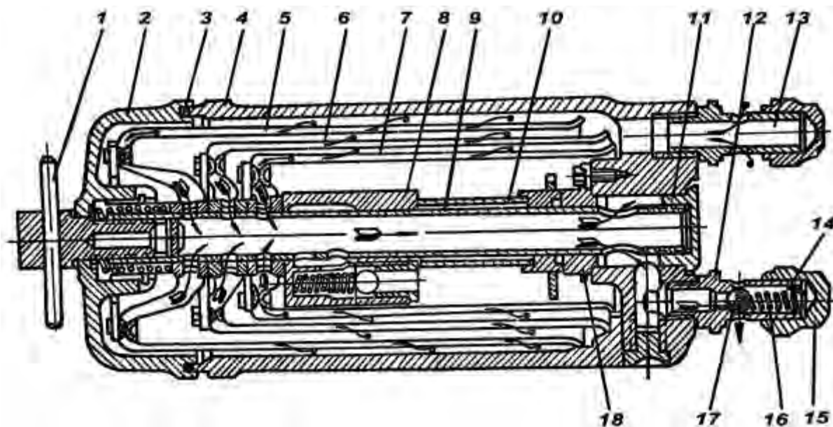
Рис. 8.23. Масляный фильтр:
