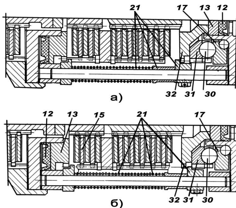
Рис. 9.8. Коробка передач (окончание):
