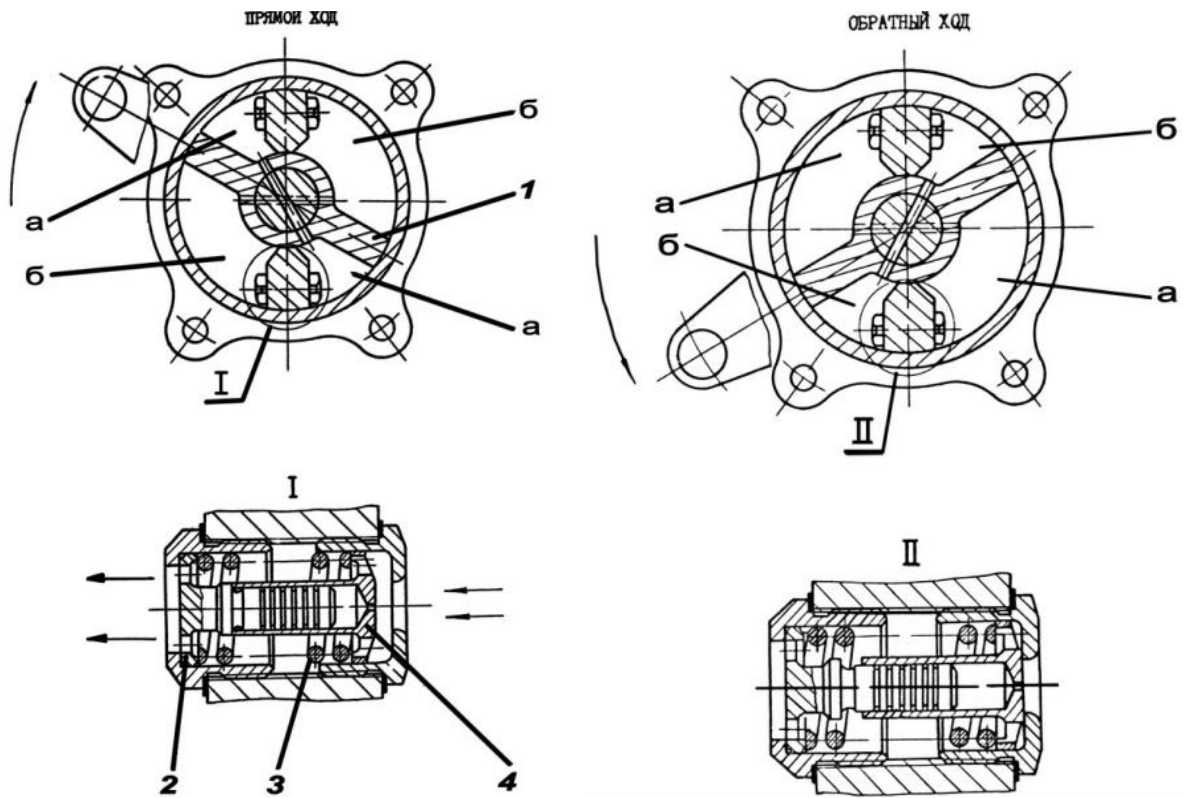
Рис. 10.7. Работа гидроамортизатора: 1 – лопасть; 2 – плунжер; 3 – пружина; 4 – клапан; а, б – рабочие камеры
