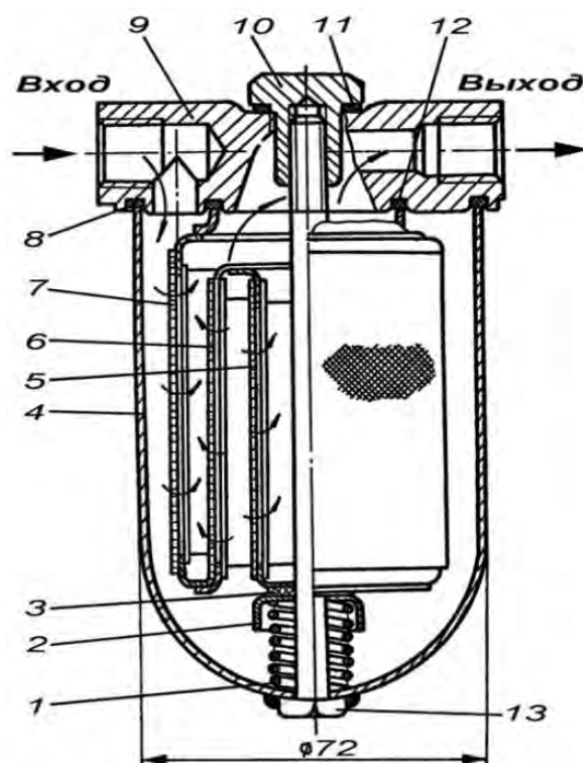
Рис. 8.7. Топливный фильтр грубой очистки:
