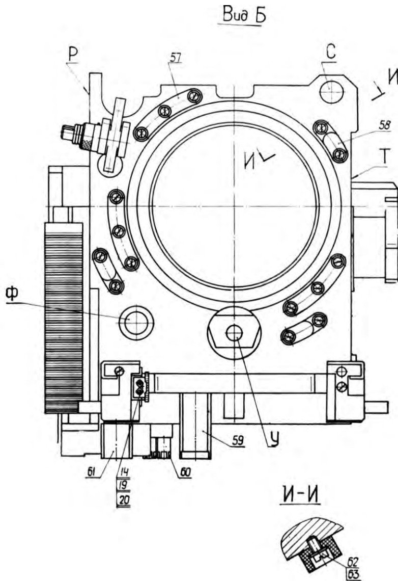
Рис. 5.11. Люлька (окончание):
