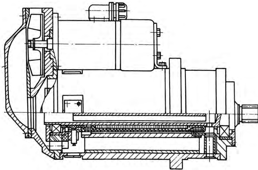
Рис. 5.42. Исполнительный электродвигатель ЭДМ-16У
