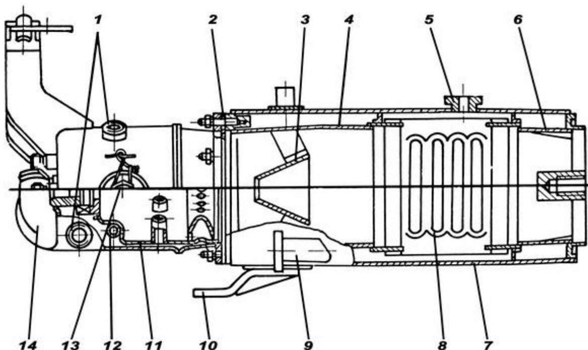
Рис. 8.34. Котел подогревателя:
