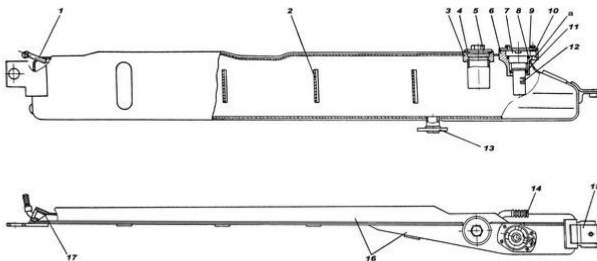
Рис. 8.28. Расширительный бачок:
