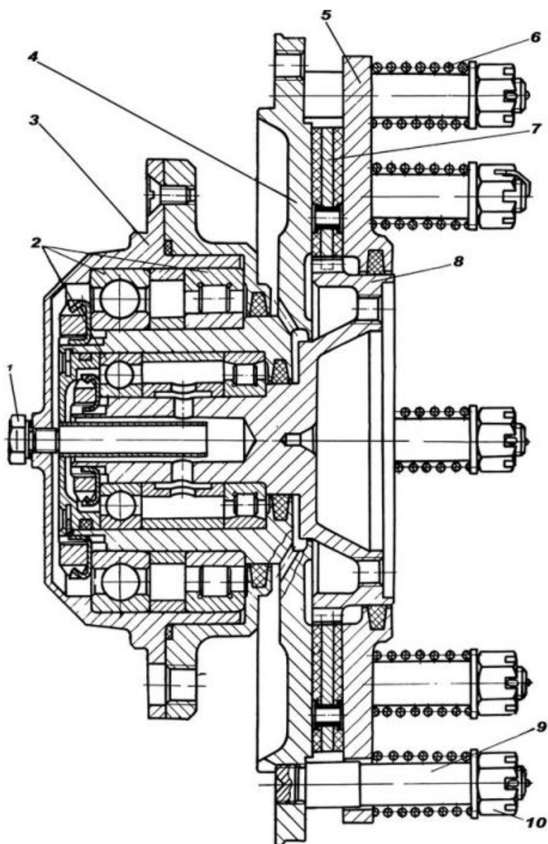
Рис. 9.7. Фрикцион вентилятора:
