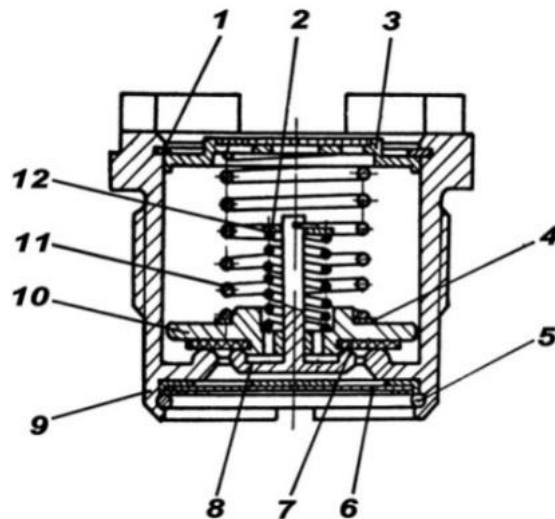
Рис. 8.30. Паровоздушный клапан:
