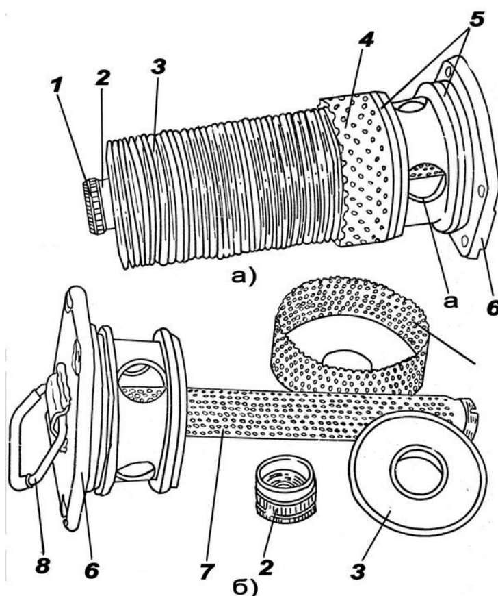
Рис. 9.20. Фильтрующий элемент: 1 – стопорное кольцо; 2 – гайка; 3 – фильтрующие секции; 4 – защитная сетка; 5 – резиновые кольца; 6 – крышка; 7 – стержень; 8 – ручка; а – окно а) элемент в сборе; б) детали элемента
