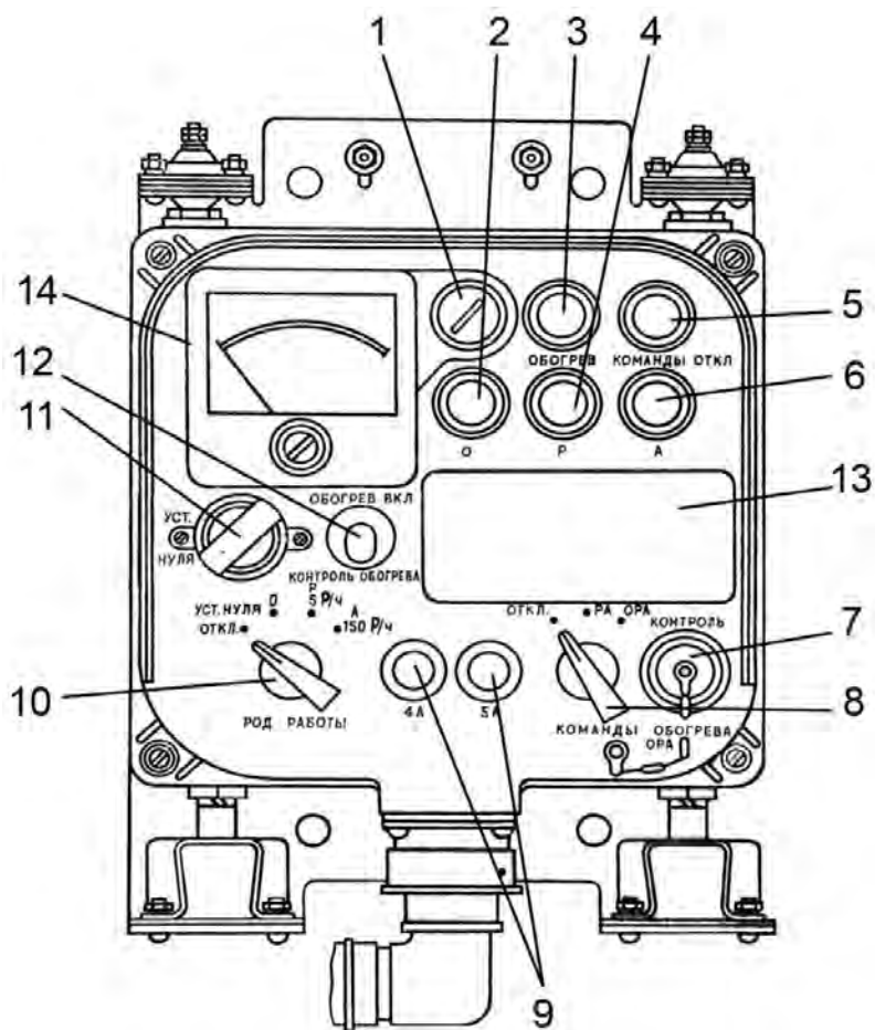
Рис. 13.1. Измерительный пульт Б-1:
