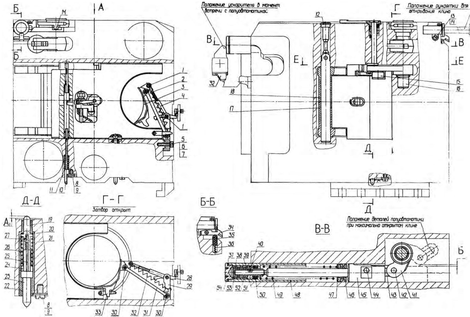
Рис. 5.4. Затвор (начало)
