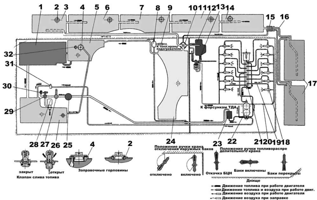
Рис. 8.14. Система питания топливом. Схема гидравлическая принципиальная: 1 – правый носовой бак; 2, 4 – заправочные горловины; 3, 6, 7, 11, 14 – наружные баки; 5 – передний бак-стеллаж; 8 – топливный насос подогревателя; 9 – топливный фильтр подогревателя; 10 – кран отключения наружных баков; 12 – расширительный бачок; 13 – поплавковый клапан; 15 – переходник для подключения бочек; 16 – оборудование для подключения бочек; 17 – бочки; 18 – форсунка; 19 – трубопровод высокого давления; 20 – трубопровод объединенного слива топлива из форсунок; 21 – топливный насос НК-12М; 22 – топливный фильтр тонкой очистки; 23 – топливоподкачивающий насос НТП-46; 24 – средний бак-стеллаж; 25 – топливный фильтр грубой очистки; 26 – левый носовой бак; 27 – ручной топливоподкачивающий насос; 28 – топливоподкачивающий насос БЦН-1; 29 – топливораспределительный кран; 30 – сливной штуцер; 31 – клапан выпуска воздуха; 32, 36 – шланги; 33 – штуцер; 34 – шланг слива отстоя; 35 – тройник; 37 – измеритель топлива
