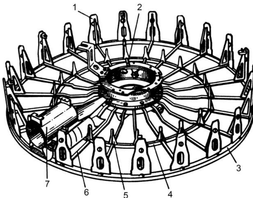
Рис. 5.63. Каркас ВТ с погонным устройством:
