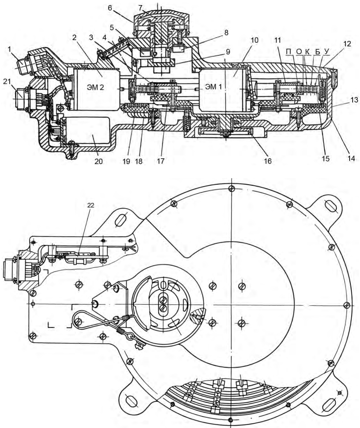
Рис. 5.80. Запоминающее устройство:
