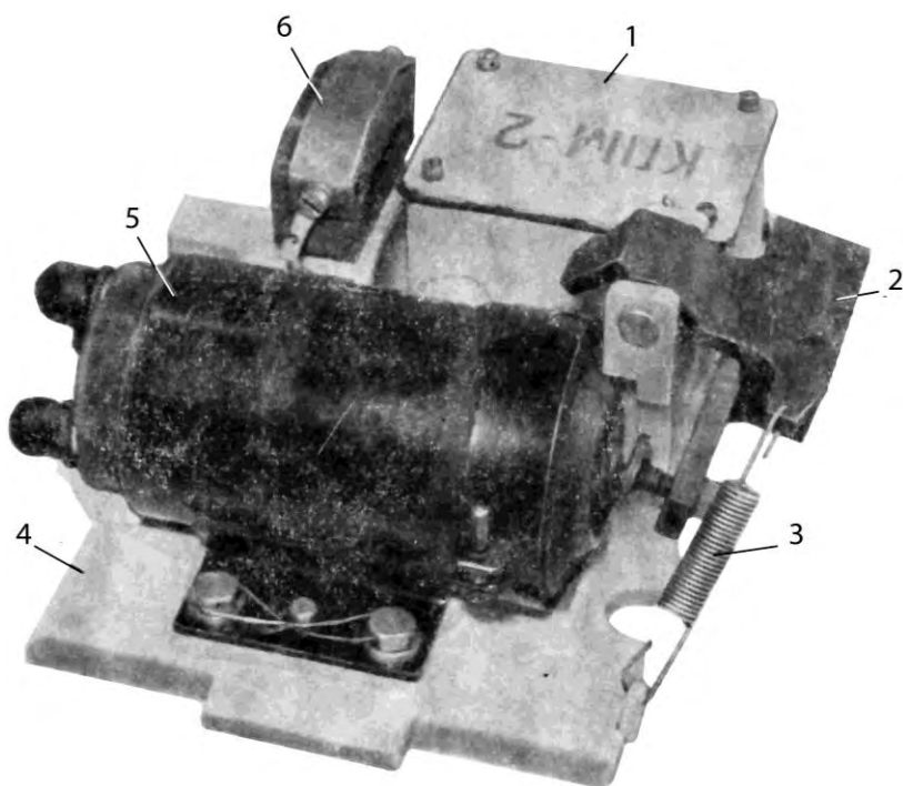
Рис. 5.8. Общий вид спускового механизма: 1 – соединительный блок; 2 – полка в сборе; 3 – пружина нажима; 4 – основание; 5 – электромагнит; 6 – контактная пластина
