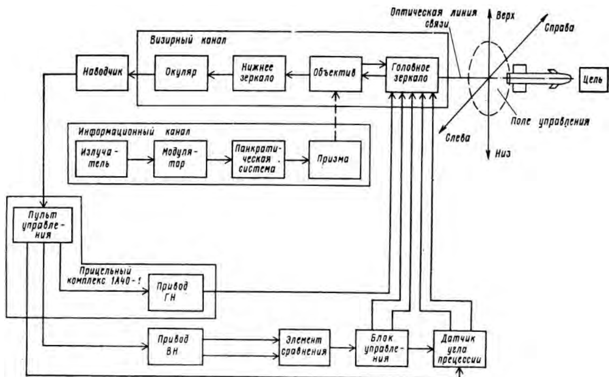
Рис. 5.52. Структурная схема системы управления комплекса 9К120
