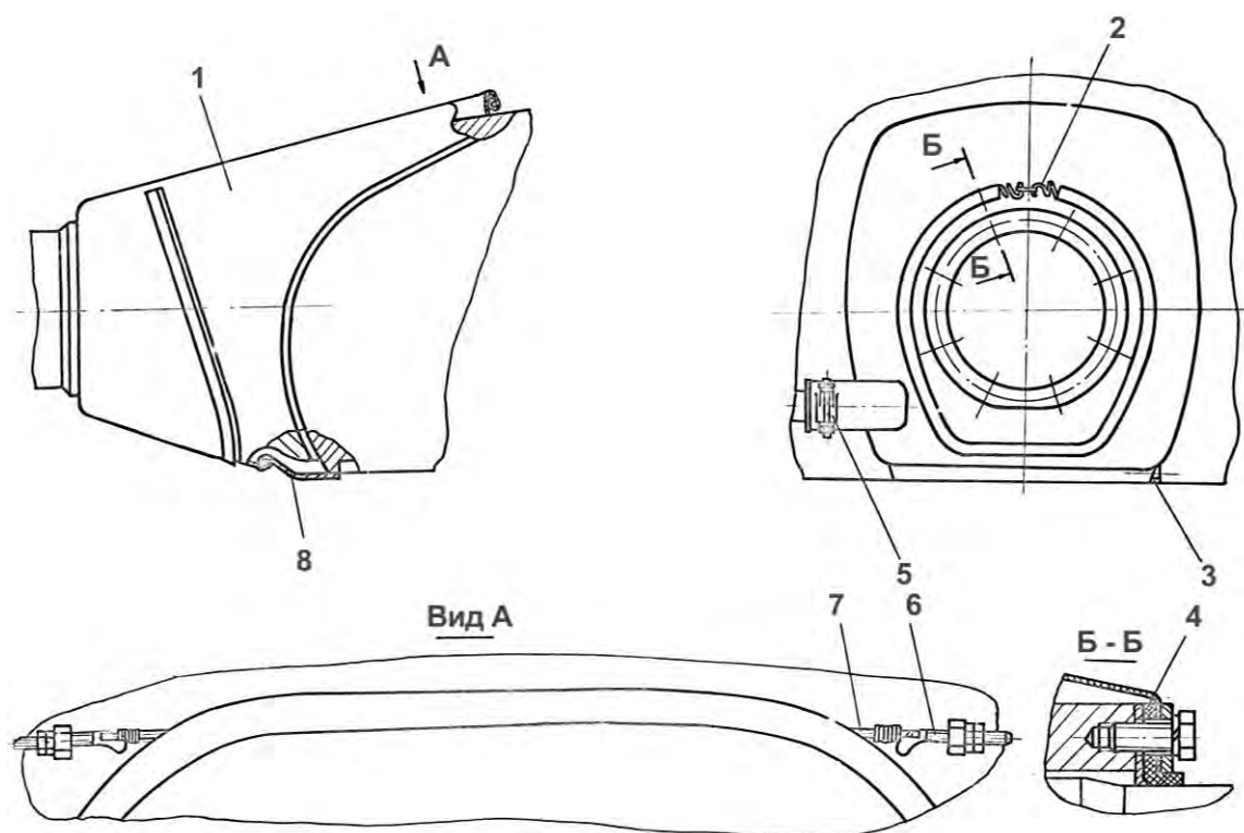
Рис. 16.5. Уплотнение броневой защиты пушки: 1 – чехол; 2 – пружина; 3 – пробка; 4 – прокладка; 5 – хомут; 6 – стяжка; 7 – трос; 8 – обечайка
