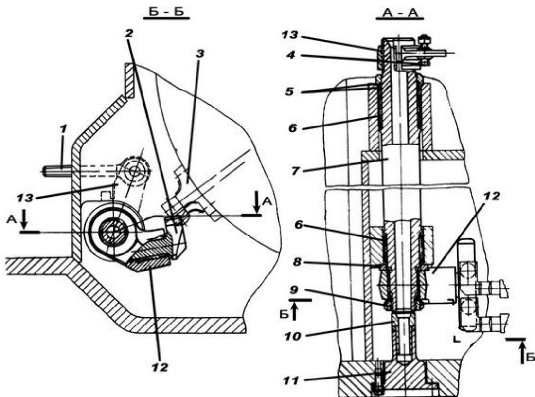
Рис. 9.14. Привод остановочного тормоза левой КП:
