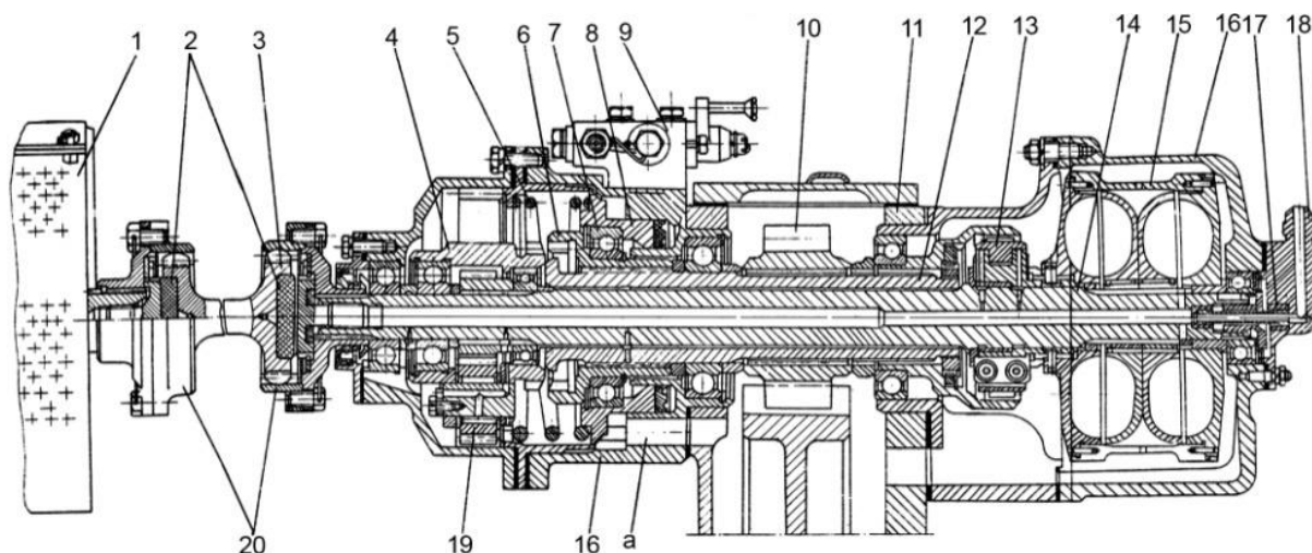
Рис. 9.4. Привод стартера-генератора:
