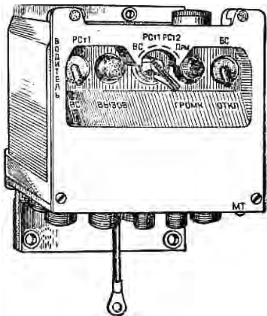
Рис. 12.3. Прибор БВ34
