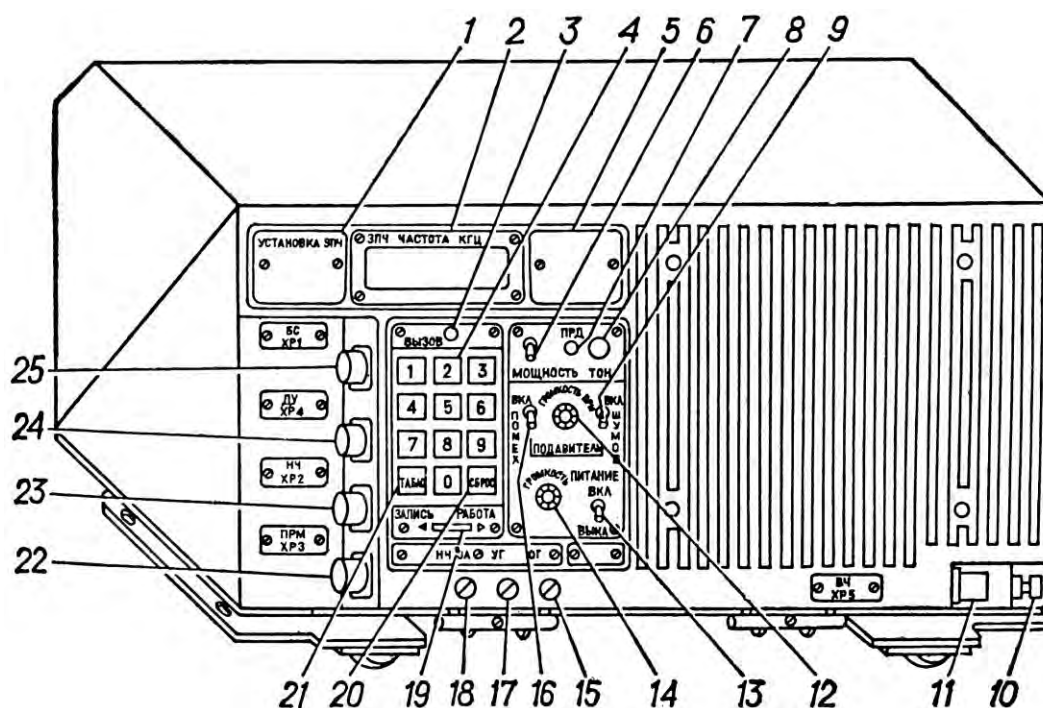
Рис. 12.1. Органы управления, регулирования и контроля радиостанции 1 – памятка УСТАНОВКА ЗПЧ; 2 – табло ЗПЧ и ЧАСТОТА кГц для цифровой индикации ЗПЧ и рабочей частоты; 3 – световой индикатор тонального вызова ВЫЗОВ; 4 – кнопки выбора и подготовки ЗПЧ; 5 – планка для карандашных пометок; 6 – тумблер МОЩНОСТЬ для перевода радиостанции в режим полной или малой мощности; 7 – световой индикатор режима передачи ПРД; 8 – кнопка ТОН для посылок тонального вызова; 9 – тумблер ПОДАВИТЕЛЬ ШУМОВ; 10 – клемма корпуса для подключения к массе объекта (минусовая шина бортсети); 11 – высокочастотный разъем ВЧ ХР5 для подключения антенны или БАФ; 12 – ручка ГРОМКОСТЬ ПРМ для регулирования громкости сигнала радиоприемника Р-173П; 13 – тумблер включения питания радиостанции; 14 – ручка регулятора громкости ГРОМКОСТЬ; 15, 17 и 18 – пробки; 16 – тумблер ПОДАВИТЕЛЬ ПОМЕХ; 19 – фиксатор ЗАПИСЬ–РАБОТА; 20 – кнопка СБРОС для стирания ЗПЧ; 21 – кнопка ТАБЛО; 22 – разъем ПРМ ХР3 для подключения радиоприемника Р-173П; 23 – разъем НЧ ХР2 для подключения переговорного устройства; 24 – разъем ДУ ХР4 для подключения питания БАФ; 25 – разъем БС ХР1 для подключения плюсовой шины бортсети машины
