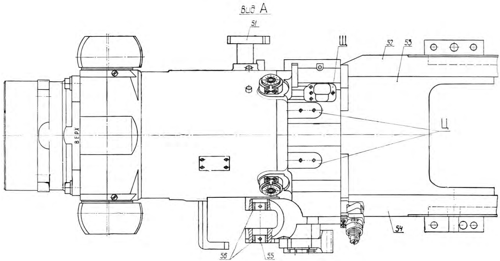
Рис. 5.11. Люлька (продолжение)
