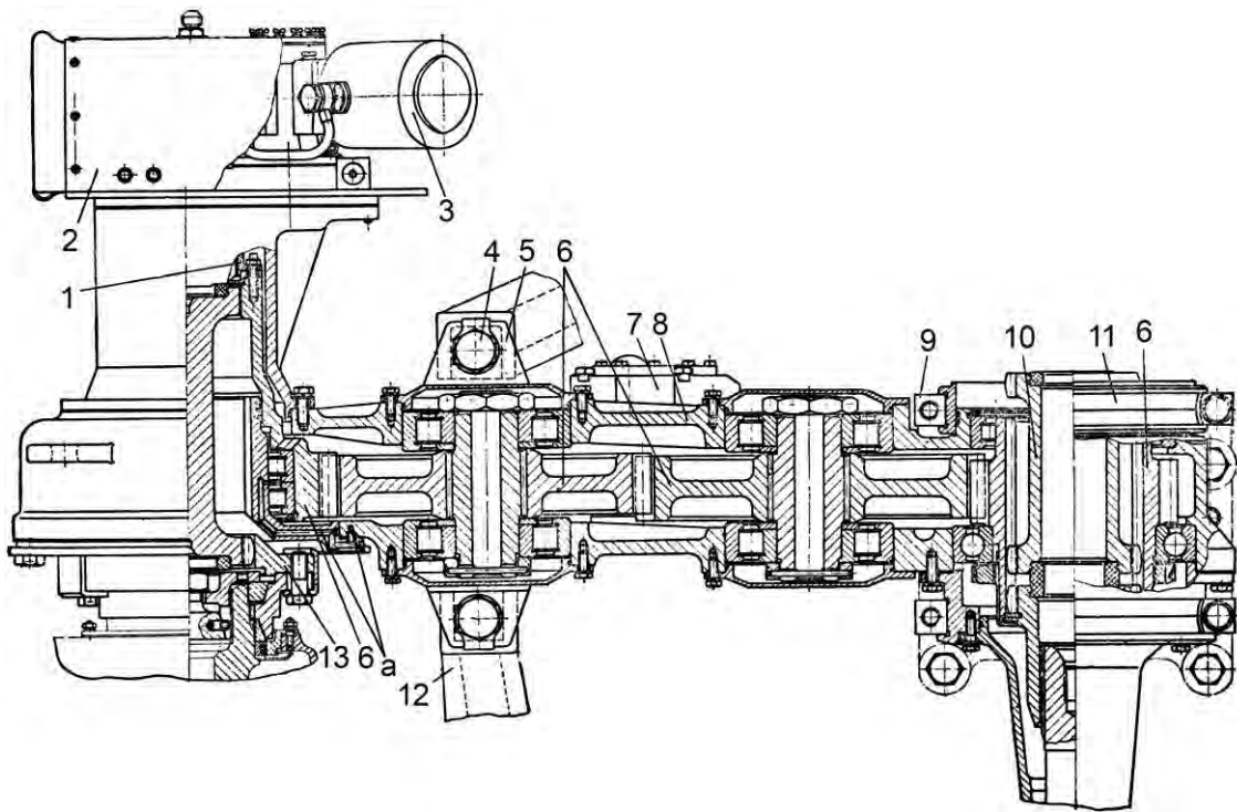
Рис. 9.1. Гитара:
