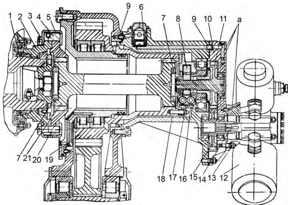
Рис. 9.2. Привод компрессора:
