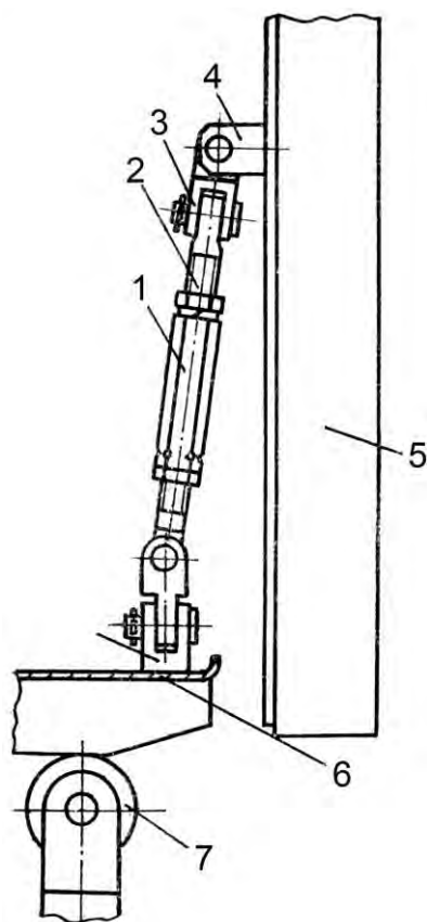
Рис. 5.67. Стяжка:
