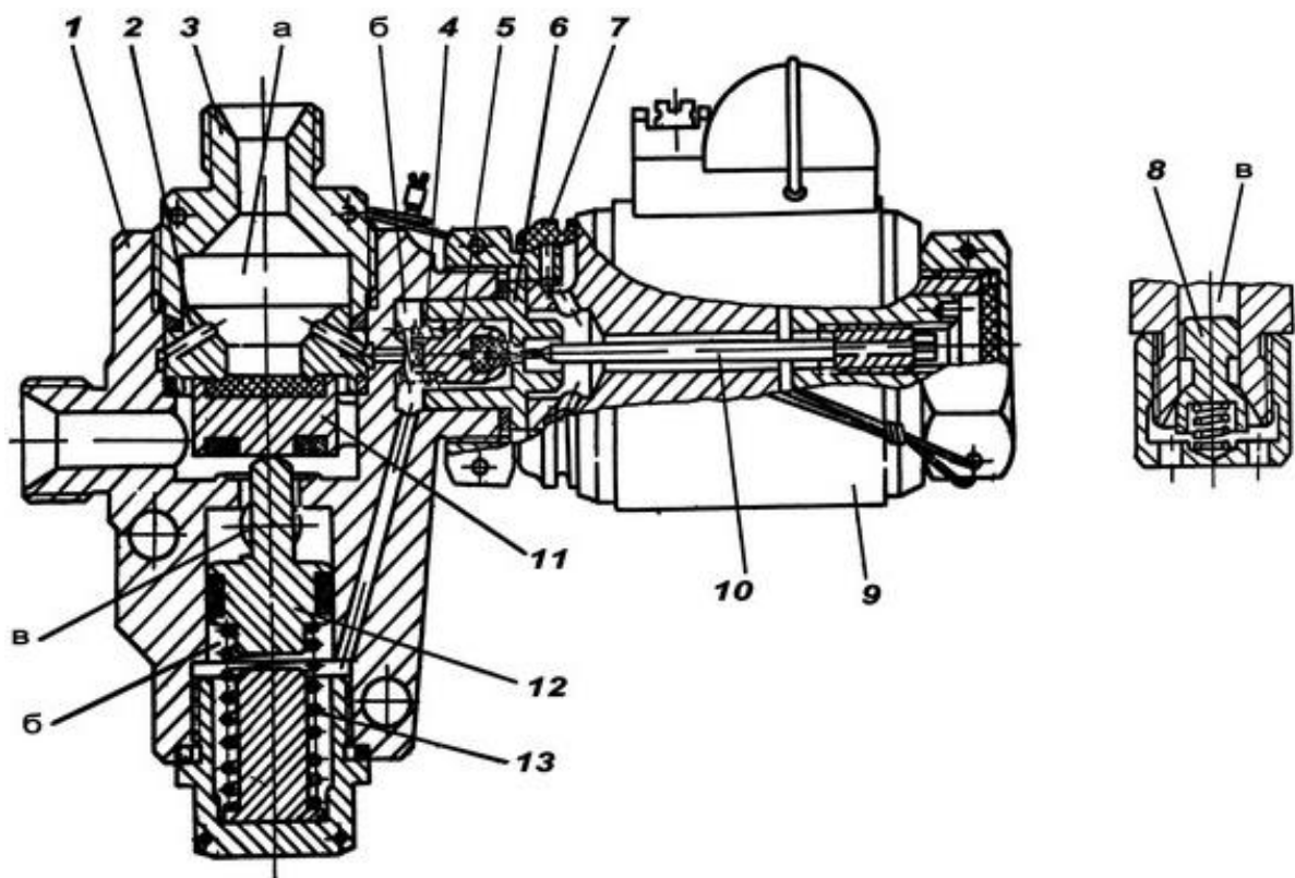
Рис. 8.42. Пусковой клапан:
