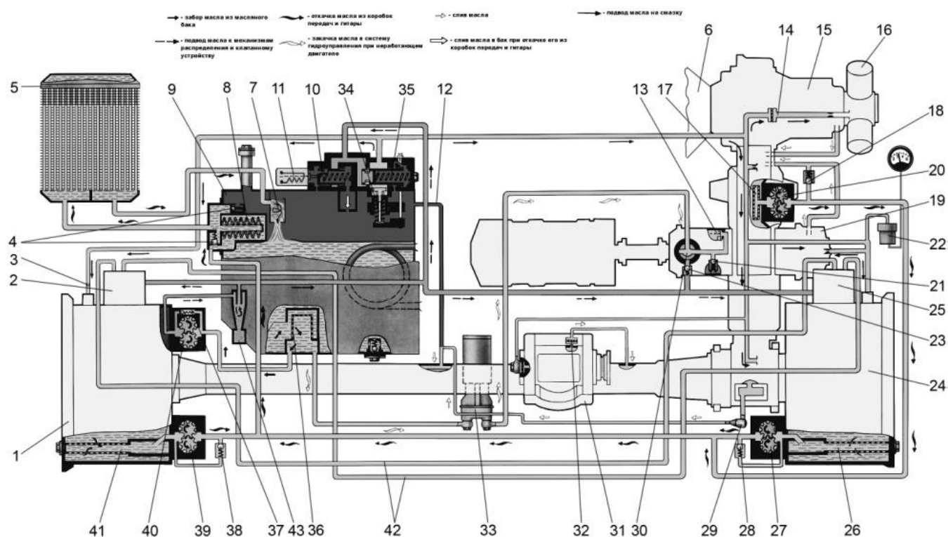
Рис. 9.18. Система гидроуправления и смазки силовой передачи. Схема гидравлическая принципиальная:
