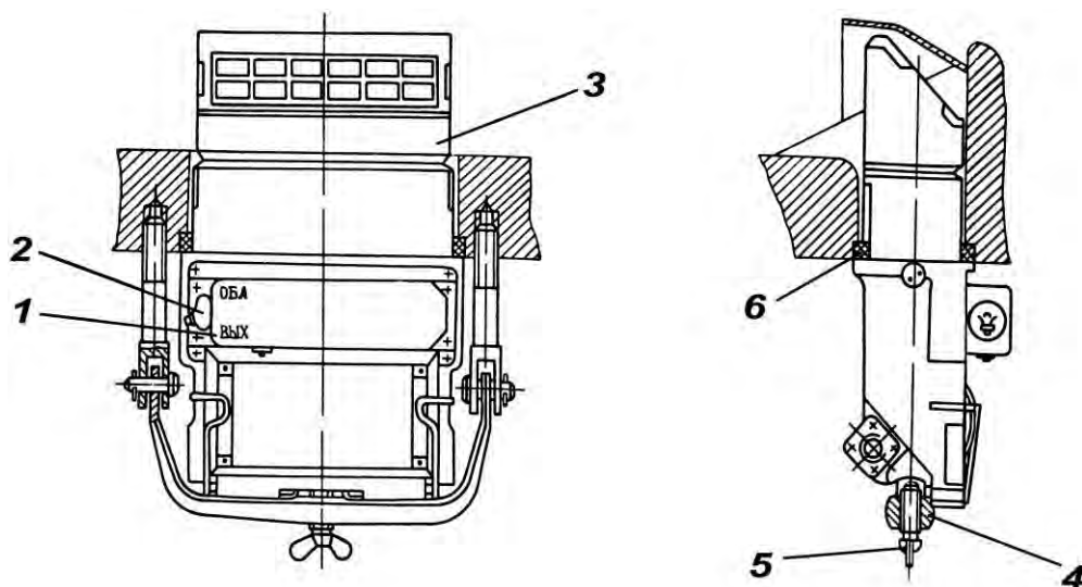
Рис. 6.3. Установка прибора ТНПО-160:
