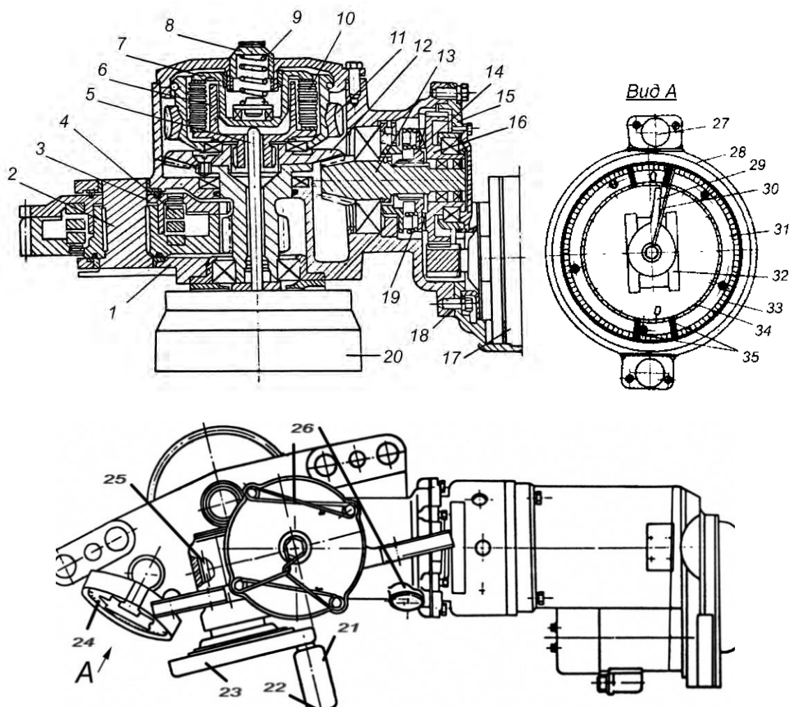
Рис. 4.12. Электромеханический механизм поворота и азимутальный указатель: 1 – картер; 2 – эксцентриковая ось; 3 – разрезная шестерня; 4 – пружина; 5 – шток; 6 – ведомый барабан со шлицами; 7 – нажимной барабан; 8 – пробка; 9 – пружина; 10 – диски фрикциона; 11 – червячная шестерня; 12 – коническое колесо; 13 – коническая шестерня; 14 – подвижная полумуфта сдающего звена; 15 – горловина; 16 – шестерня с неподвижной полумуфтой сдающего звена; 17 – электродвигатель; 18 – болт; 19 – пружина; 20 – электромагнит; 21 – рукоятка; 22 – кнопка; 23 – маховик; 24 – азимутальный указатель; 25 – червяк; 26 – пробка; 27 – светильник; 28 – корпус азимутального указателя; 29 – стрелка грубого отсчета; 30 – стрелка точного отсчета; 31 – диск; 32 – контур машины; 33 – шкала точного отсчета; 34 – шкала грубого отсчета; 35 – красные риски
