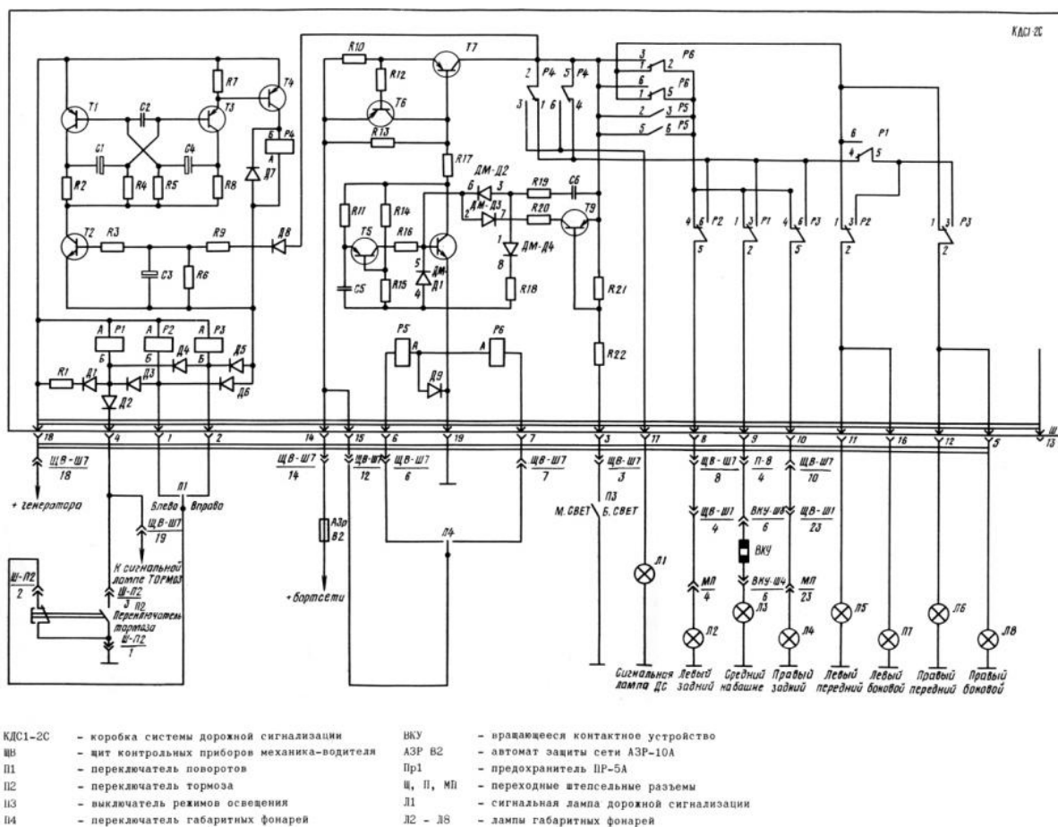
Рис. 11.3. Электрическая схема дорожной сигнализации
