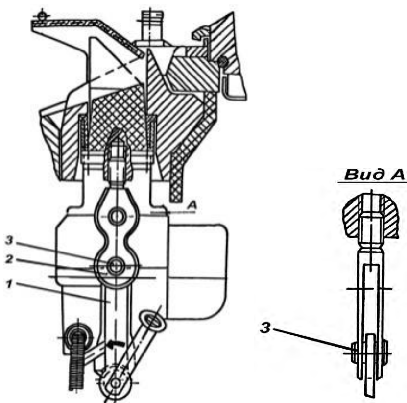
Рис. 6.6. Установка прибора ТВНЕ-4Б по-боевому:
