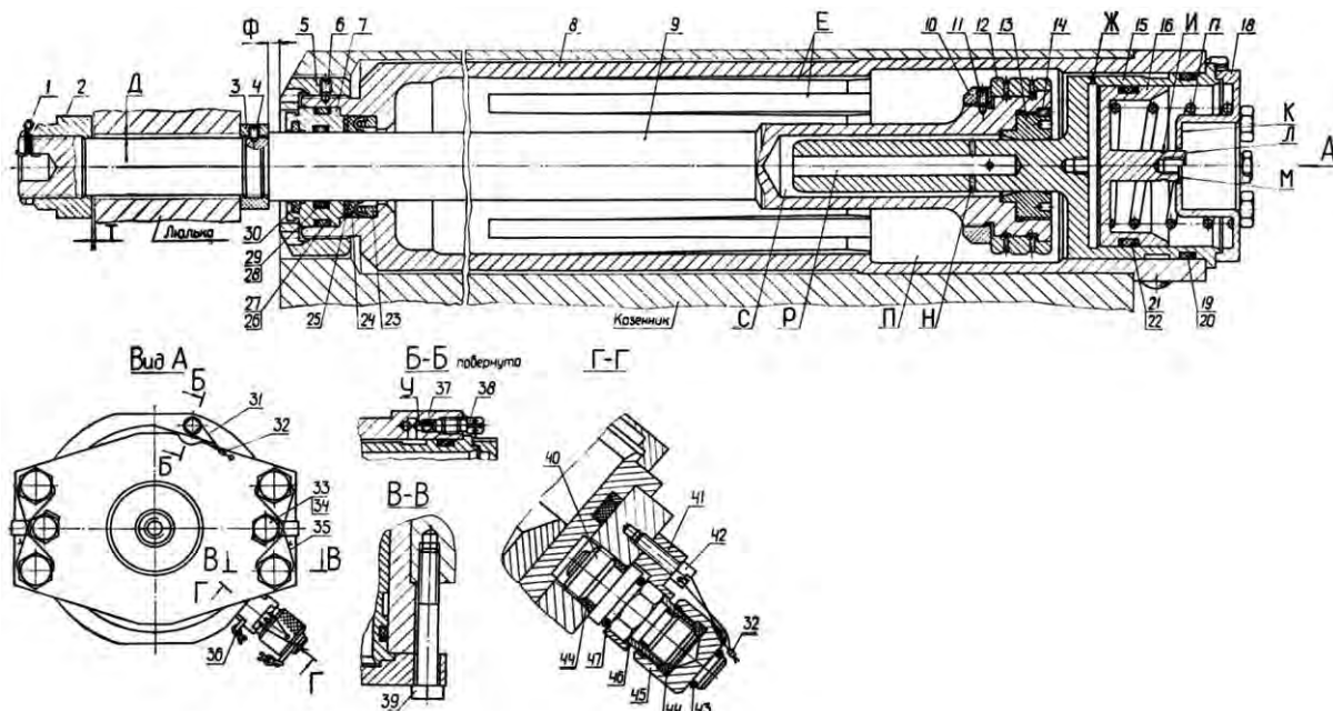
Рис. 5.9. Тормоз откатных частей:
