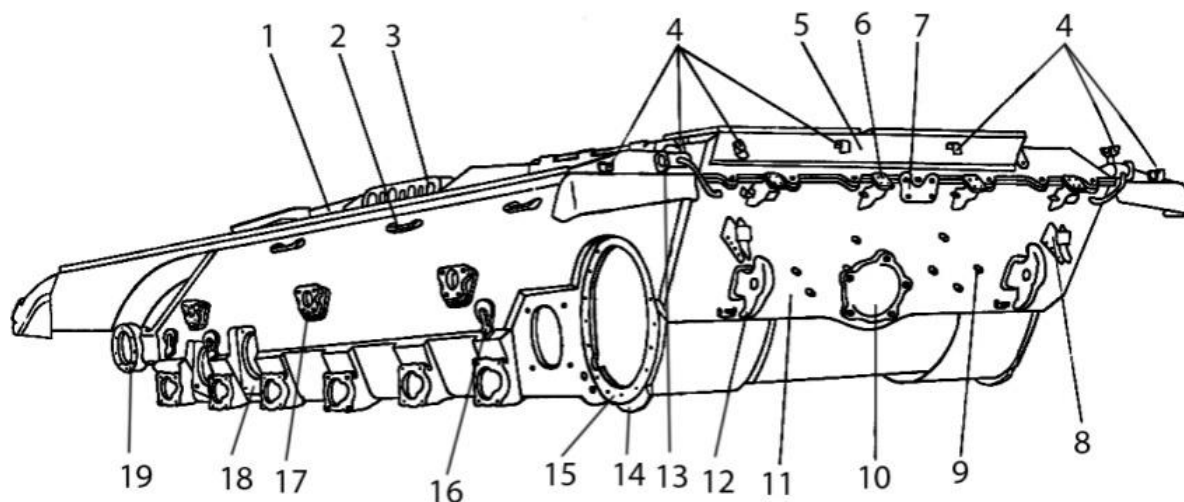
Рис. 3.2. Корпус. Вид сзади слева:
