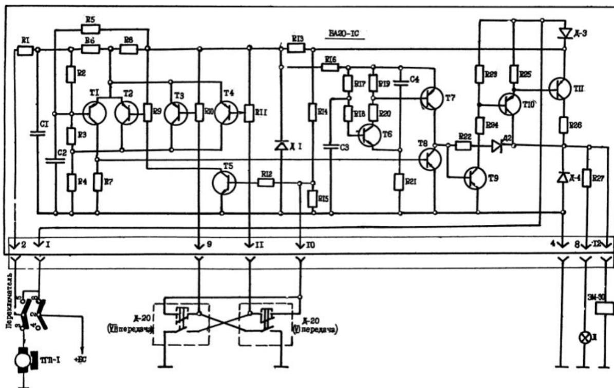
Рис. 9.11. Блокировка избирателя передач. Схема электрическая принципиальная
