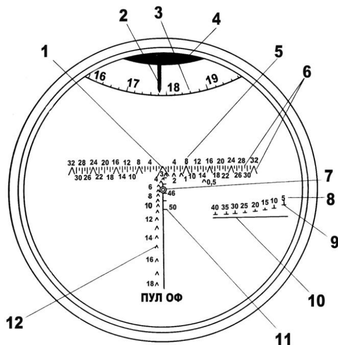
Рис. 5.31. Вид поля зрения 1А40-1:
