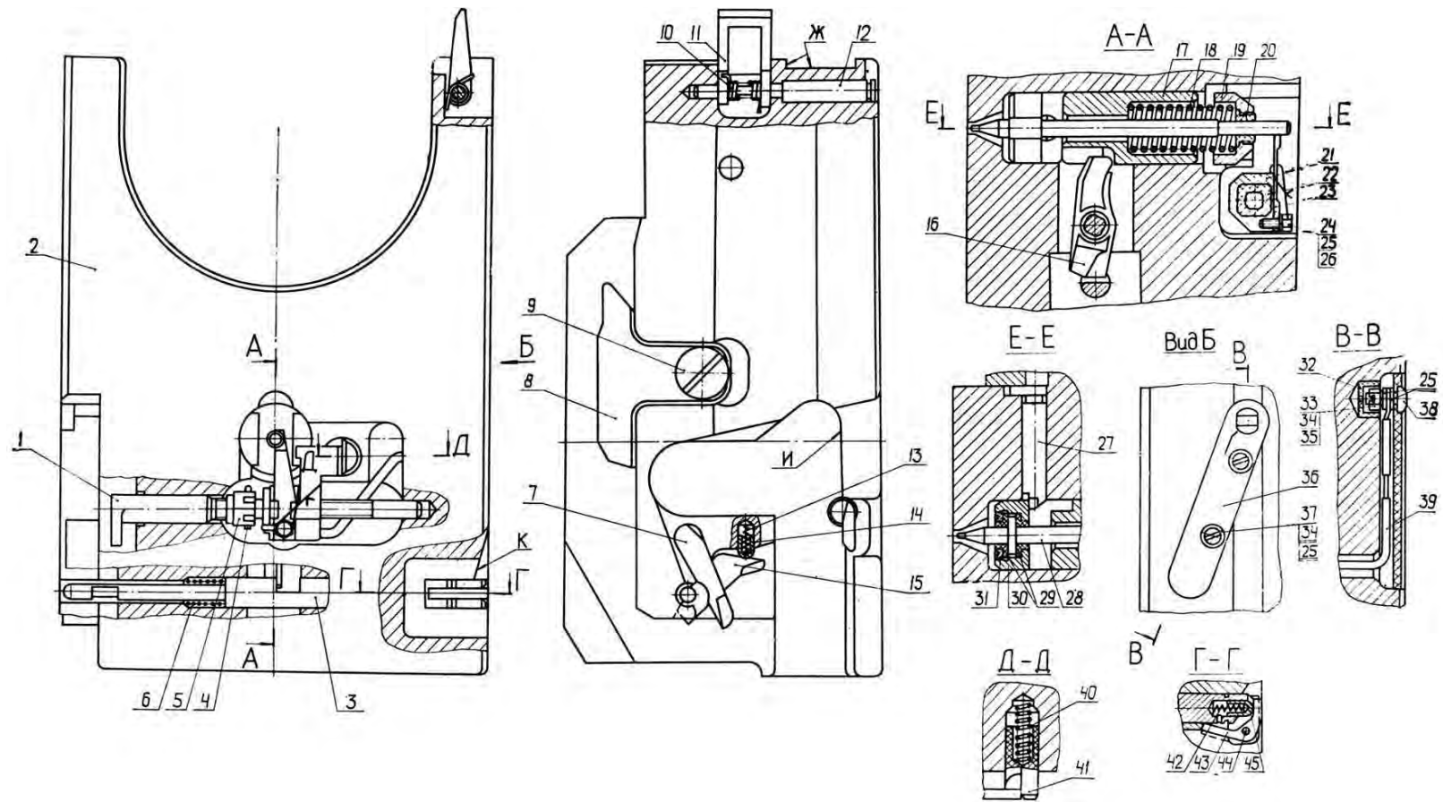
Рис. 5.5. Клин затвора:
