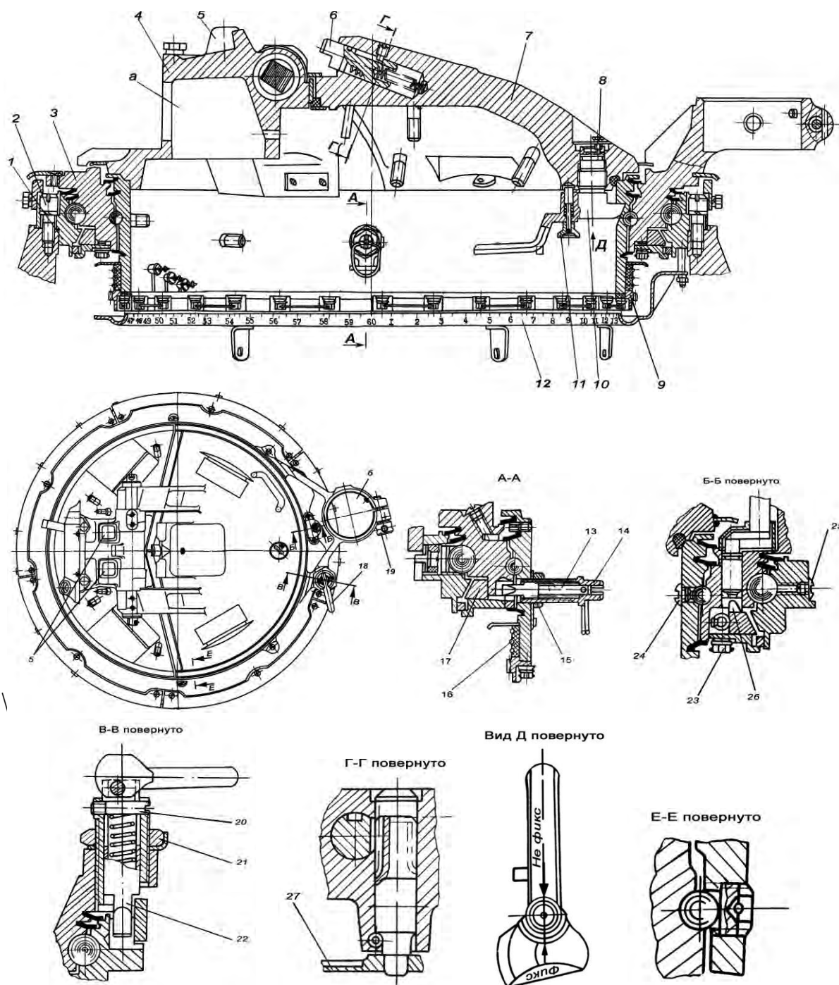
Рис. 4.13. Командирская башенка:
