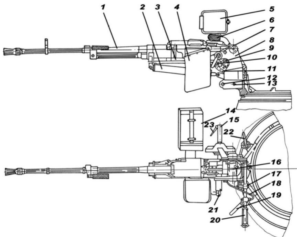
Рис. 5.15. Зенитно-пулеметная установка:
