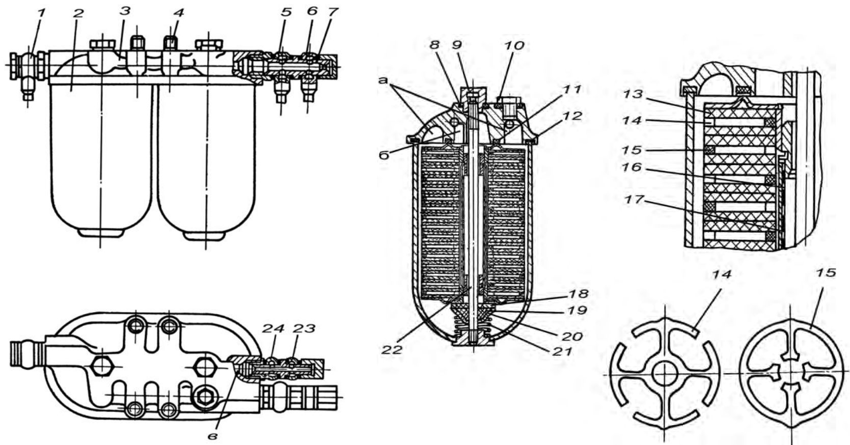
Рис. 8.8. Топливный фильтр тонкой очистки:
