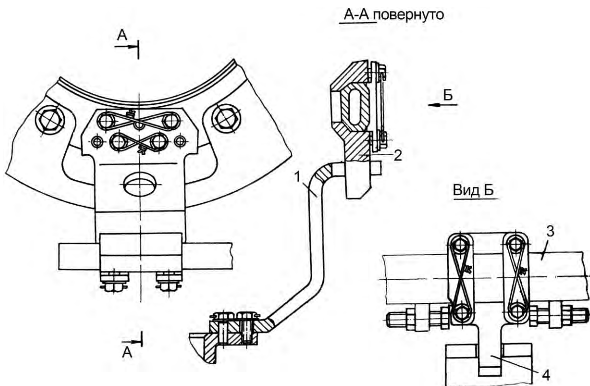
Рис. 5.64. Поводковое устройство: 1 – кронштейн; 2 – поводок; 3 – труба; 4 – штырь поводка
