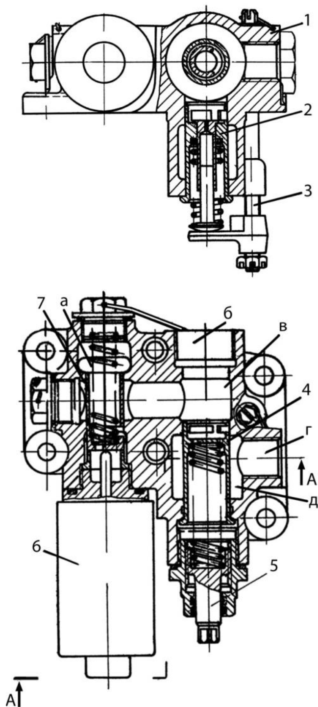
Рис. 9.19. Клапанное устройство:
