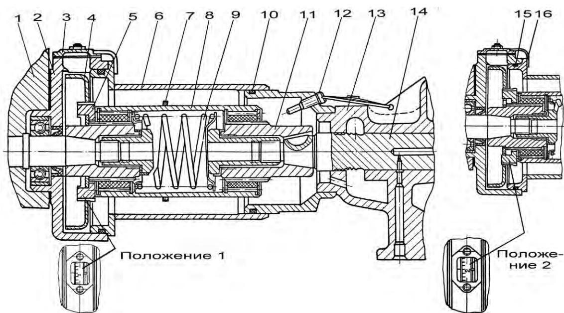
Рис. 8.10. Муфта привода топливного насоса:
