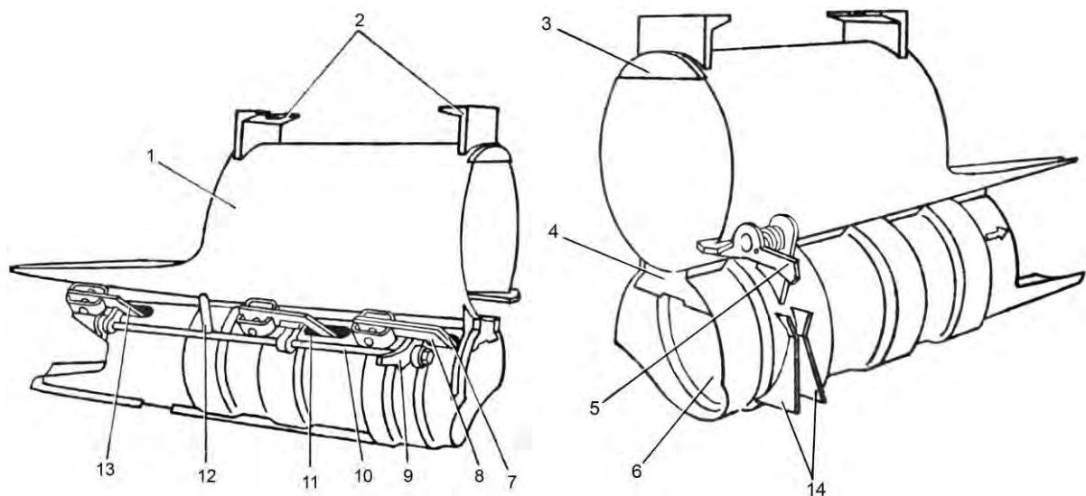
Рис. 5.66. Кассета:
