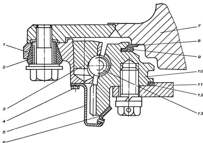
Рис. 4.10. Шариковая опора башни:
