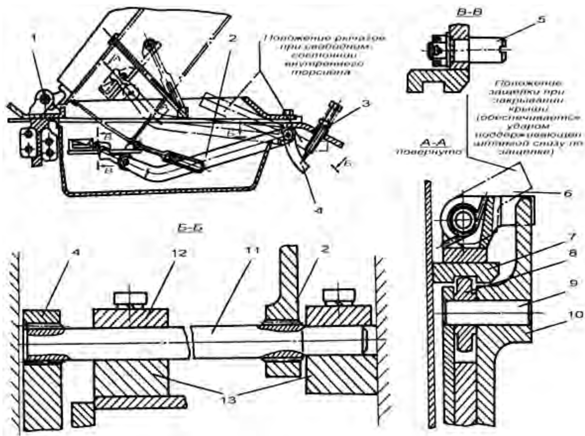
Рис. 4.6. Подъемное устройство крыши:
