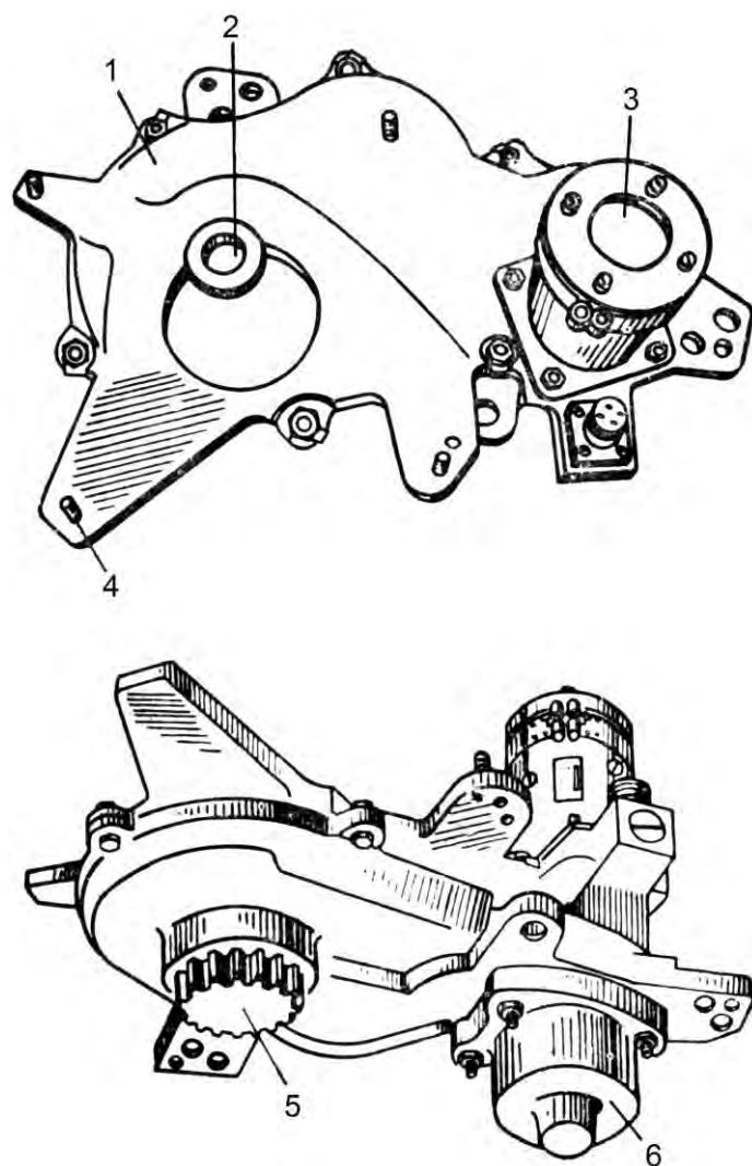
Рис. 5.65. Электромеханический привод ВТ: 1 – редуктор; 2 – шестерня; 3 – электродвигатель; 4 – шпилька; 5 – выходная шестерня; 6 – пружинное предохранительное звено
