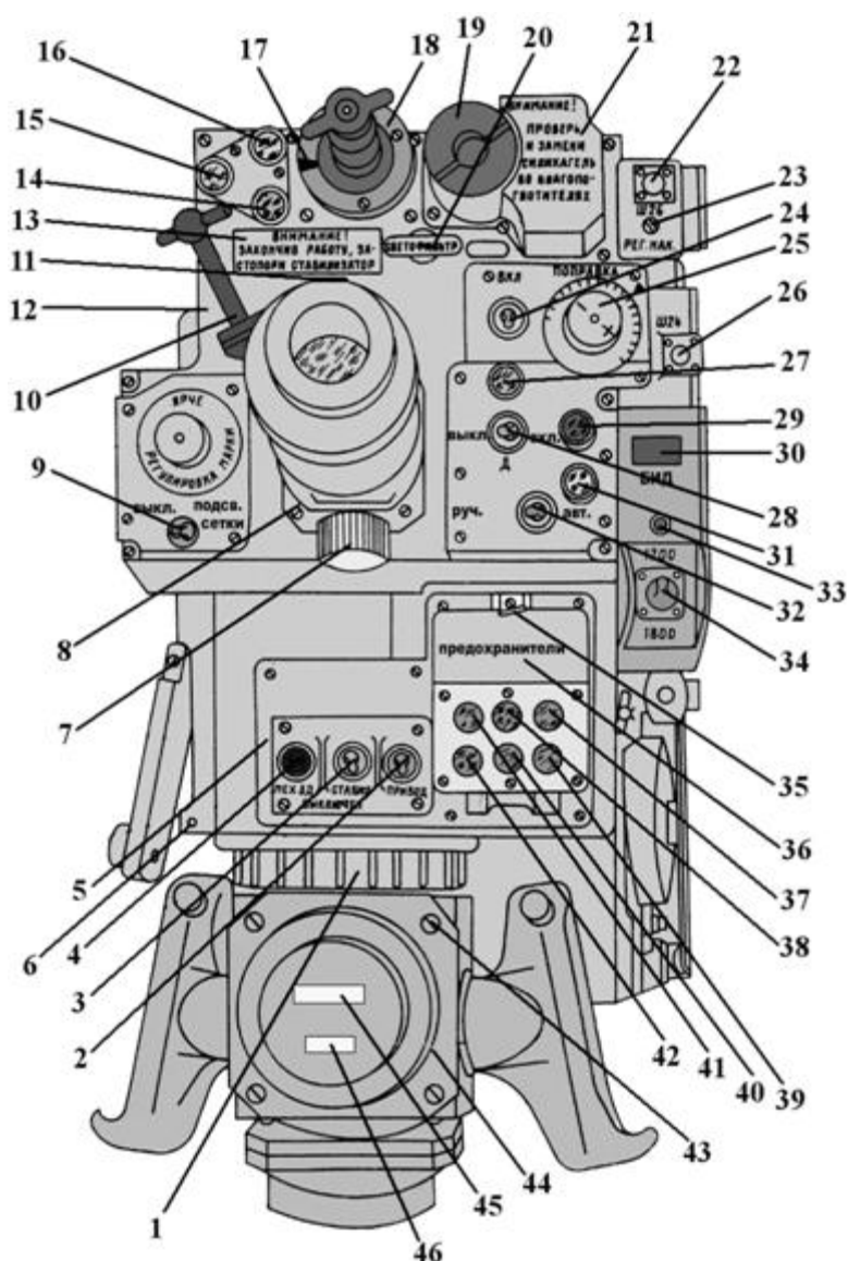
Рис. 5.33. Прибор управления (вид спереди):
