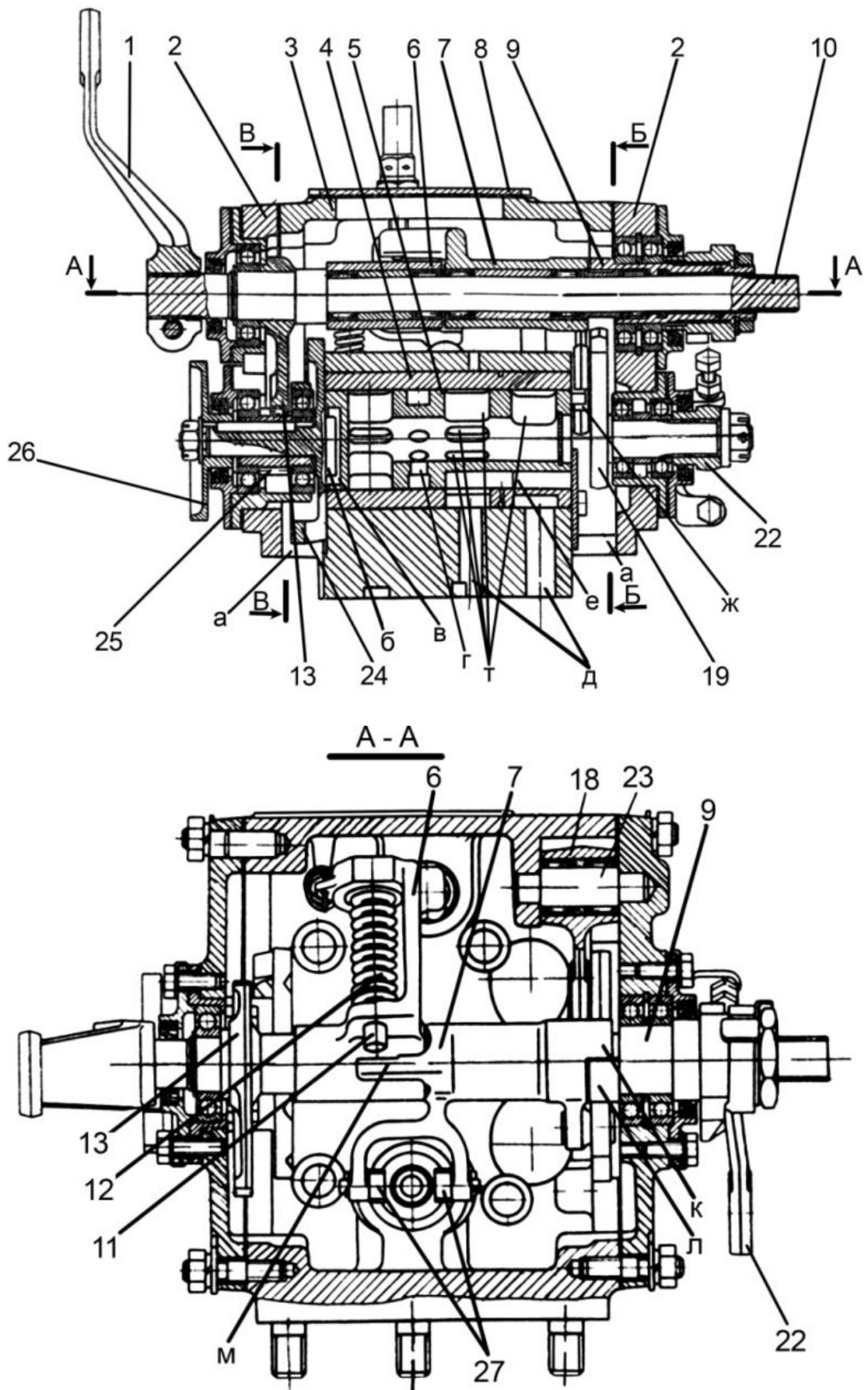
Рис. 9.15. Механизм распределения (начало)
