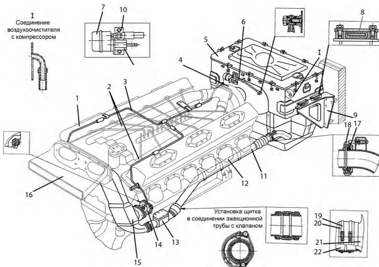
Рис. 8.16. Система питания двигателя воздухом и устройство для выпуска отработавших газов:
