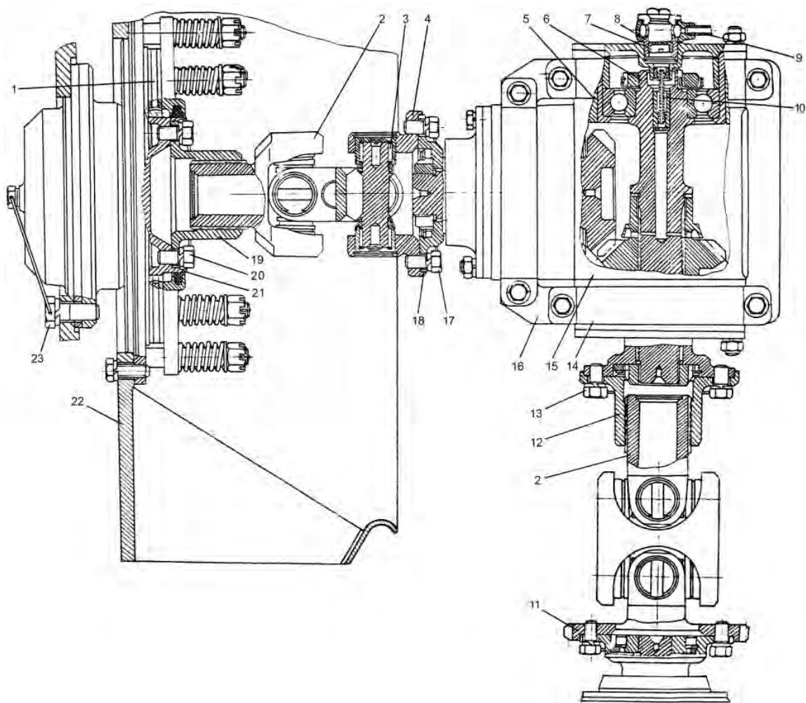
Рис. 9.5. Привод вентилятора:
