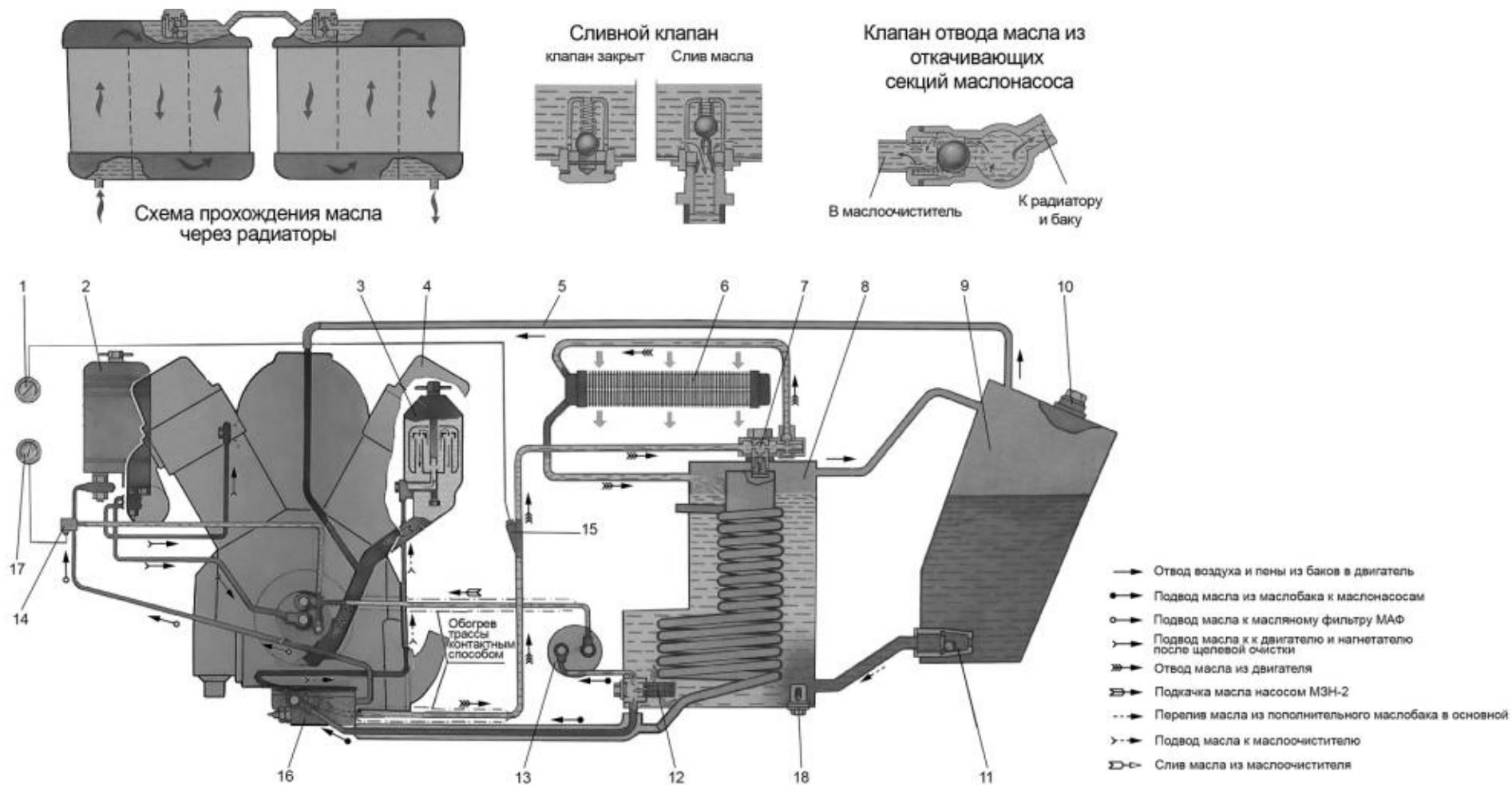
Рис. 8.26. Система смазки двигателя:
