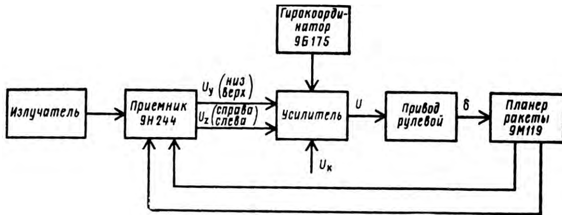
Рис. 5.53. Функциональная схема системы управления ракетой 9М119
