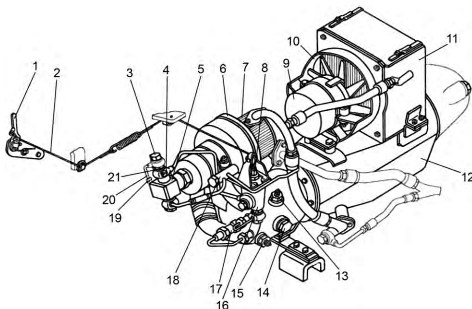
Рис. 8.33. Подогреватель:
