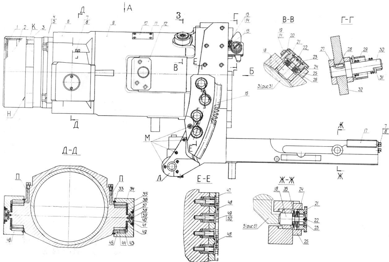
Рис. 5.11. Люлька (начало)
