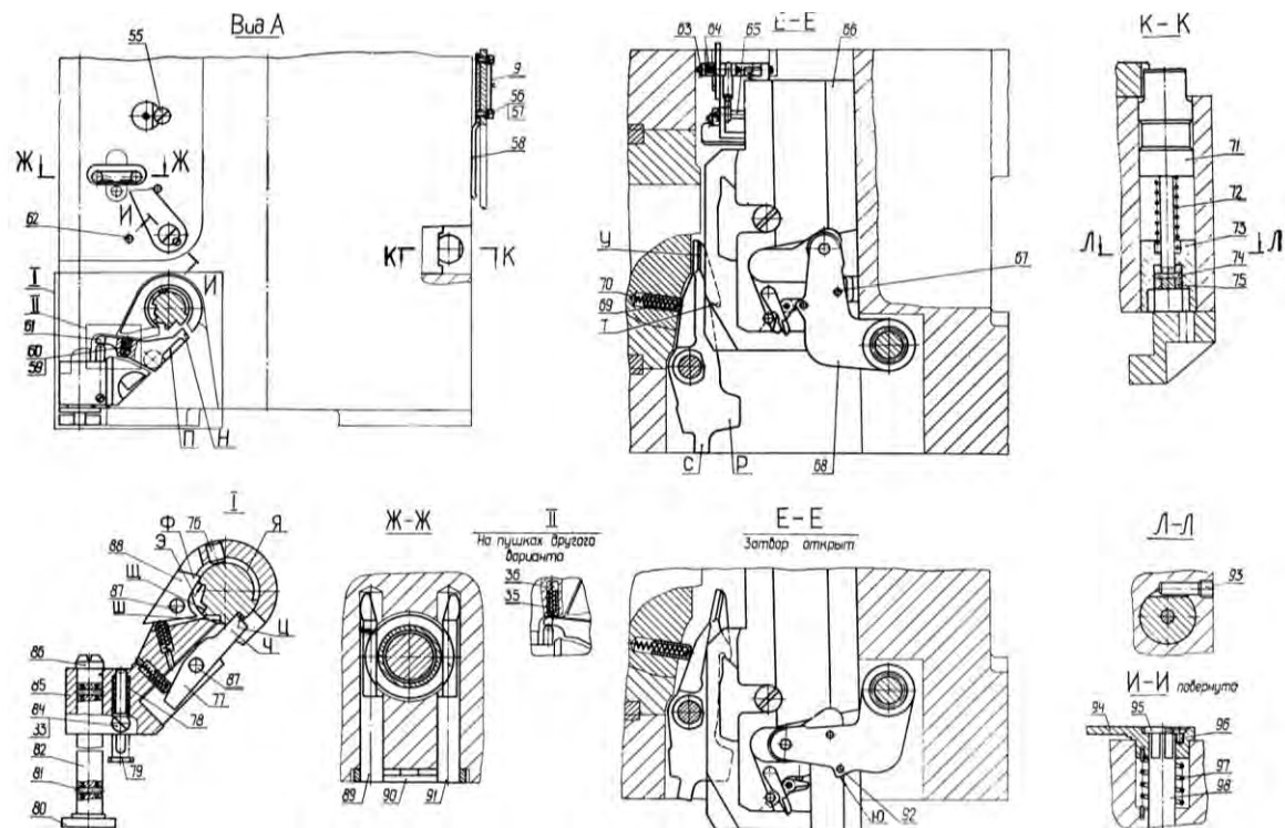
Рис. 5.4. Затвор (окончание):
