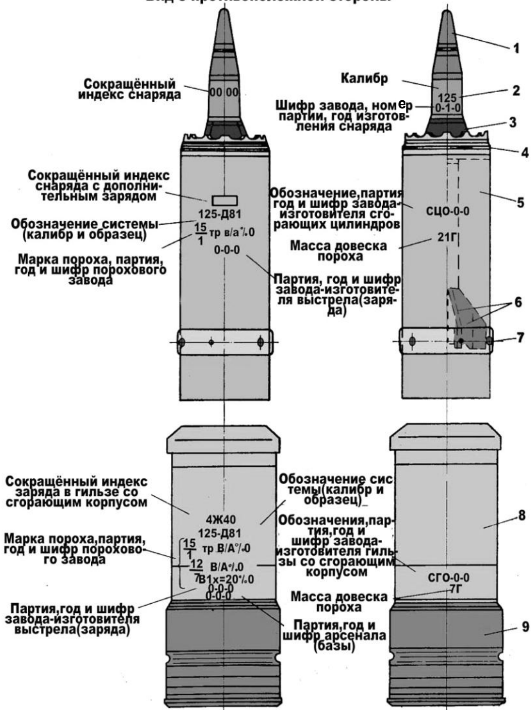
Рис. 5.22. Выстрел с бронебойным подкалиберным снарядом:
