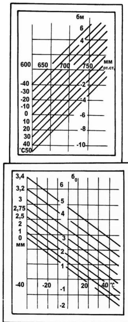
Рис. 5.37. Номограммы (пластина)
