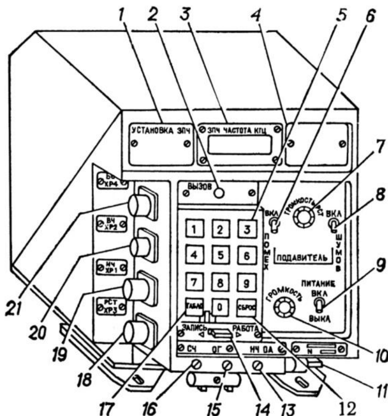
Рис. 12.2. Радиоприемник Р-173П:
