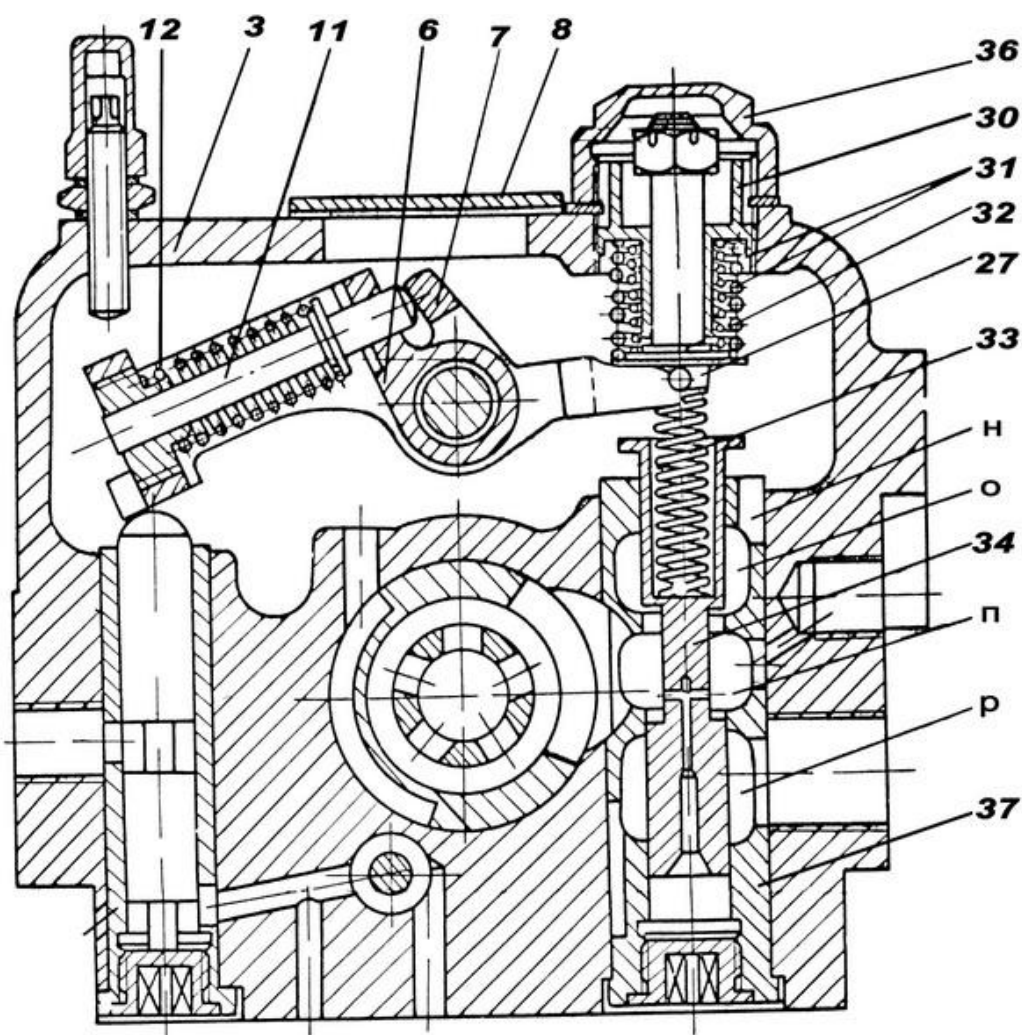
Рис. 9.17. Механизм распределения.
