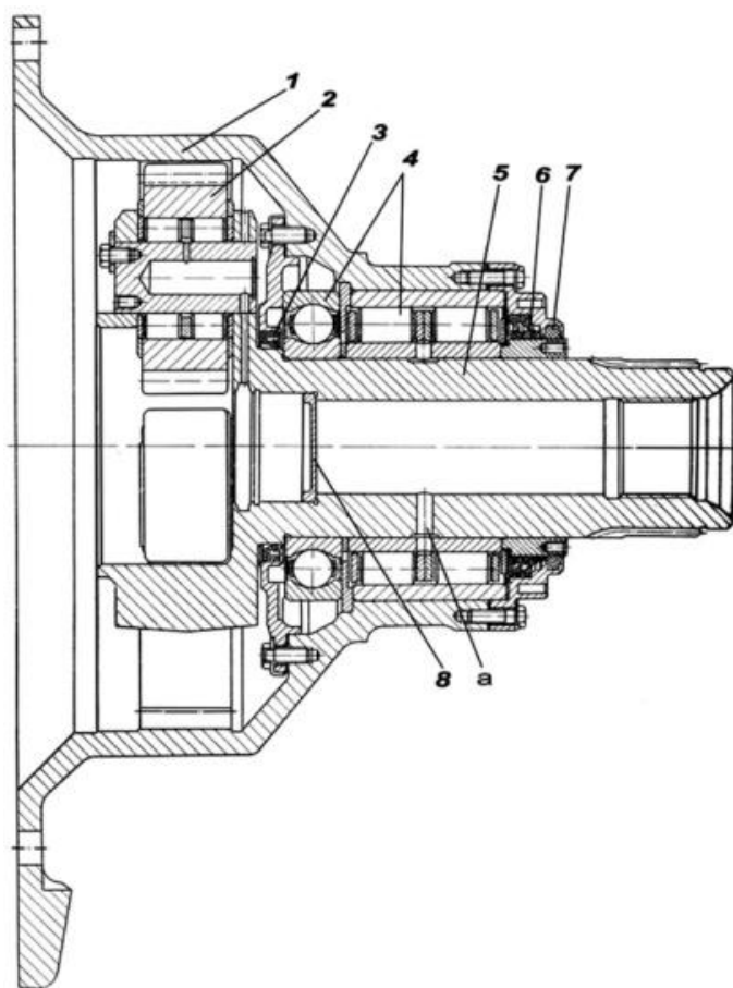
Рис. 9.9. Бортовая передача:
