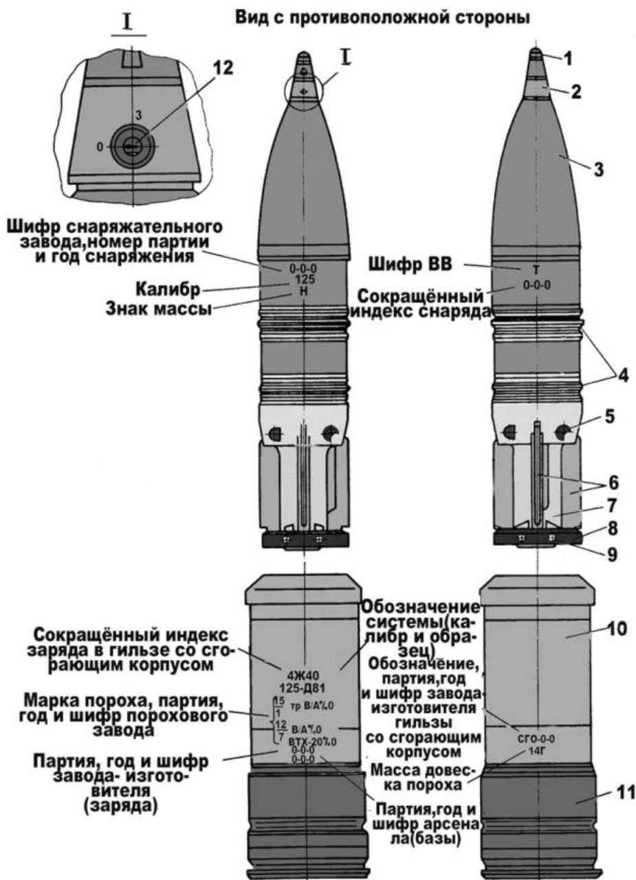
Рис. 5.25. Выстрел с осколочно-фугасным снарядом:
