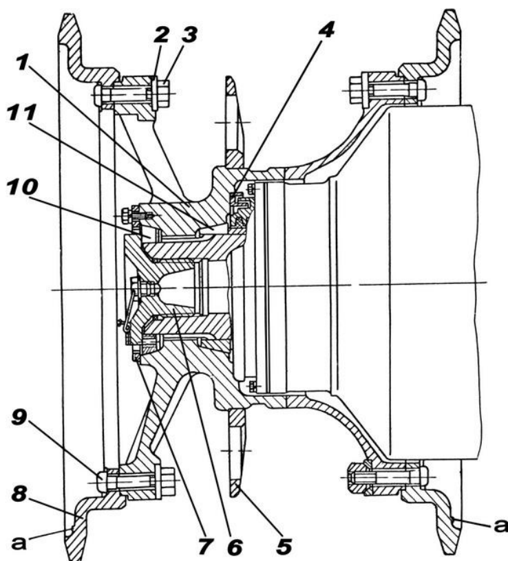
Рис. 10.1. Ведущее колесо:
