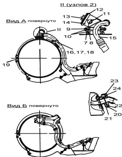
Рис. 8.4. Оборудование для подключения бочек: 1 – бочка; 2 – лента крепления бочки; 3 – скоба; 4 – палец; 5 – трубка к поплавковому клапану; 6 – наружный пятый бак; 7 – фланец горловины бочки; 8 – штуцер; 9 – хомут; 10 – прокладка; 11 – воздушный патрубок; 12 – прокладка; 13 – пробка; 14 – горловина; 15 – заборная трубка; 16 – болт; 17 – шайба; 18 – пружинная шайба; 19 – болт; 20 – прокладка; 21 – переходник; 22 – фланец; 23 – шайба; 24 – болт
