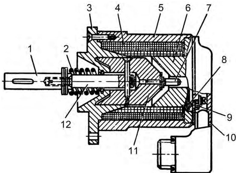
Рис. 5.74. Электромагнитный стопор МПК:
