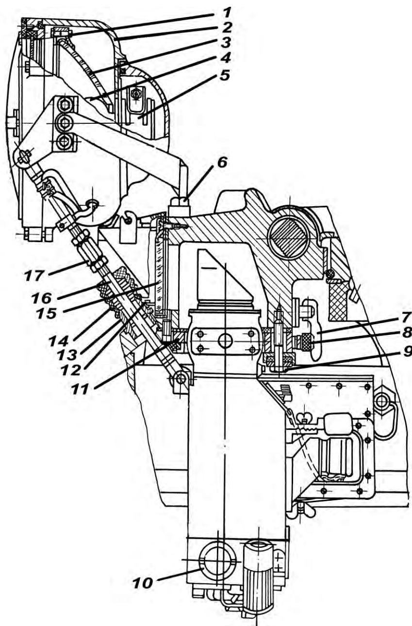
Рис. 6.2. Установка комплекта прибора ТКН-3:
