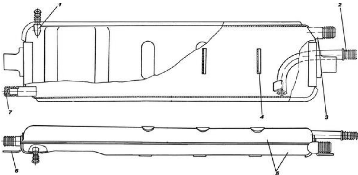
Рис. 8.29. Пополнительный бачок:
