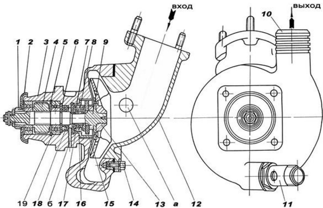
Рис. 8.31. Водяной насос:
