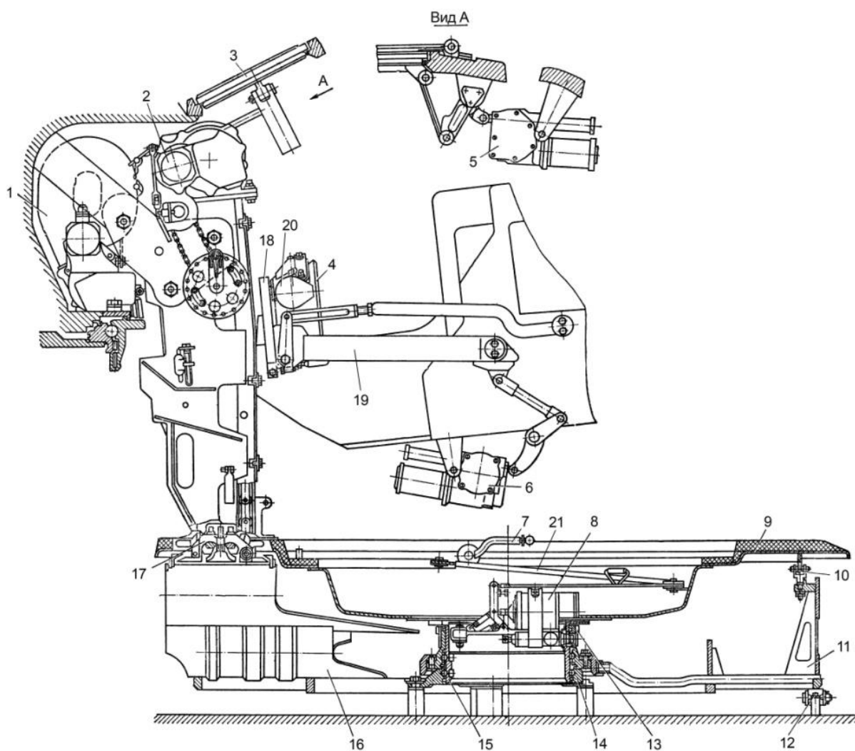
Рис. 5.60. Расположение узлов АЗ:
