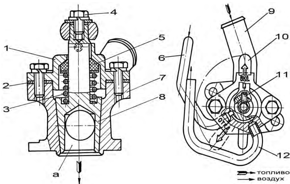
Рис. 8.6. Кран отклонения наружных топливных баков:
