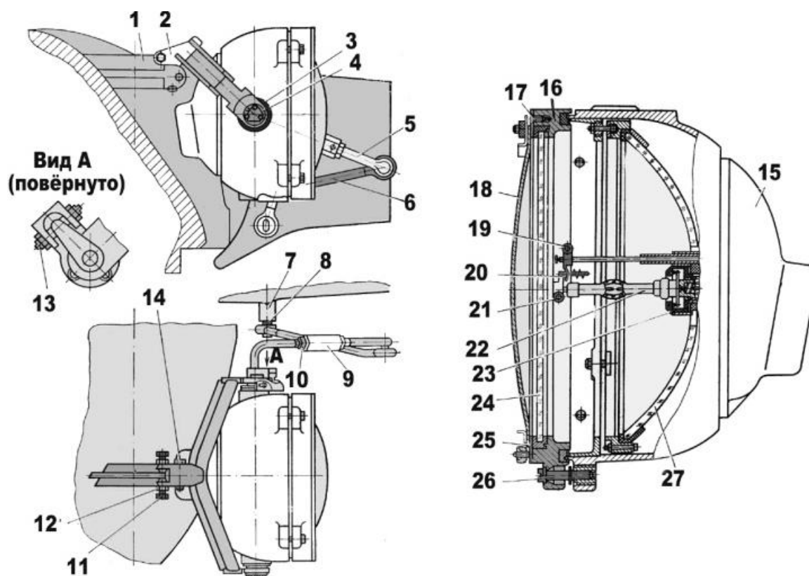
Рис. 5.59. Прожектор Л-4А:
