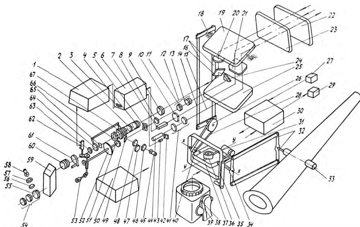
Рис. 5.36. Структурная схема изделия 1А40-1:
