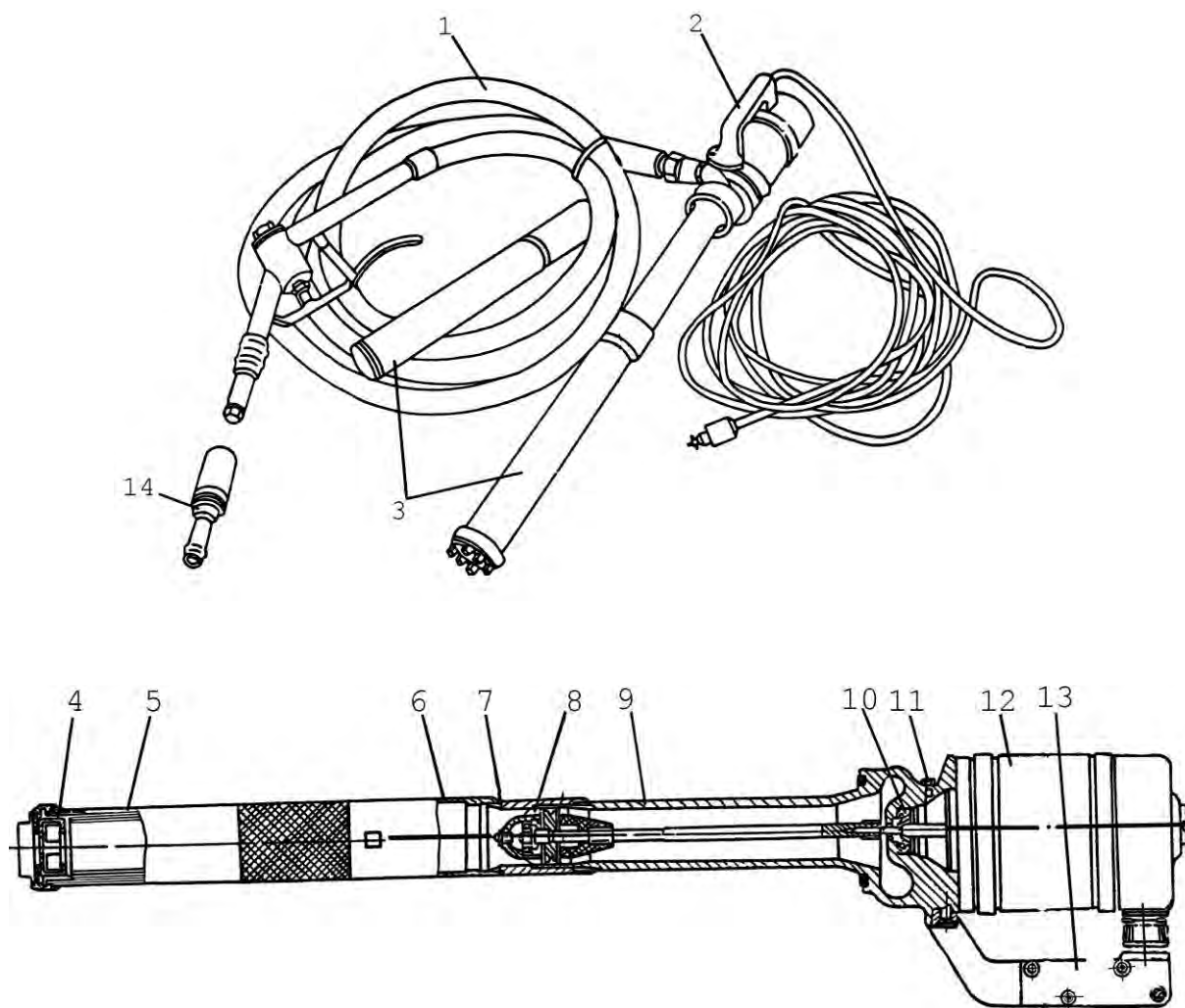
Рис. 8.15. Малогабаритный заправочный агрегат МЗА-3: 1 – шланг с раздаточным краном РК-25; 2 – насос в сборе с электродвигателем; 3, 6 – удлинители всасывающей трубы; 4 – обратный клапан; 5 – сетчатый фильтр; 7 – уплотнительное кольцо; 8 – осевой насос; 9 – корпус; 10 – сальник; 11 – винт отверстия для контроля за работой сальника; 12 – электродвигатель; 13 – рукоятка; 14 – переходник для заправки насосом МЗА-3 левого носового бака после полной выработки топлива
