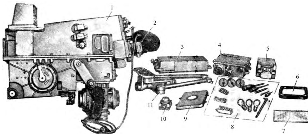
Рис. 5.27. Состав прицельного комплекса 1А40-1:
