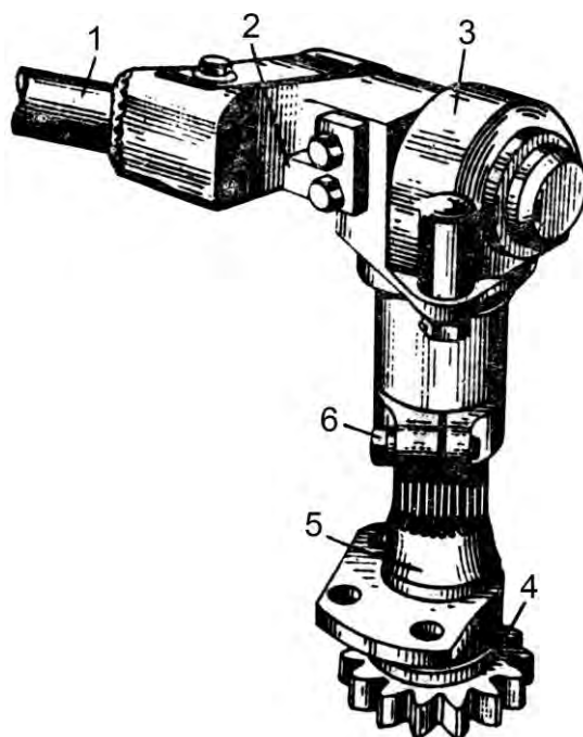
Рис. 5.71. Ручной привод ВТ: 1 – рукоятка; 2 – клин; 3 – головка; 4 – выходная шестерня; 5 – стойка; 6 – стяжной болт
