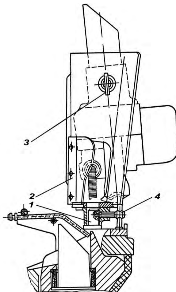
Рис. 6.7. Установка прибора ТВНЕ-4Б по-походному: 1 – ось; 2 – кронштейн; 3 – винт; 4 – стопор
