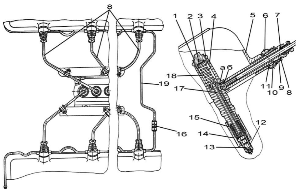
Рис. 8.12. Форсунка с объединенным сливом топлива:
