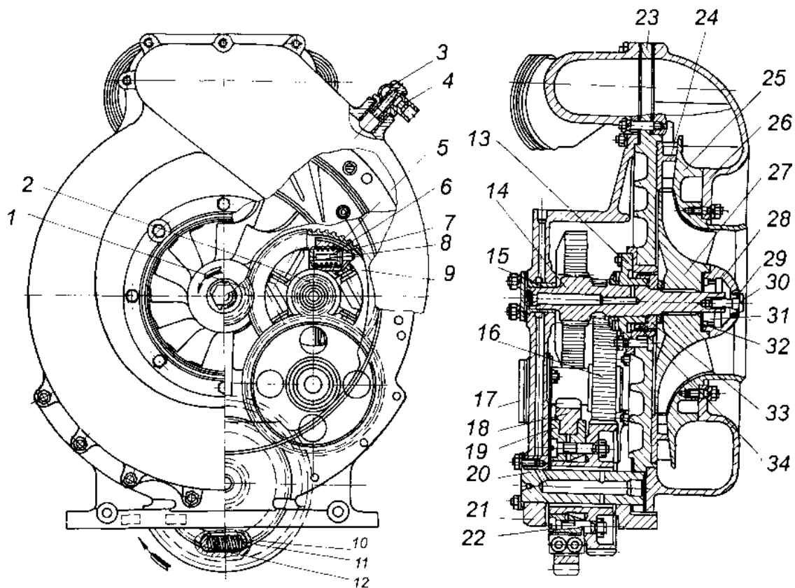
Рис. 8.2. Нагнетатель Н-46:
