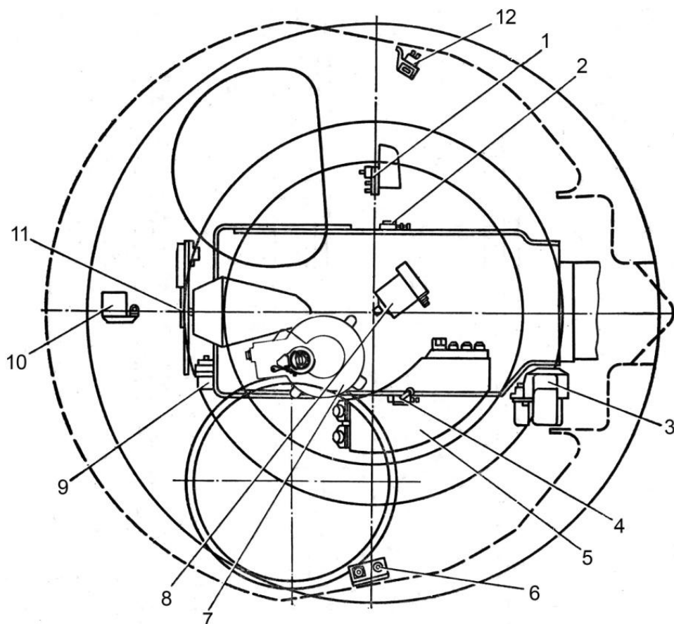
Рис. 5.61. Размещение электрооборудования АЗ:
