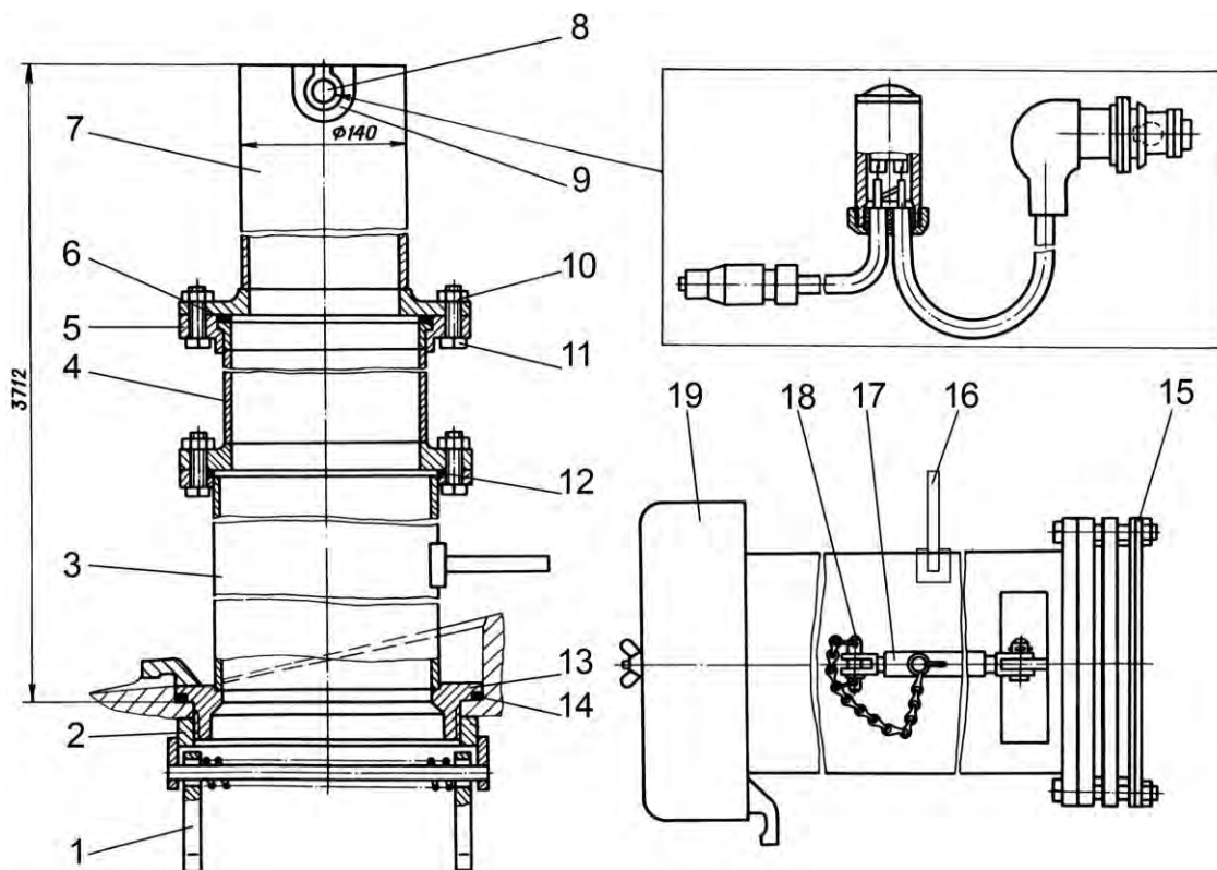
Рис. 16.2. Воздухопитающая труба:
