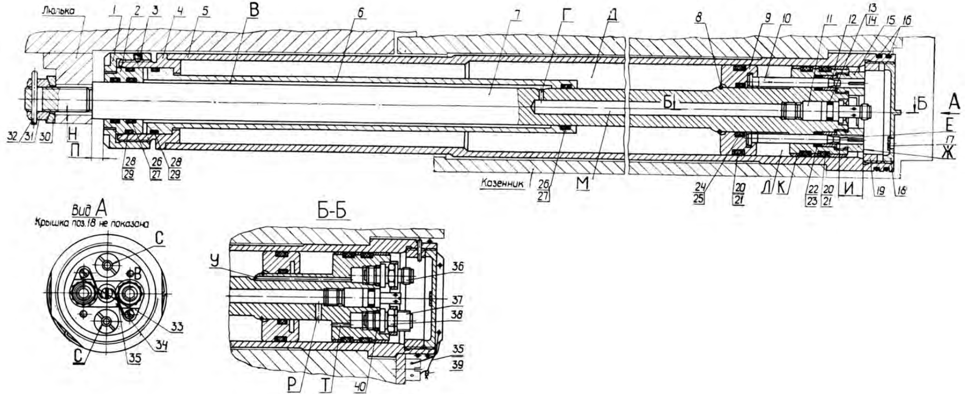
Рис. 5.10. Накатник:
