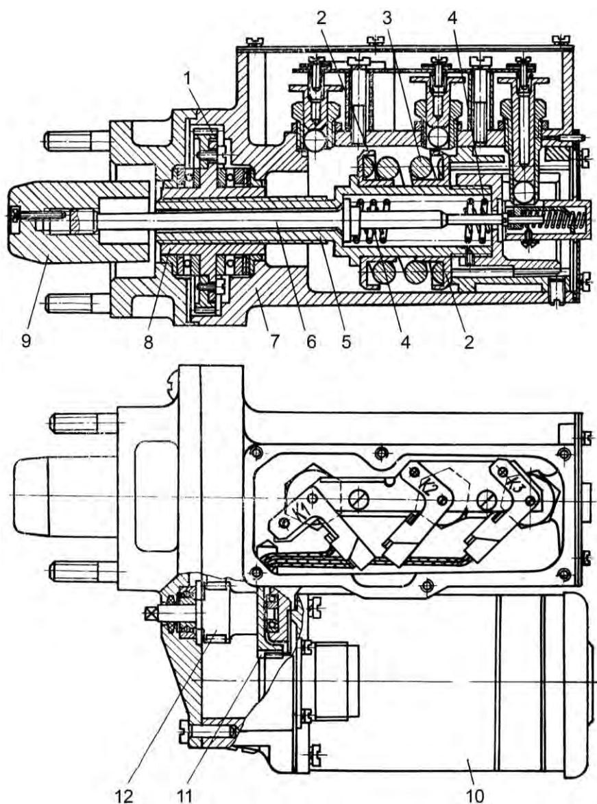
Рис. 5.79. Электромашинный стопор пушки:
