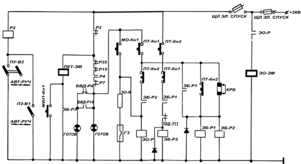
Рис. 5.21. Цепи стрельбы. Схема электрическая функциональная
