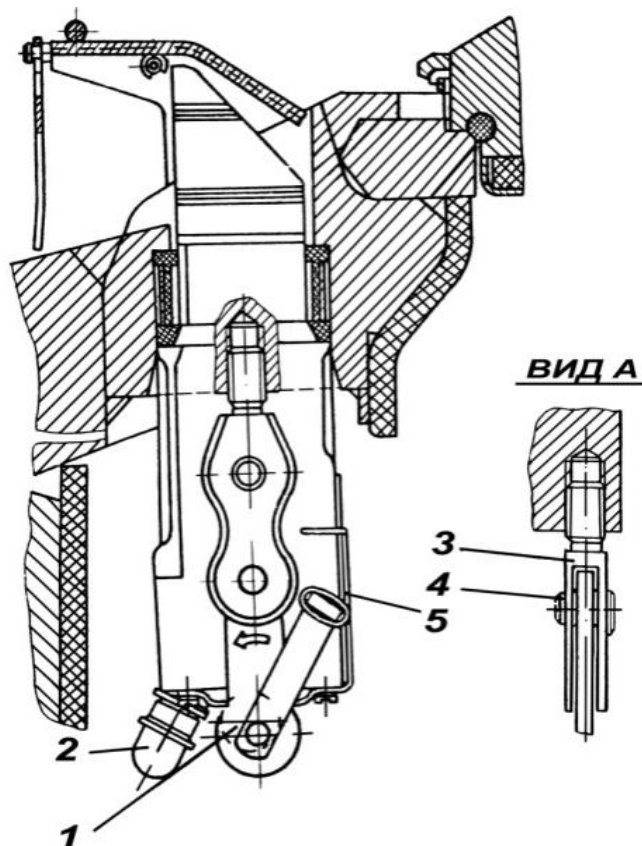
Рис. 6.4. Установка прибора ТНПО-168В:
