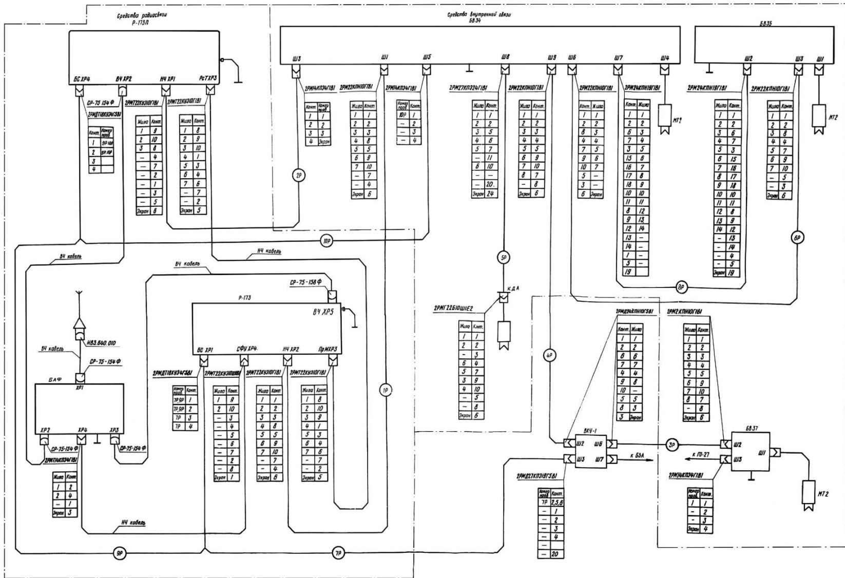
Рис. 12.5. Схема электрических соединений переговорного устройства
