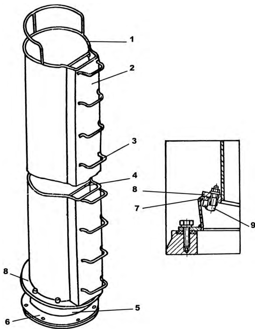
Рис. 16.3. Труба-лаз:
