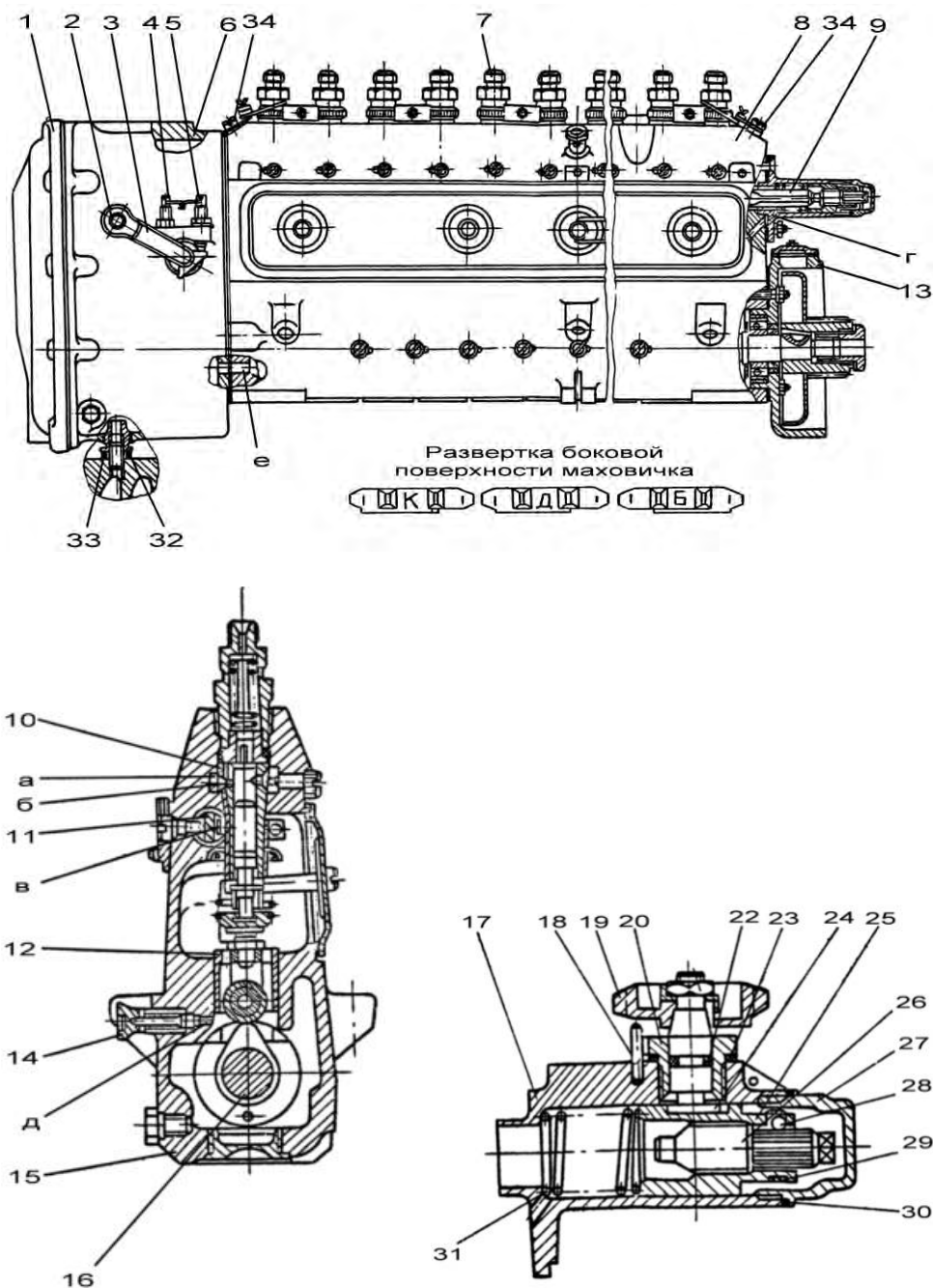
Рис. 8.9. Топливный насос высокого давления НК-12М:
