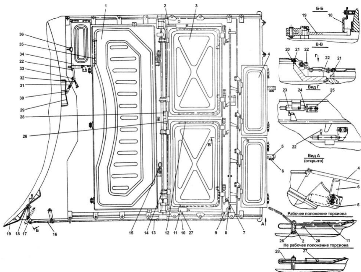
Рис. 16.1. Уплотнение крыши над силовым отделением:
