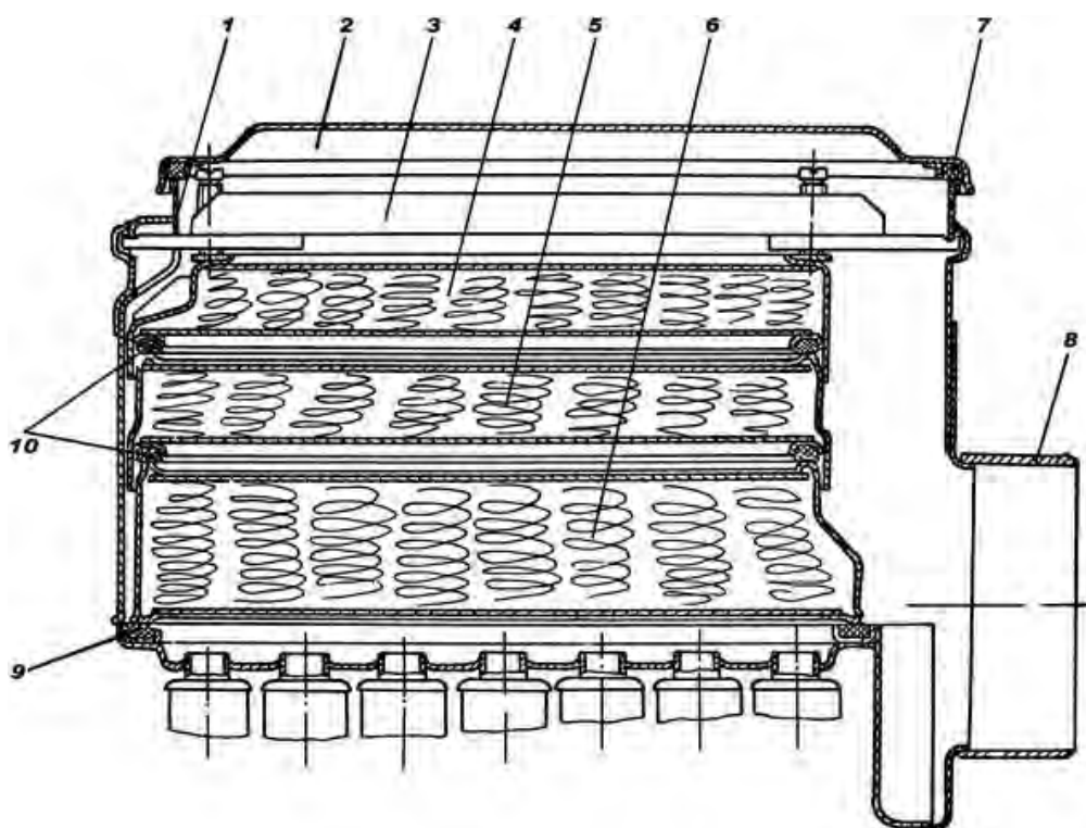
Рис. 8.17. Установка кассет в головке воздухоочистителя:
