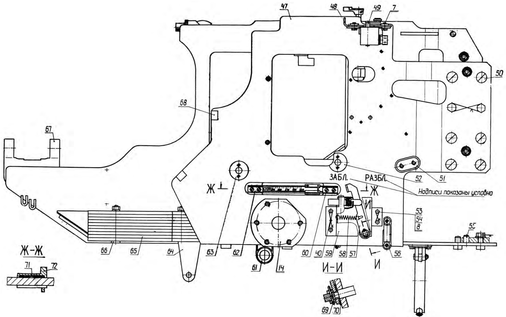
Рис. 5.7. Ограждение (продолжение)
