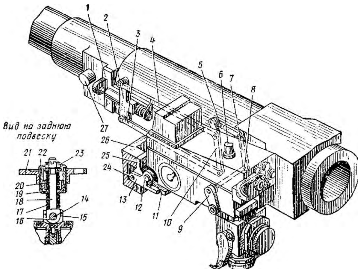
Рис. 5.28. Установка прицела-дальномера:
