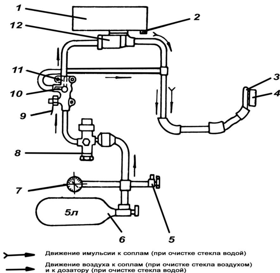
Рис. 7.1. Система гидропневматической очистки защитного стекла прицела-дальномера. Схема принципиальная:
