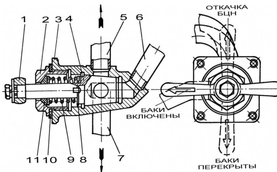
Рис. 8.5. Топливораспределительный кран:
