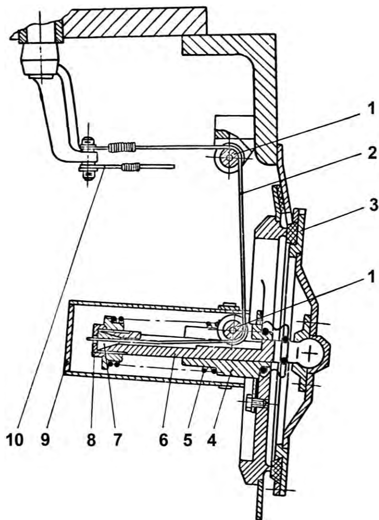
Рис. 16.7. Клапан ОПВТ с приводом: 1 – направляющие ролики; 2 – тросик; 3 – клапан; 4 – направляющая втулка; 5 – пружина; 6 – шток; 7 – сухарики; 8 – гайка; 9 – кожух; 10 – трос привода лючка перетока воды
