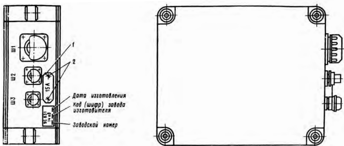
Рис. 5.58. Преобразователь напряжения 9С831: 1 – крышка; 2 – винт
