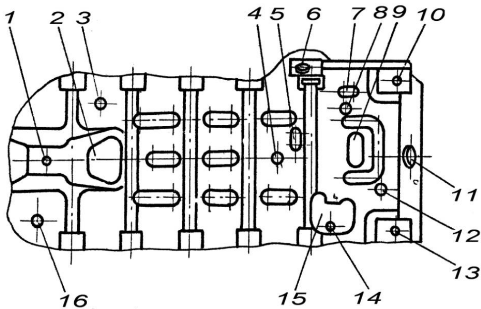
Рис. 4.2. Расположение люков на днище. Вид сверху:
