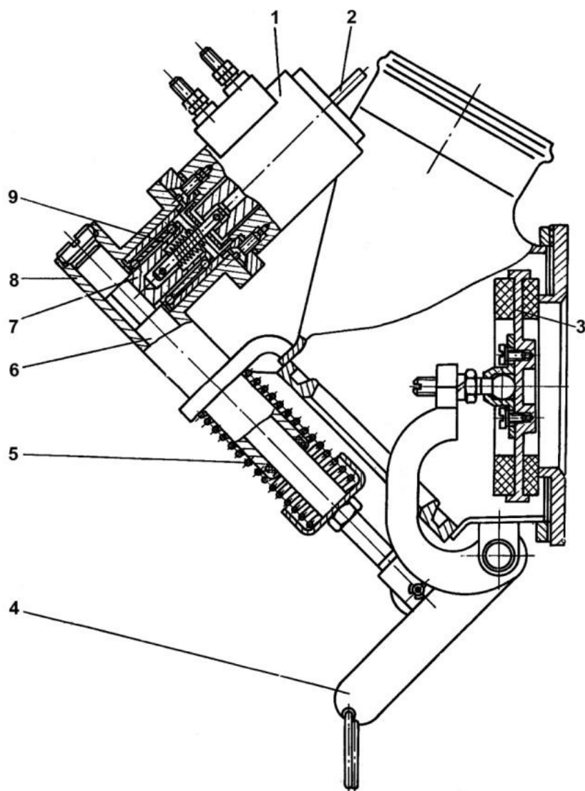
Рис. 13.6. Исполнительный механизм:
