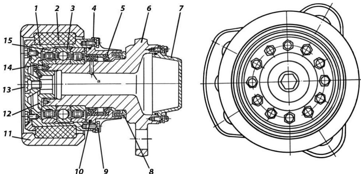
Рис. 10.3. Поддерживающий каток:
