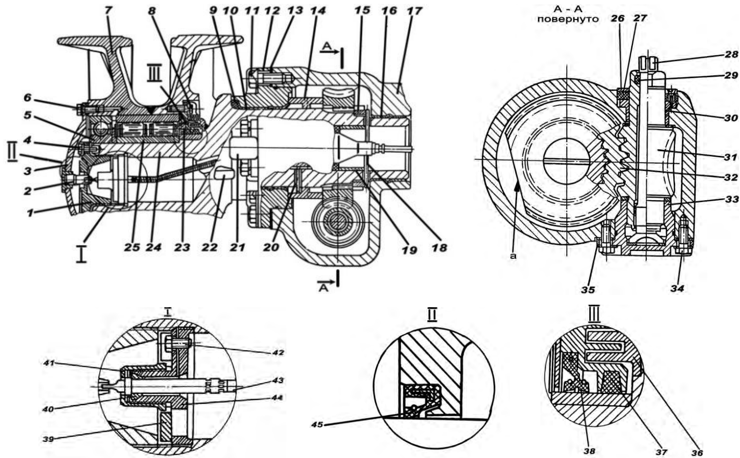
Рис. 10.4. Направляющее колесо и натяжной механизм:
