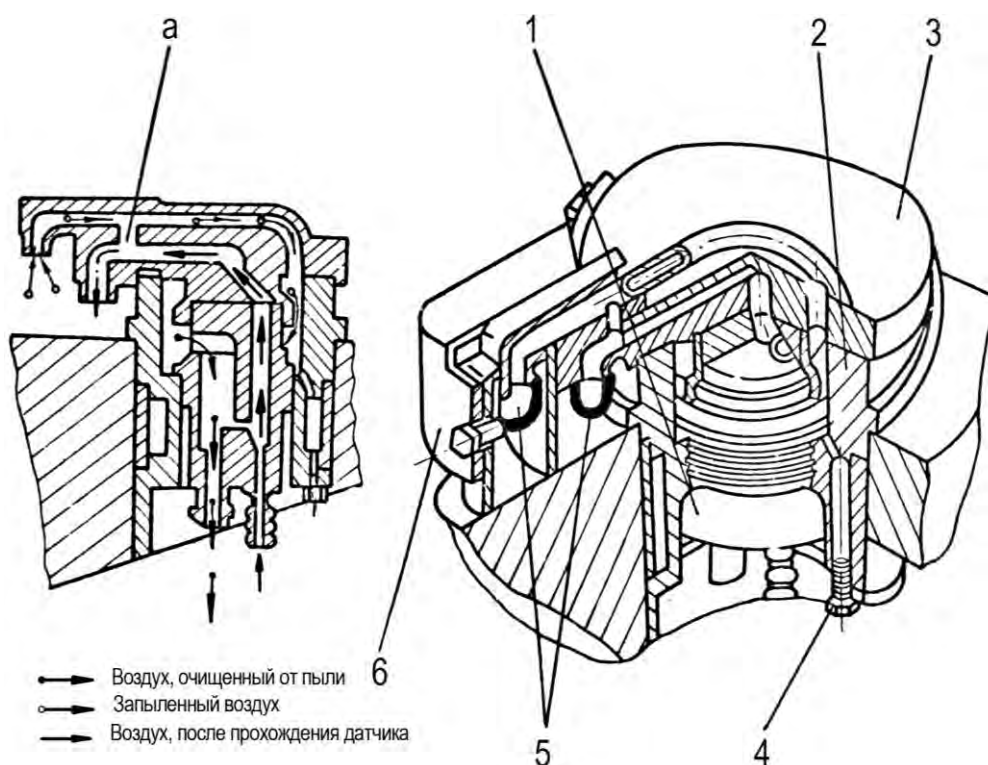
Рис. 13.3. Воздухозаборное устройство:
