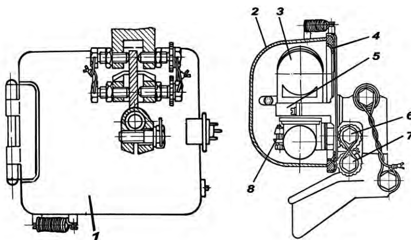
Рис. 5.18. Установка коллиматорного прицела К10-Т:
