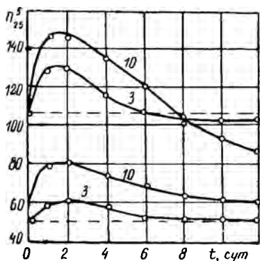
Рис. 1. Зависимость пенетрации дегтей с добавкой серы от времени
