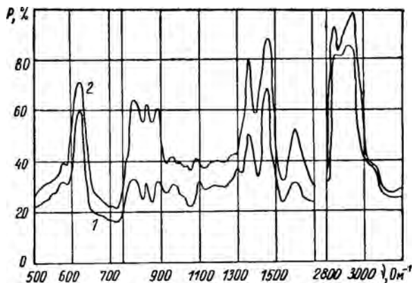
Рис. 2. ИК-спектры битумов с добавкой СШ, вводимого при температуре 130—140 °С
